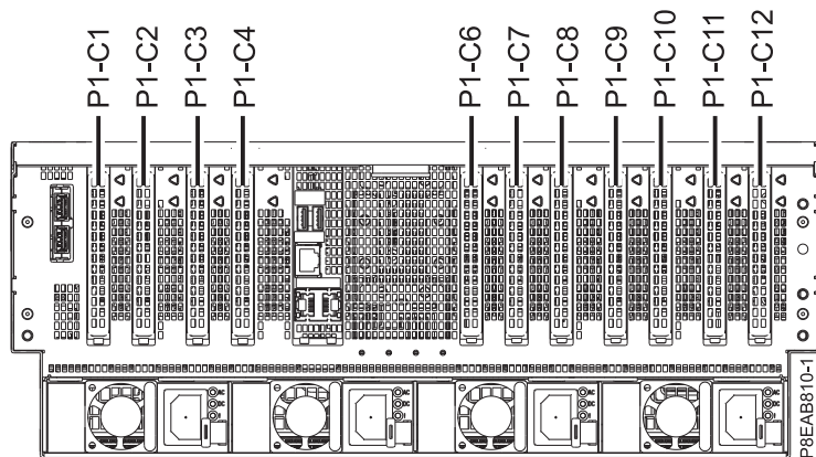
Rysunek 1. Widok z tyłu serwera 8408-44E lub 8408-E8E z kodami położenia gniazd PCIe
