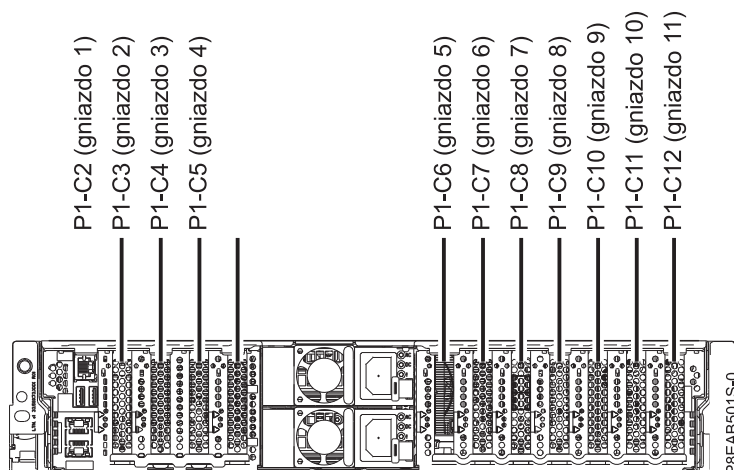
Rysunek 1. Widok z tyłu serwera 5148-21L, 5148-22L, 8247-21L, 8247-22L, 8284-21A lub 8284-22A z kodami położenia gniazd PCIe
