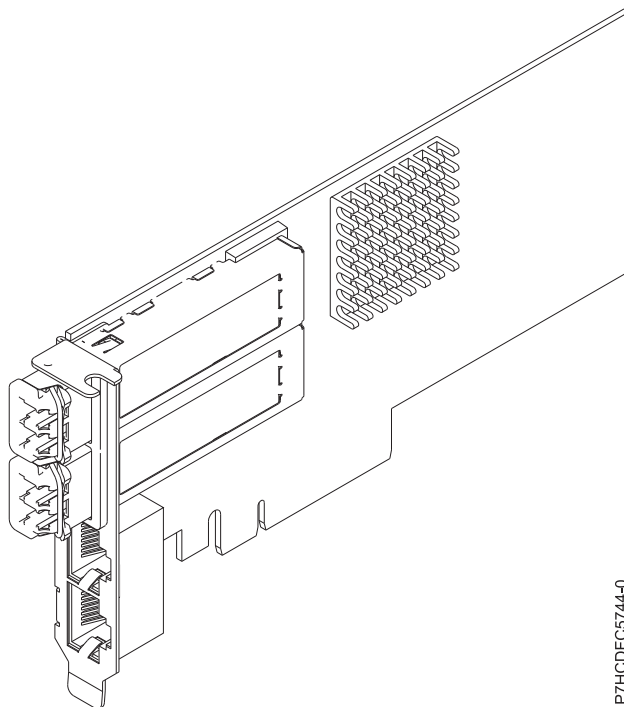
図 42. FC EN0V アダプター
