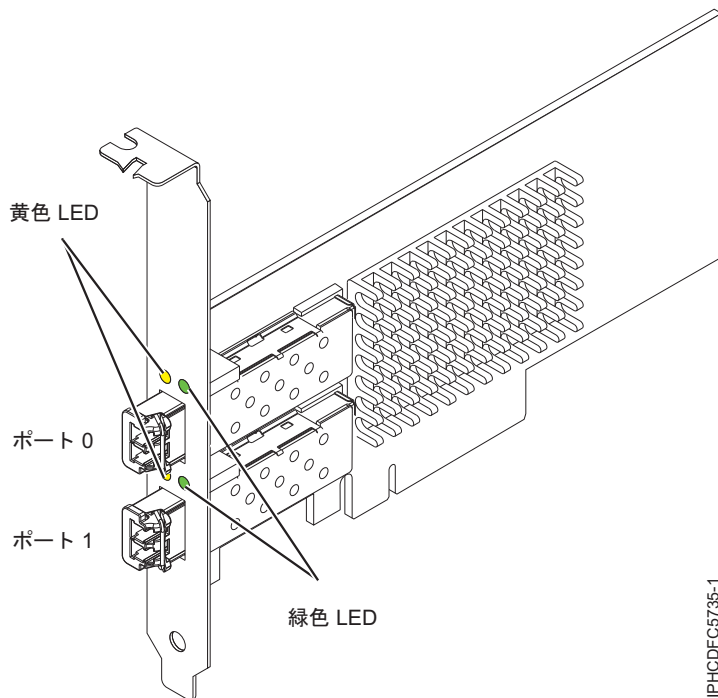
図 10. EN0B アダプター
