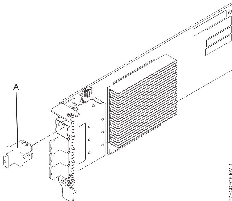
図 18. PCIe3 LP 4 x8 SAS ポート・アダプター
