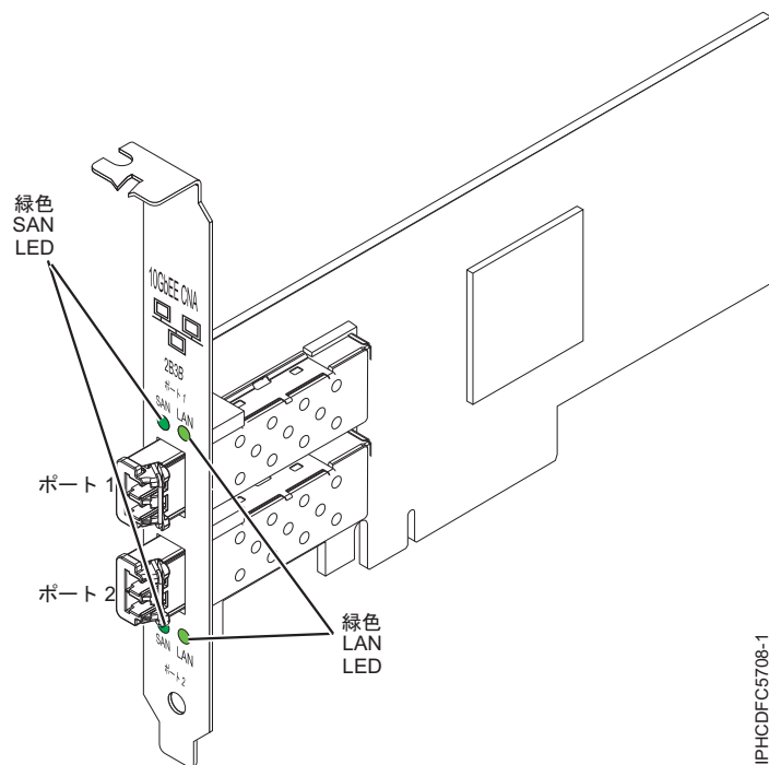
図 20. PCIe LP 10-Gb FCoE 2 ポート・アダプター
