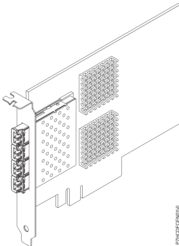
図 11. PCIe2 LP 8 Gb 4 ポート・ファイバー・チャンネル・アダプター
