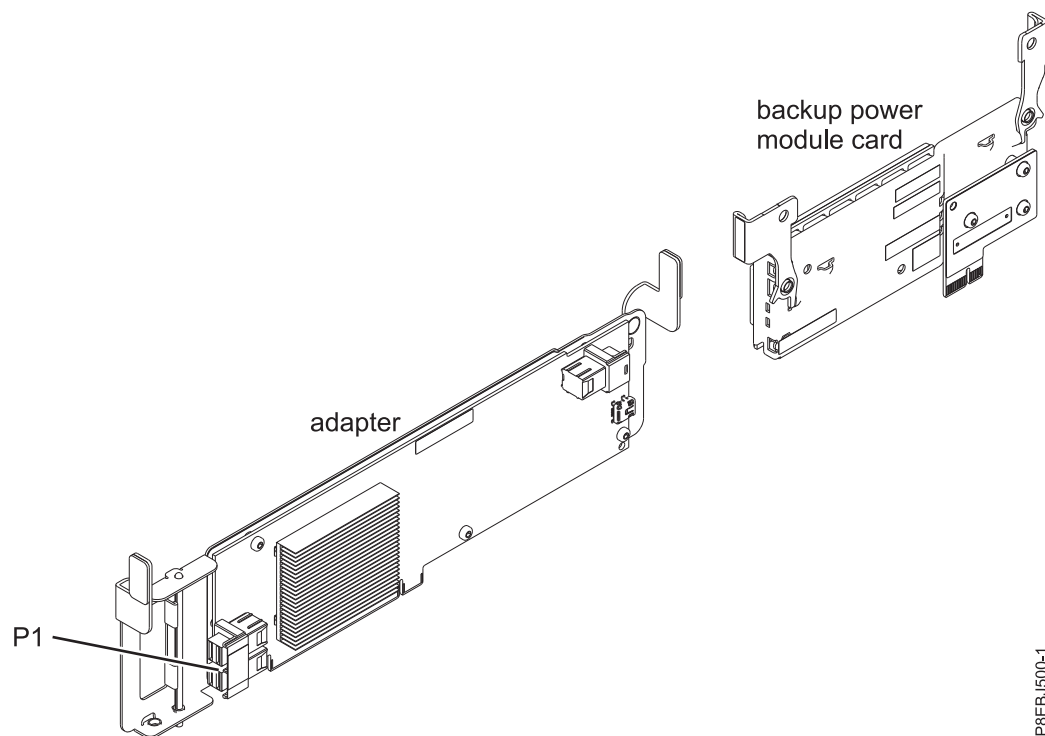
図 56. PCIe x8 キャッシュ SAS RAID 内部アダプター 6Gb
