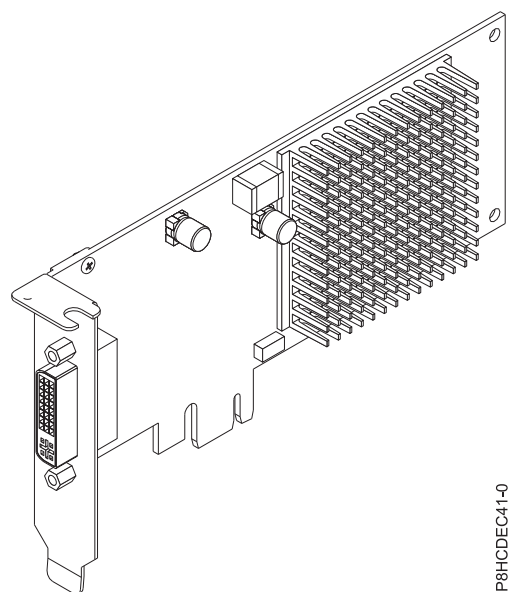
図 13. PCIe2 LP 3D グラフィックス・アダプター
