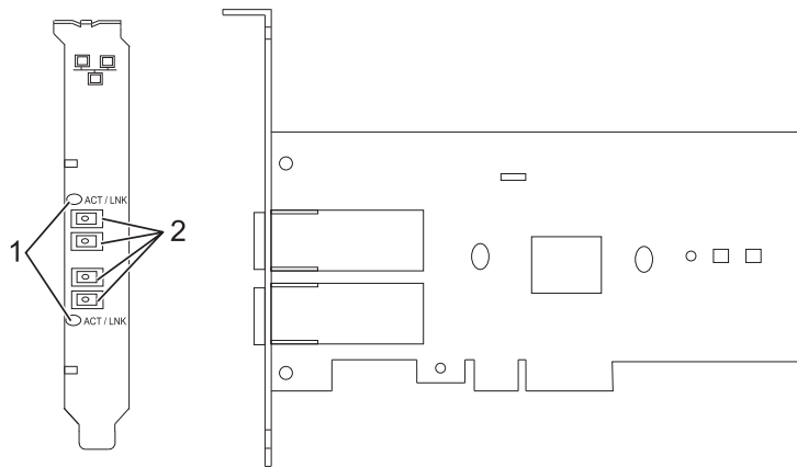
図 21. PCIe LP 2 ポート 1GbE SX アダプター
