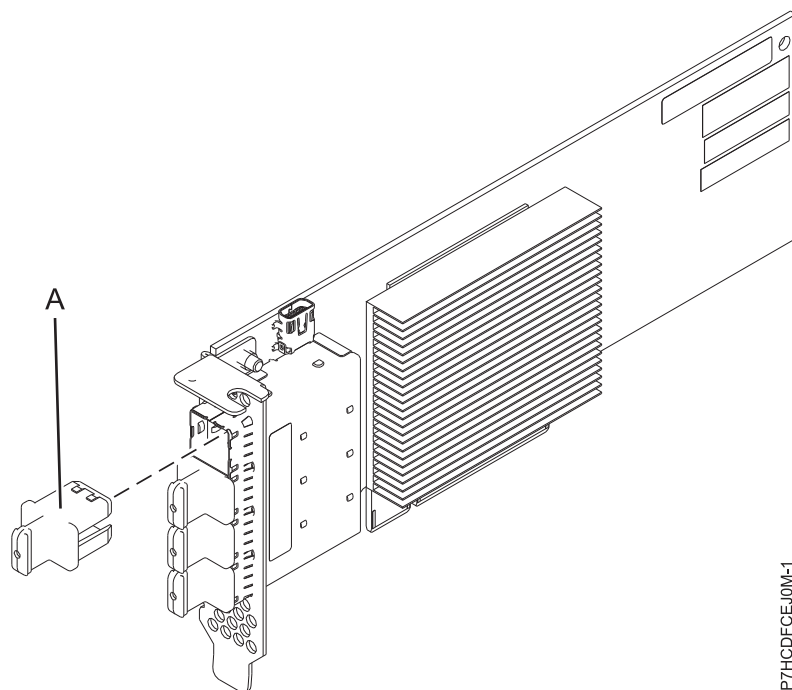
図 17. PCIe3 RAID SAS クワッド・ポート 6 Gb LP アダプター
