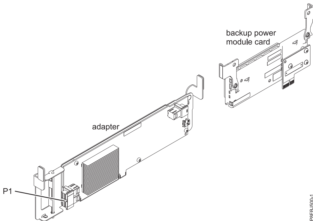
図 55. PCIe3 x8 キャッシュ SAS RAID 内部アダプター 6Gb
