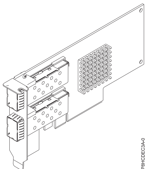
図 29. FC EC3A アダプター
