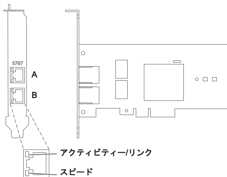
図 24. 2 ポート 10/100/1000 Base-TX イーサネット PCI Express アダプター
