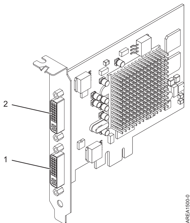
図 12. PCIe LP POWER GXT145 グラフィックス・アクセラレーター・アダプター
