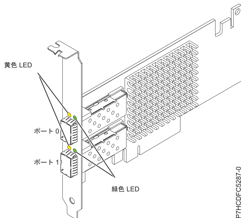
図 25. PCIe2 LP 2 ポート 10GbE SR アダプター
