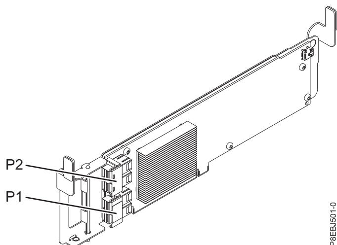
図 54. PCIe3 x8 SAS RAID 内部アダプター 6Gb
