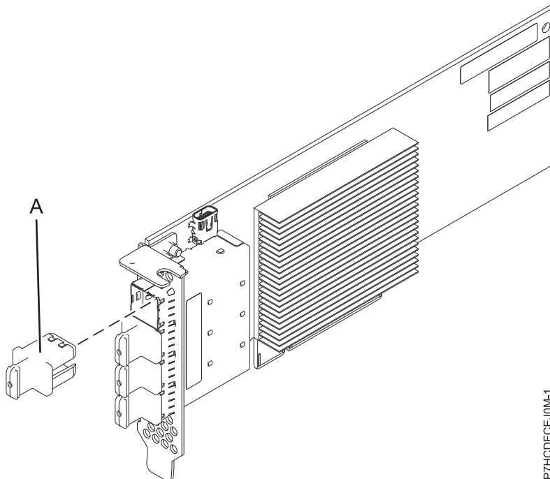
図 16. PCIe3 LP 4 x8 SAS ポート・アダプター
