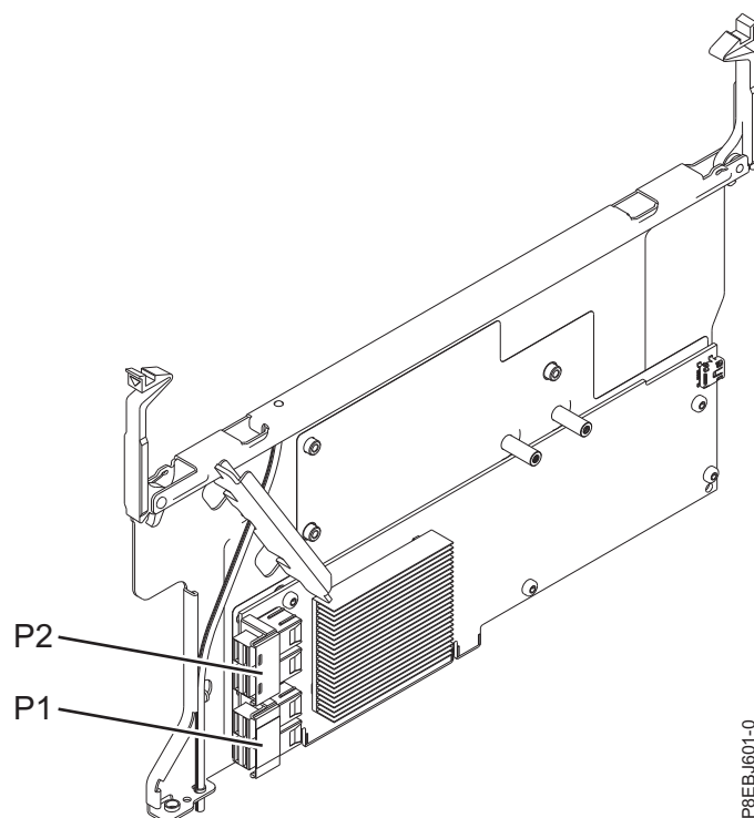
図 43. PCIe3 x8 SAS RAID 内部アダプター 6Gb
