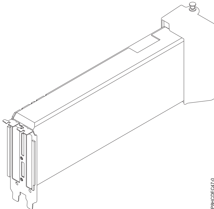
図 36. PCIe 第 3 世代 x16 GPU アダプター
