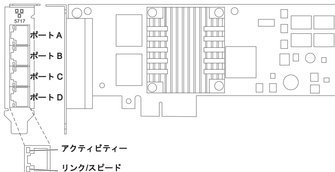
図 16. 4 ポート 10/100/1000 Base-TX PCIe アダプター
