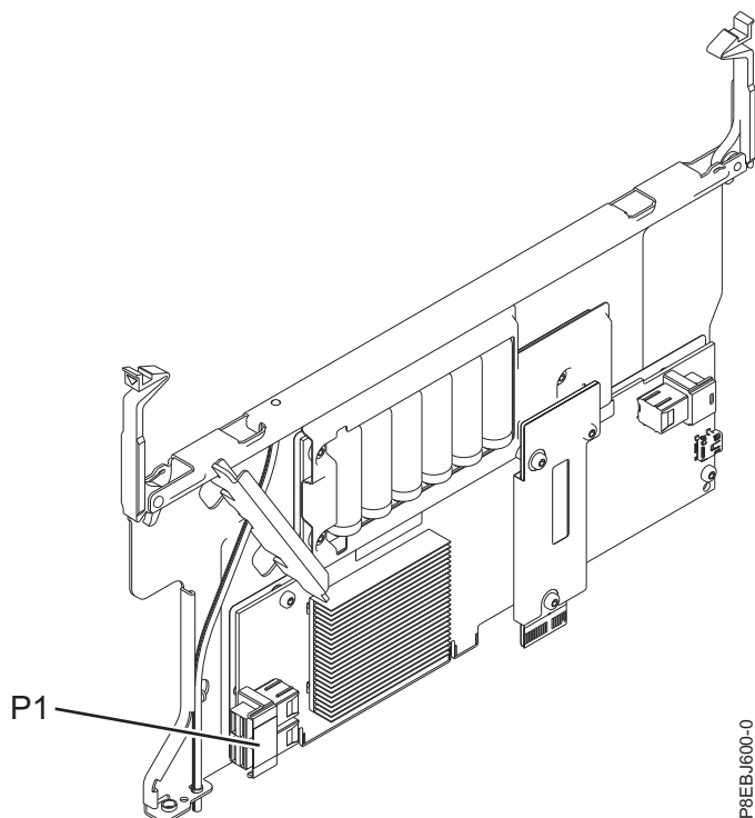
図 44. PCIe x8 キャッシュ SAS RAID 内部アダプター 6Gb
