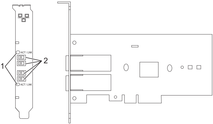
図 19. 2 ポート・ギガビット・イーサネット SX PCI Express アダプター
