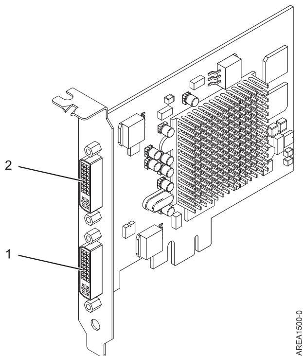
図 9. POWER GXT145 PCI Express グラフィックス・アクセラレーター アダプター
