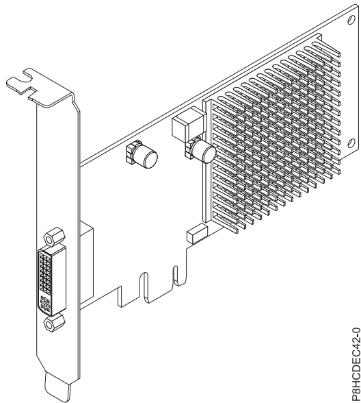
図 10. PCIe2 3D グラフィックス・アダプター
