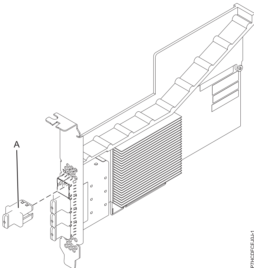
図 13. PCIe3 4 x8 SAS ポート・アダプター
