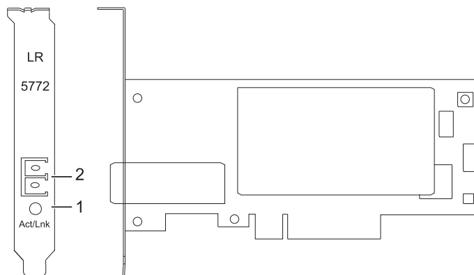
図 21. 10 ギガビット・イーサネット LR PCI Express アダプター
