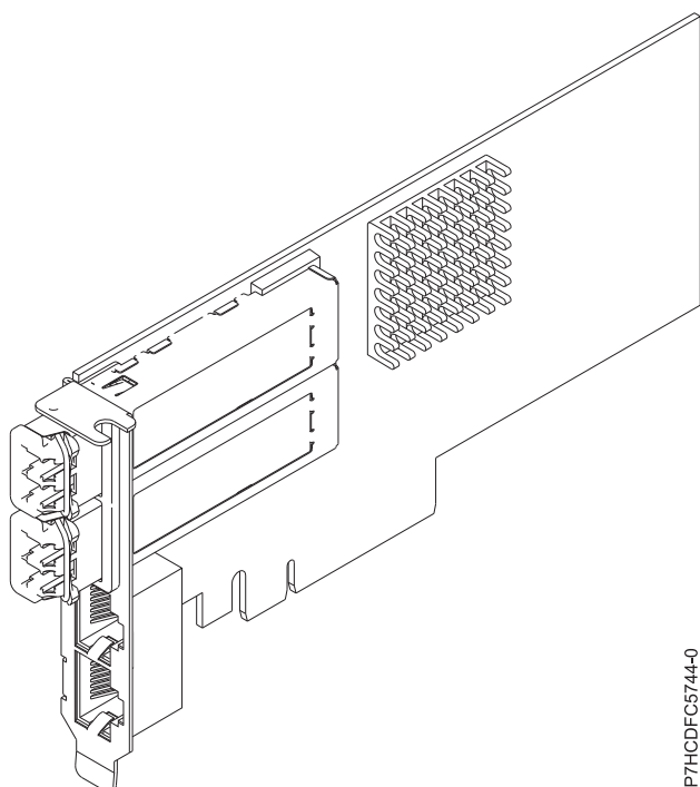
図 17. PCIe2 2x10GbE SR 2x1GbE UTP アダプター
