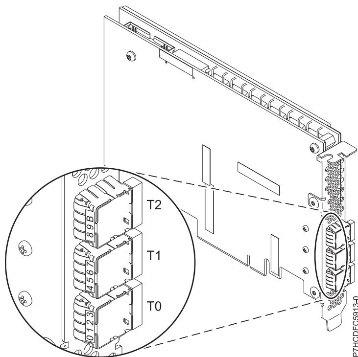
図 42. ESA3 アダプター
