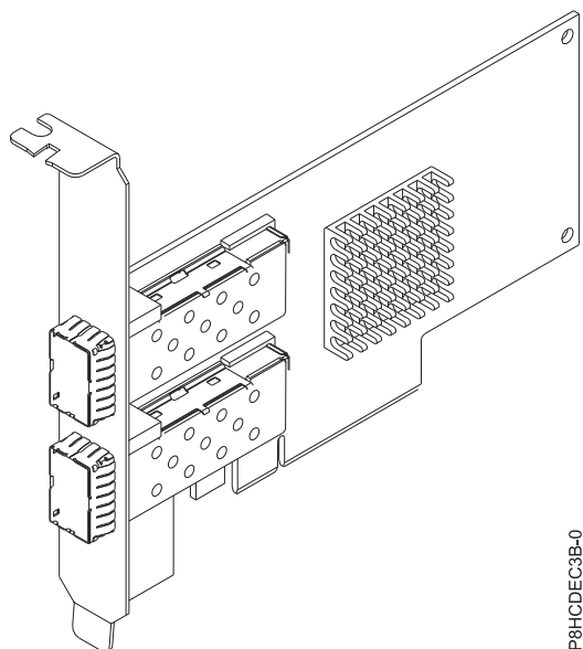
図 26. FC EC3B アダプター
