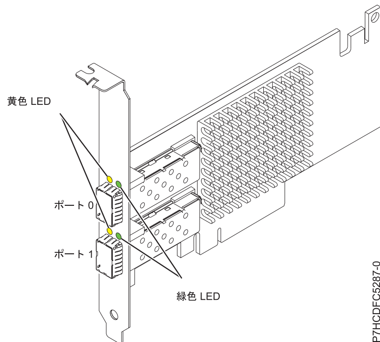
図 14. PCIe 2 ポート 10GbE SR アダプター
