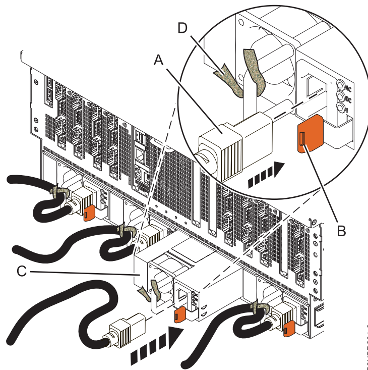
図 13. 8408-E8E システムの電源装置の取り替え
