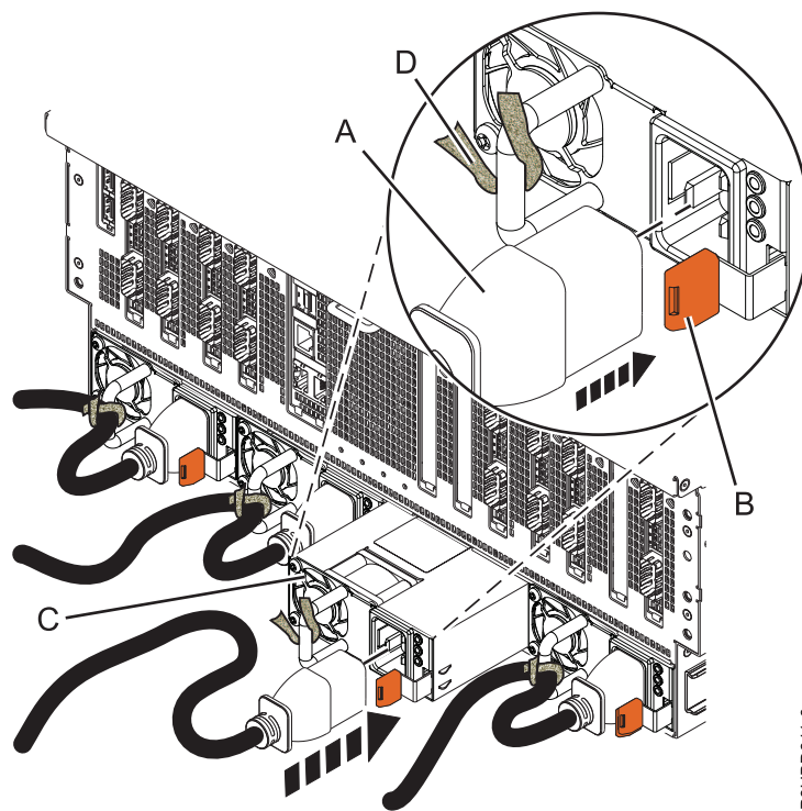
図 12. 8408-44E システムの電源装置の取り替え
