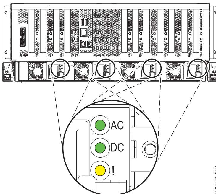
図 1. 8408-44E または 8408-E8E システムでの電源装置および LED の位置
