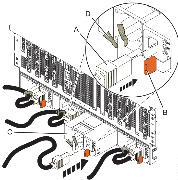
図 6. 8408-E8E システムの電源装置の取り替え
