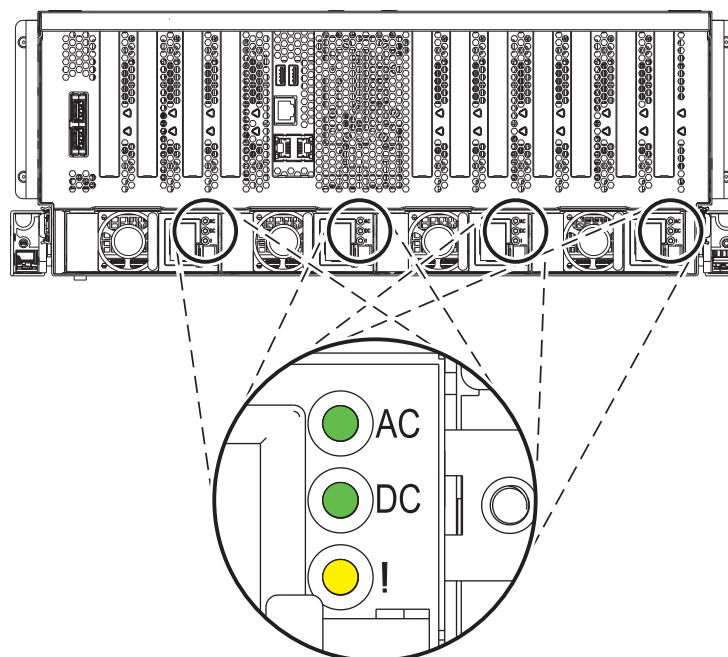
図 8. 8408-44E または 8408-E8E システムでの電源装置および LED の位置
