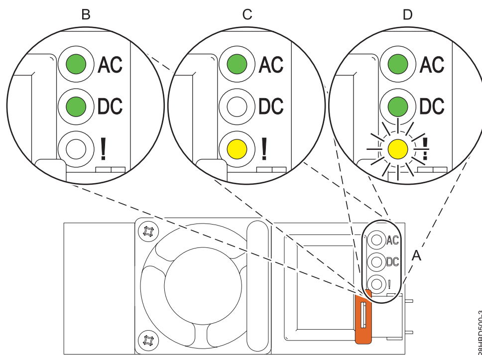
図 2. 正常に作動している電源装置および障害のある電源装置の LED
