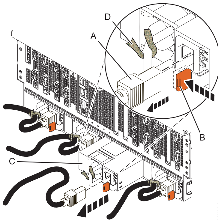
図 11. 8408-E8E システムからの電源装置の取り外し
