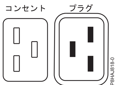
図 24. 8408-44E システムのコネクター
