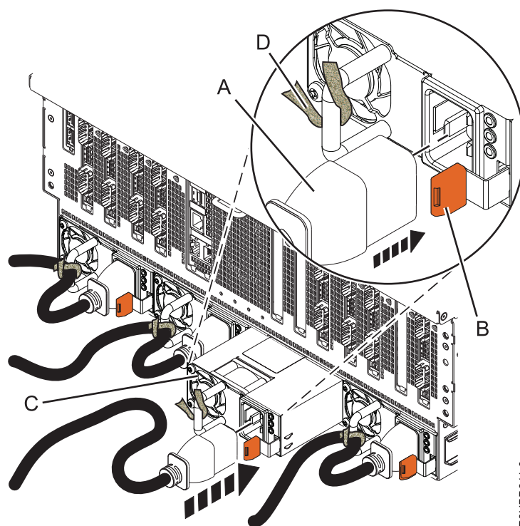
図 5. 8408-44E システムの電源装置の取り替え
