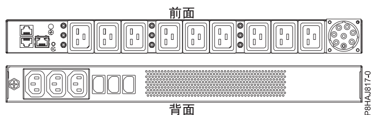
図 25. 8408-44E システムの PDU
