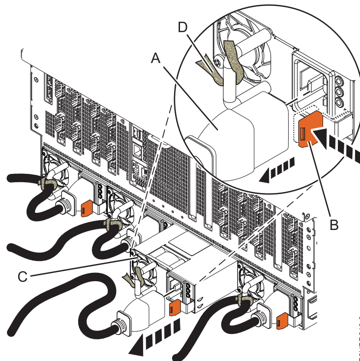
図 10. 8408-44E システムからの電源装置の取り外し
