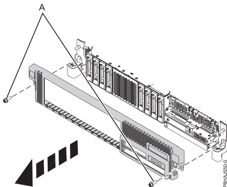
図 27. 前面カバーの取り外し
