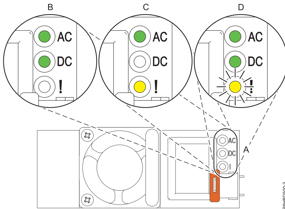
図 8. 正常に作動している電源装置および障害のある電源装置の LED
