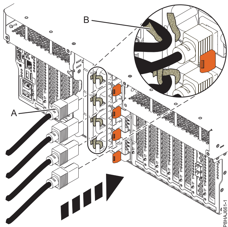
図 24. 8247-42L、8286-41A、または 8286-42A システムへの電源コードの接続
