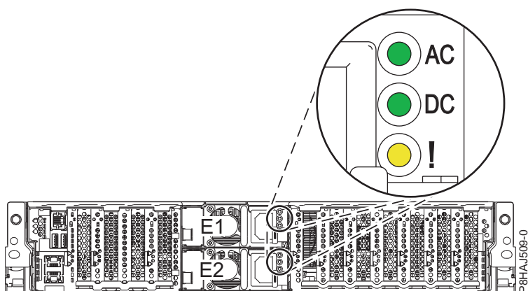
図 1. システムの電源装置と LED の位置
