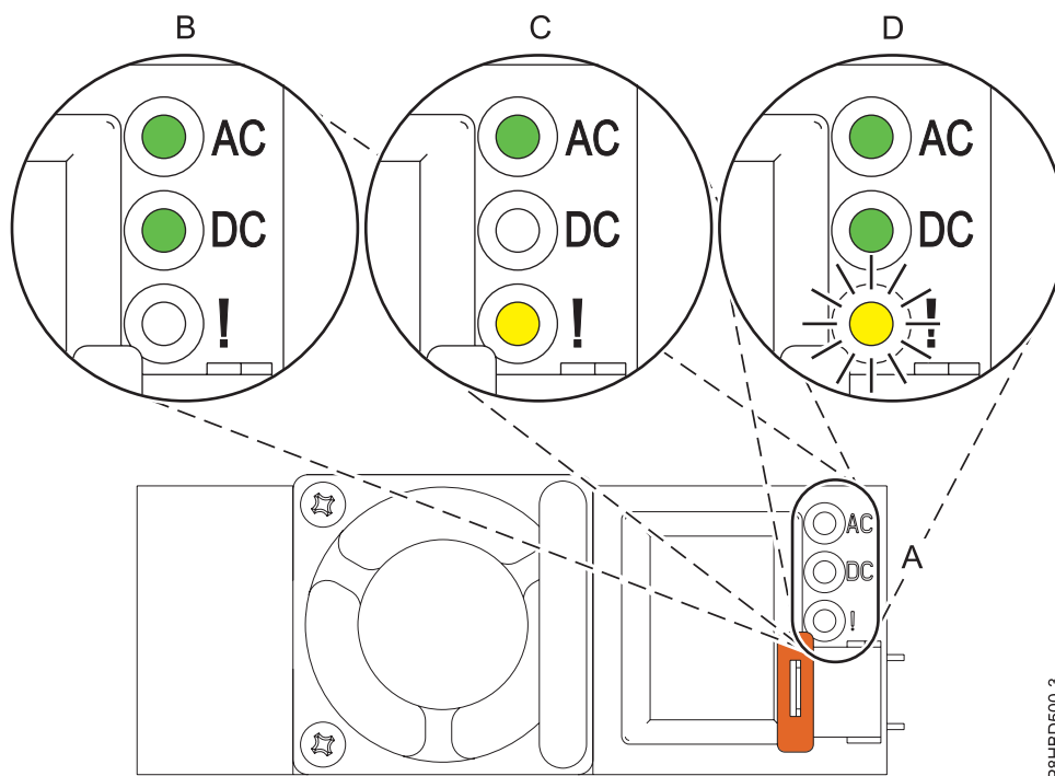
図 6. 正常に作動している電源装置および障害のある電源装置の LED
