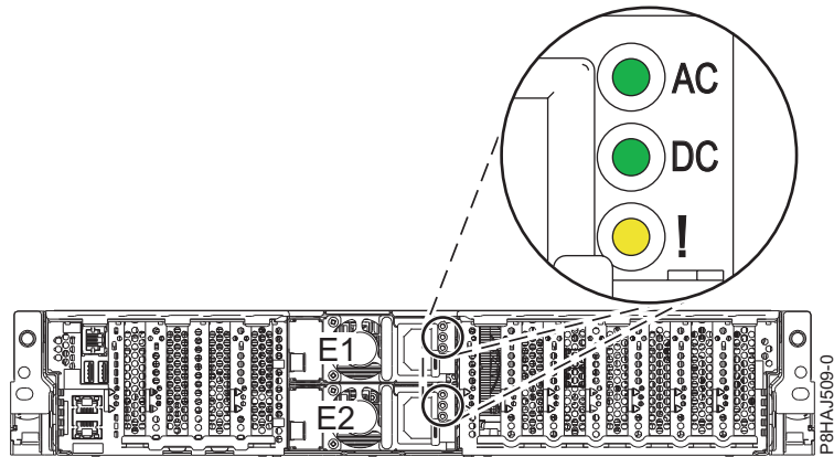
図 7. システムの電源装置と LED の位置
