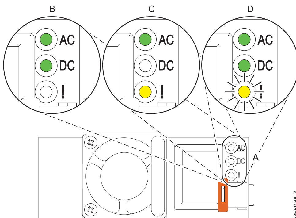
図 12. 正常に作動している電源装置および障害のある電源装置の LED
