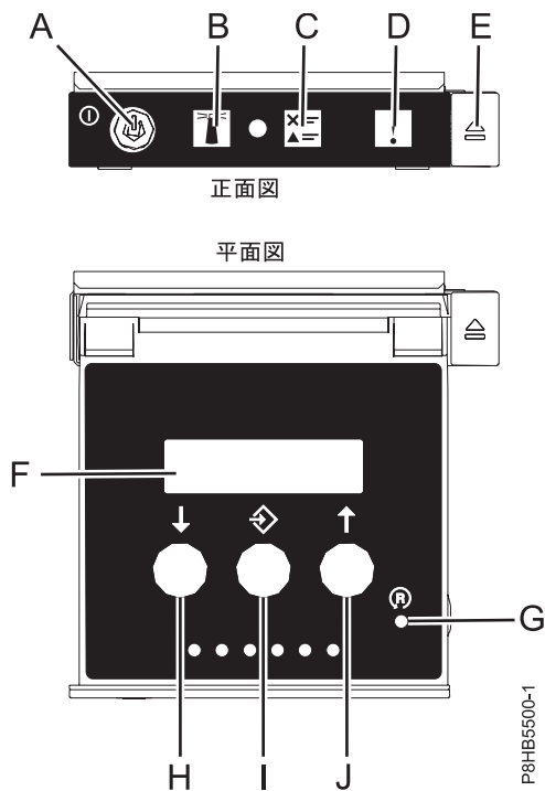
図 14. コントロール・パネル
