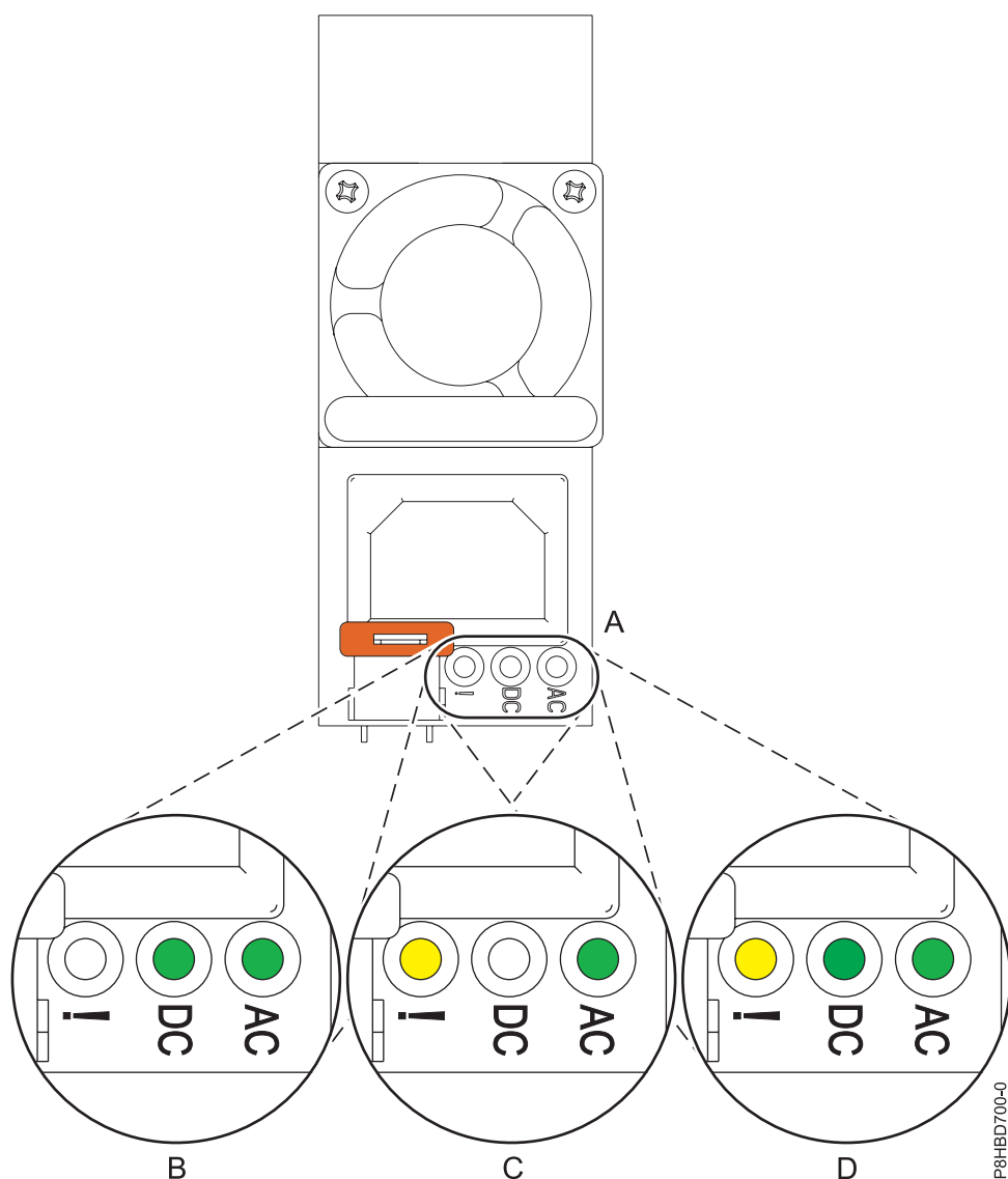
図 18. スタンドアロン型システムでの正常に作動している電源装置および障害のある電源装置の LED
