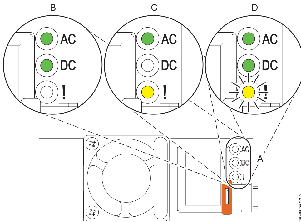
図 17. ラック・マウント型システムでの正常に作動している電源装置および障害のある電源装置の LED
