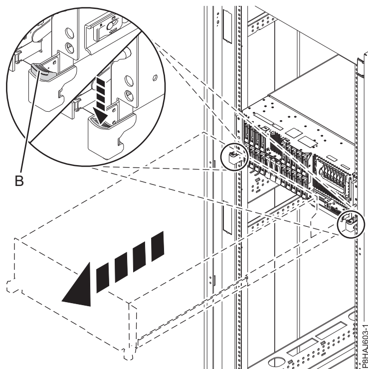
図 63. サイド・ラッチのリリース
