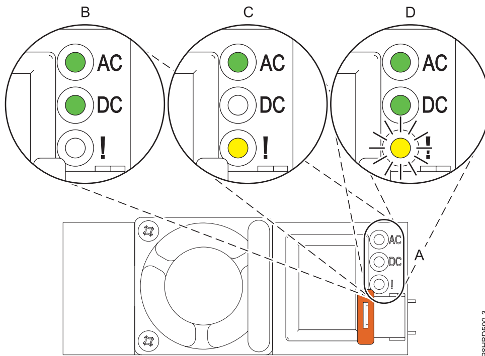
図 23. ラック・マウント型システムでの正常に作動している電源装置および障害のある電源装置の LED
