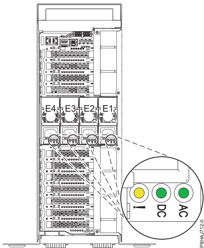
図 2. スタンドアロン型システムの電源装置と LED の位置
