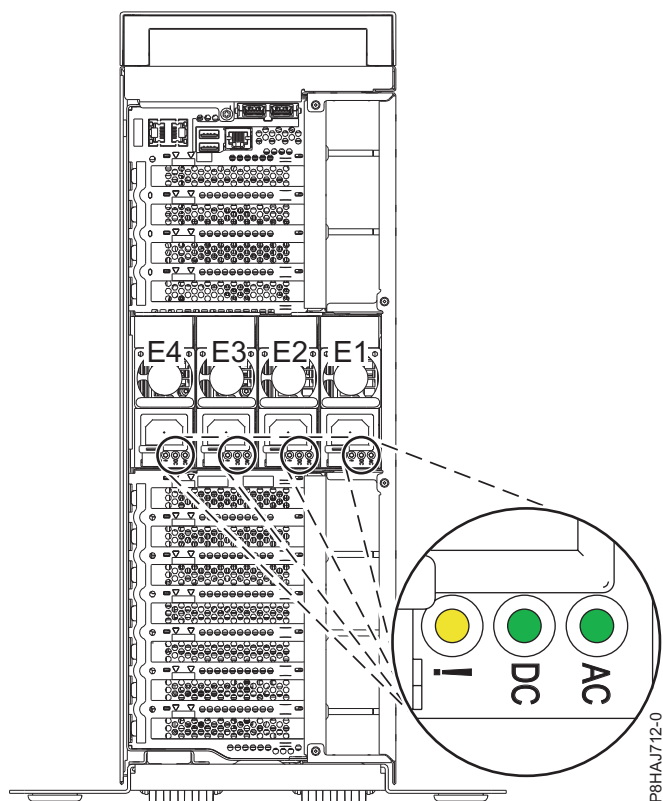
図 14. スタンドアロン型システムの電源装置と LED の位置
