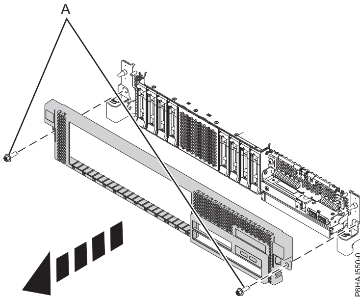
図 39. 前面カバーの取り外し
