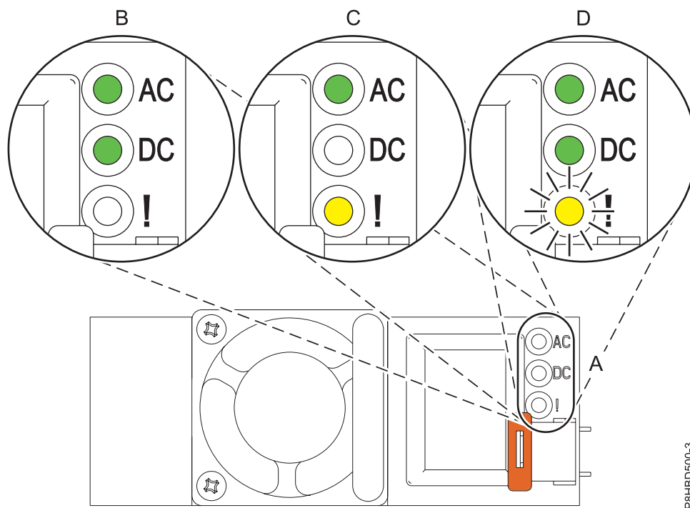
図 15. ラック・マウント型システムでの正常に作動している電源装置および障害のある電源装置の LED
