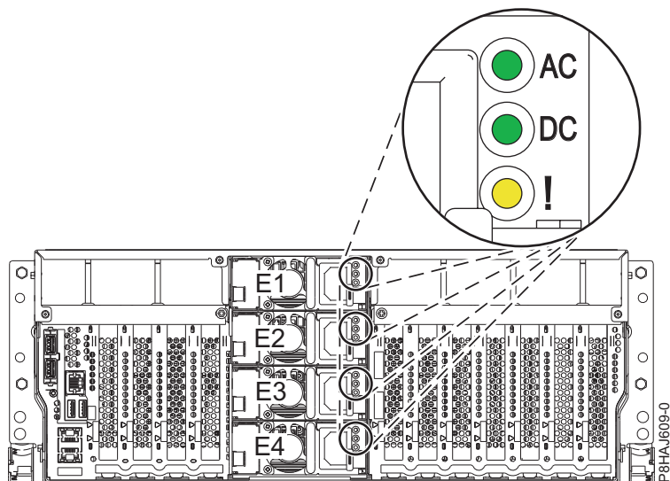
図 13. ラック・マウント型システムの電源装置と LED の位置
