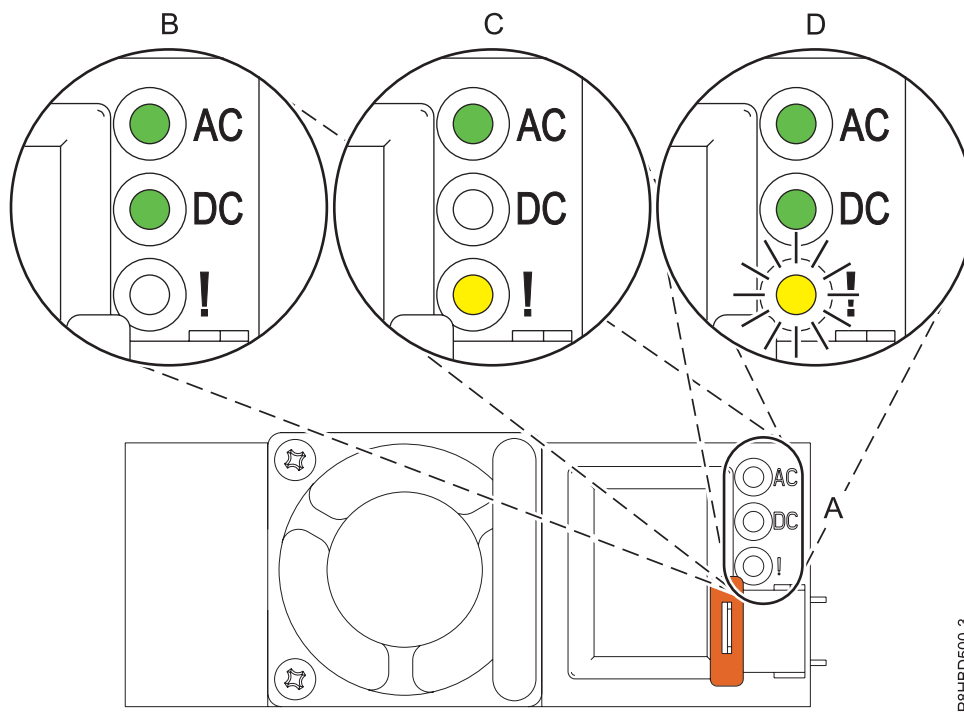
図 5. ラック・マウント型システムでの正常に作動している電源装置および障害のある電源装置の LED
