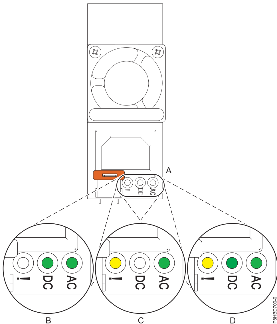
図 16. スタンドアロン型システムでの正常に作動している電源装置および障害のある電源装置の LED
