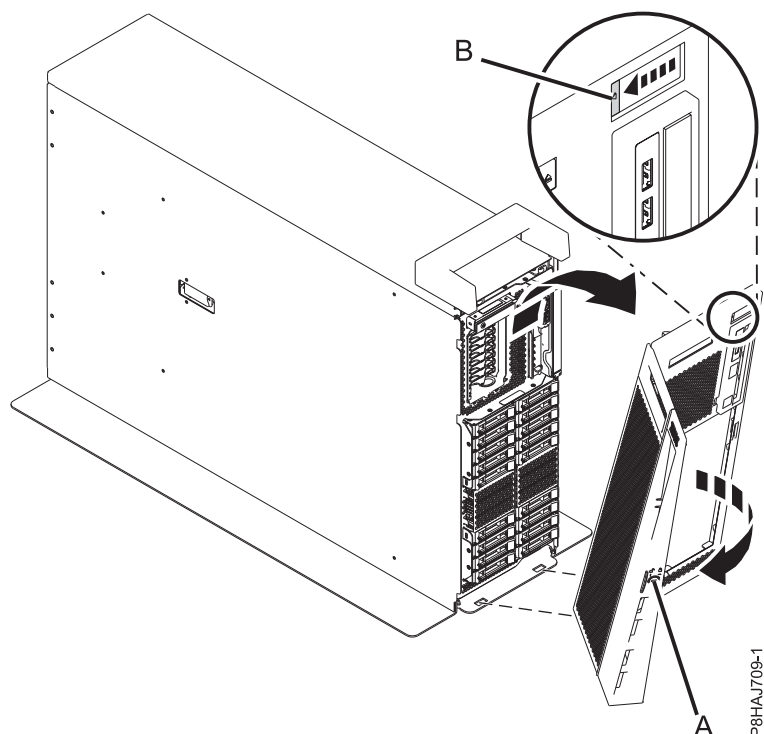
図 41. 前面カバーの取り外し
