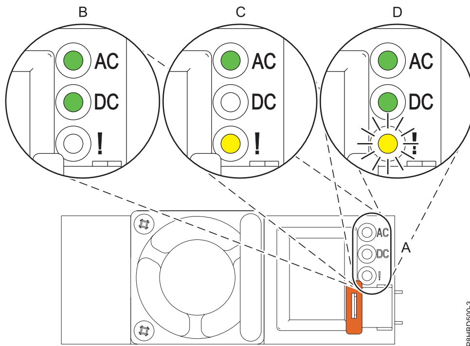
図 11. ラック・マウント型システムでの正常に作動している電源装置および障害のある電源装置の LED
