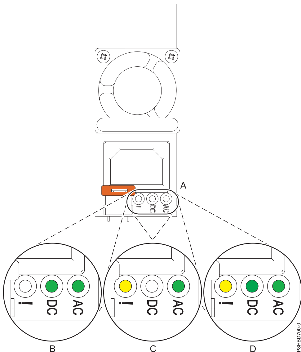
図 12. スタンドアロン型システムでの正常に作動している電源装置および障害のある電源装置の LED
