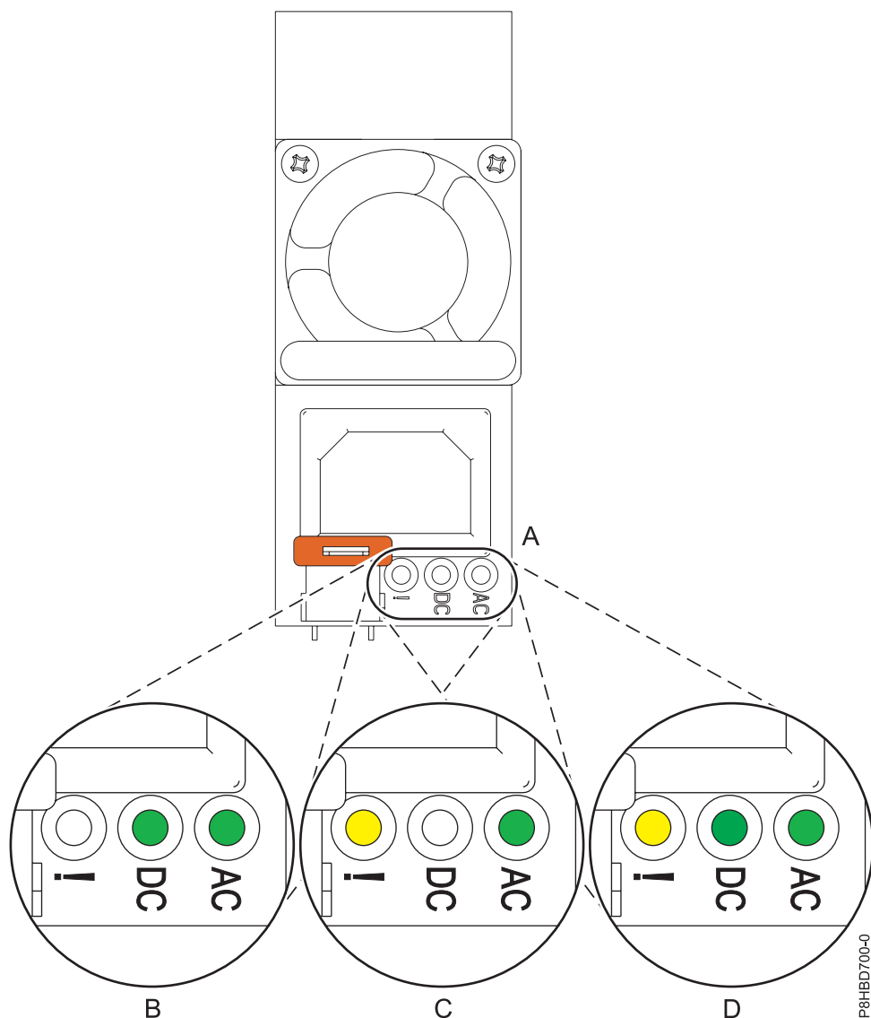
図 6. スタンドアロン型システムでの正常に作動している電源装置および障害のある電源装置の LED
