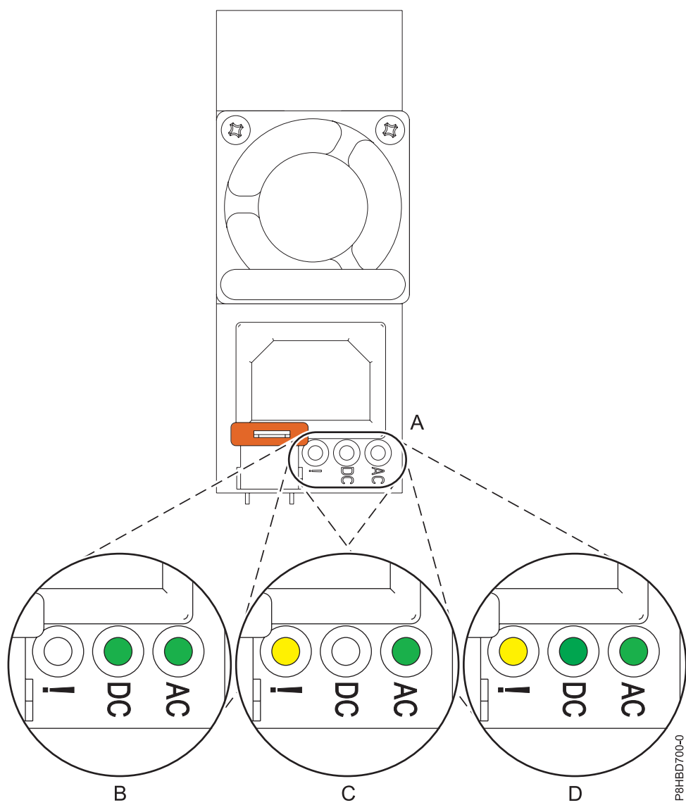
図 24. スタンドアロン型システムでの正常に作動している電源装置および障害のある電源装置の LED
