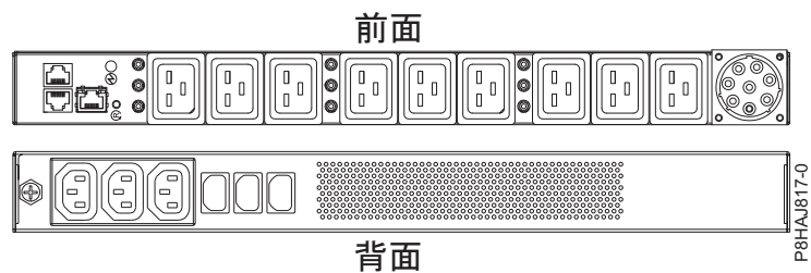
図 20. 8408-44E システムの PDU
