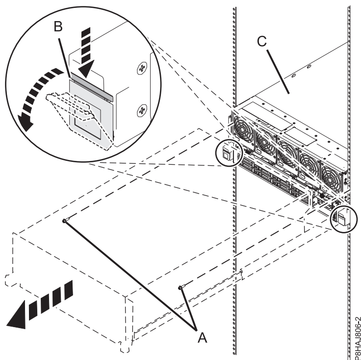
図 16. システムの保守位置への設置
