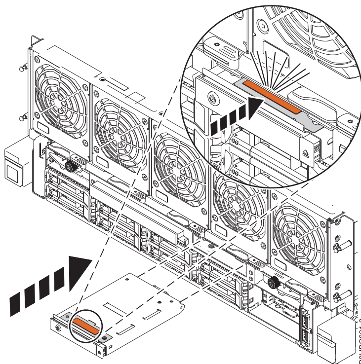
図 2. 8408-44E または 8408-E8E システムでのコントロール・パネルの再取り付け
