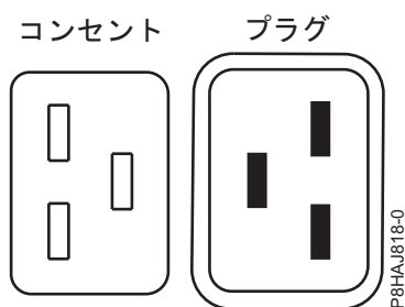
図 19. 8408-44E システムのコネクタ
