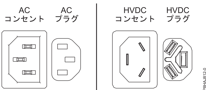
図 24. AC コネクターと HVDC コネクター
