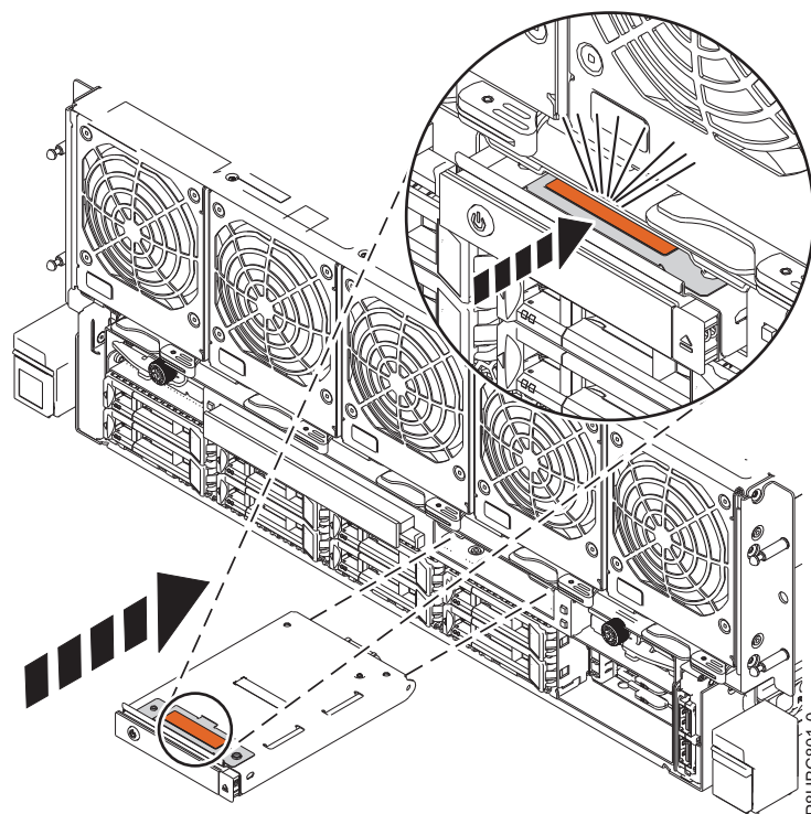
図 5. 8408-44E または 8408-E8E システムでのコントロール・パネルの再取り付け
