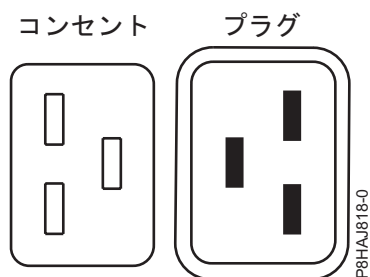
図 25. 8408-44E システムのコネクター
