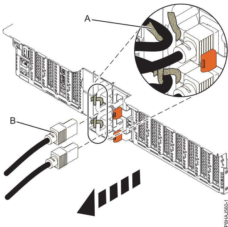
図 22. 5148-21L、5148-22L、8247-21L、8247-22L、8284-21A、または 8284-22A システムからの電源コードの取り外し
