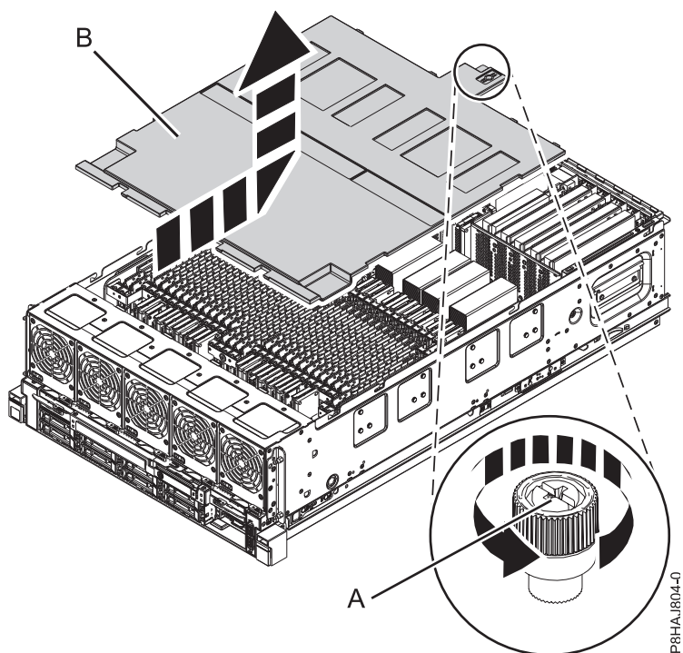
図 12. 安全カバーの取り外し
