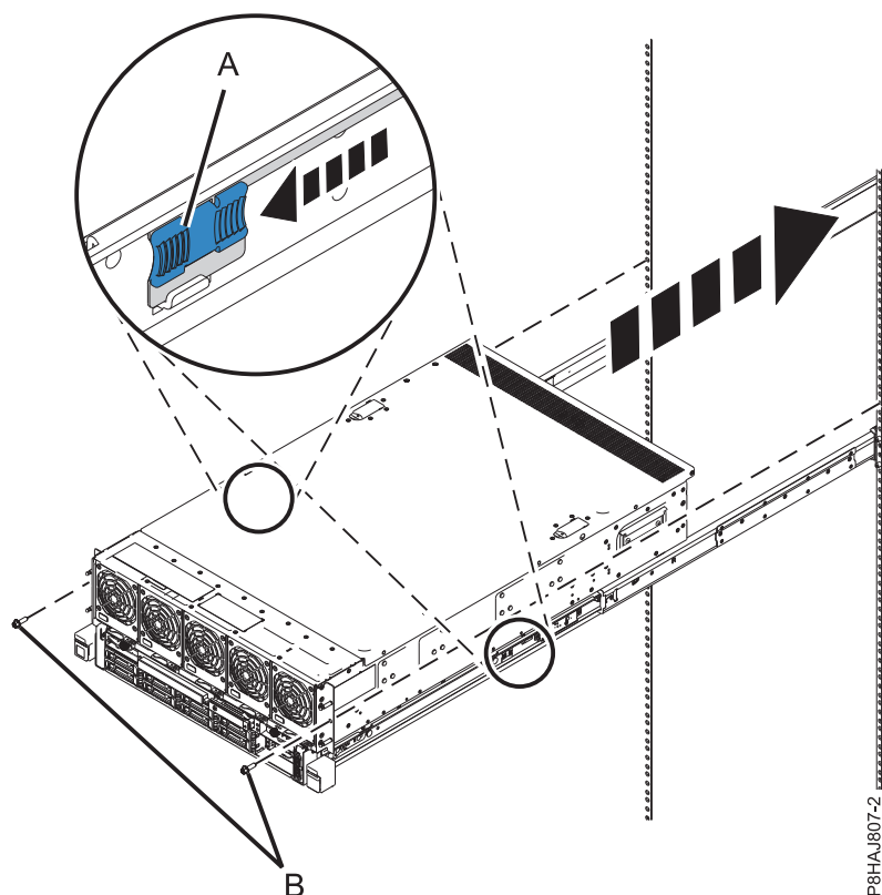
図 17. システムの操作位置への設置
