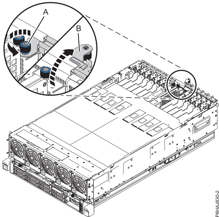
図 14. 入出力ラッチのオープン
