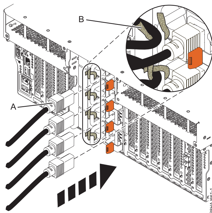
図 27. 8247-42L、8286-41A、または 8286-42A システムへの電源コードの接続
