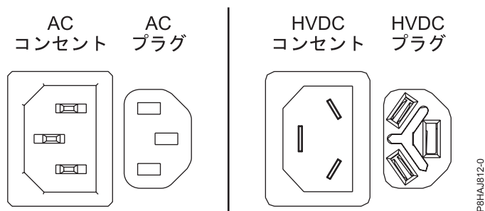
図 18. AC コネクタと HVDC コネクタ
