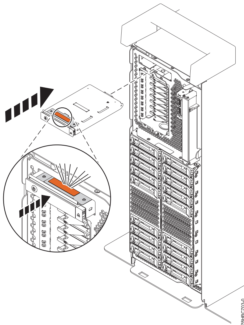
図 4. スタンドアロン・システムのコントロール・パネルの再取り付け
