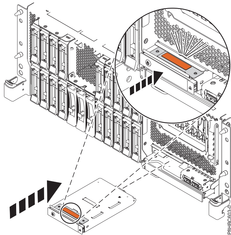
図 3. ラック・マウント型システムのコントロール・パネルの再取り付け
