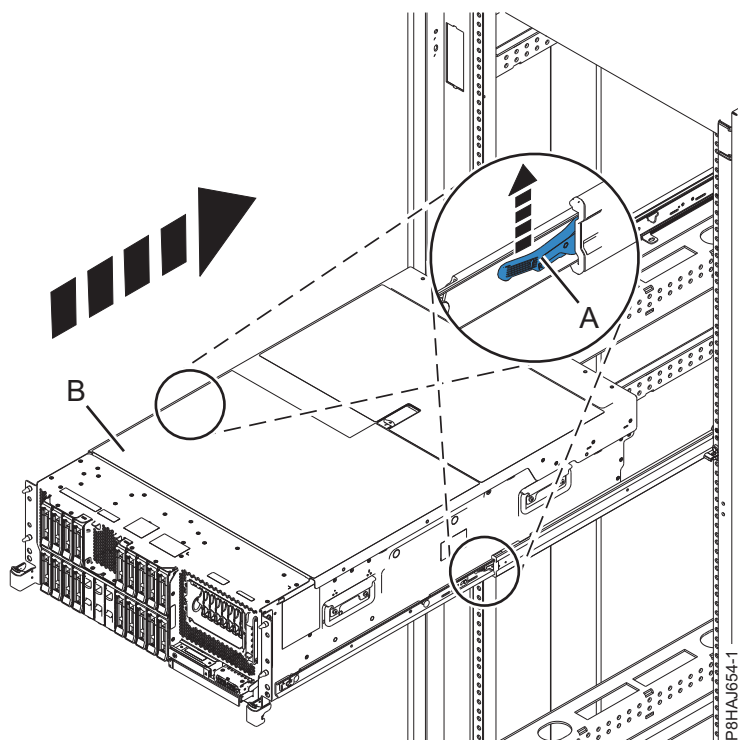
図 37. システムの操作位置への設置
