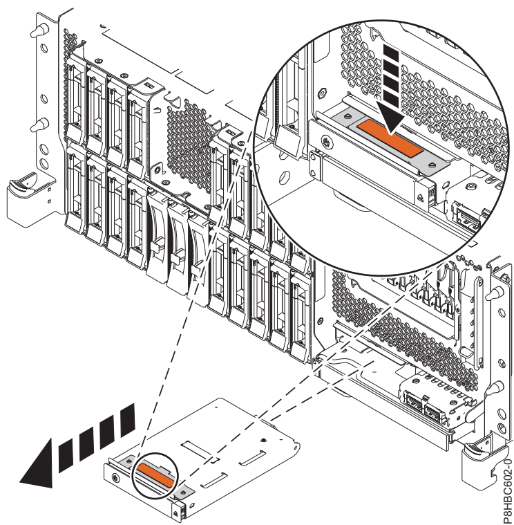
図 1. ラック・マウント型システムのコントロール・パネルの取り外し
