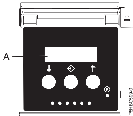
図 5. コントロール・パネルの機能画面
