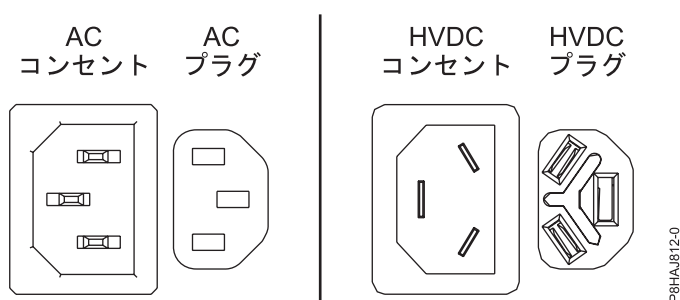
図 44. AC コネクターと HVDC コネクター
