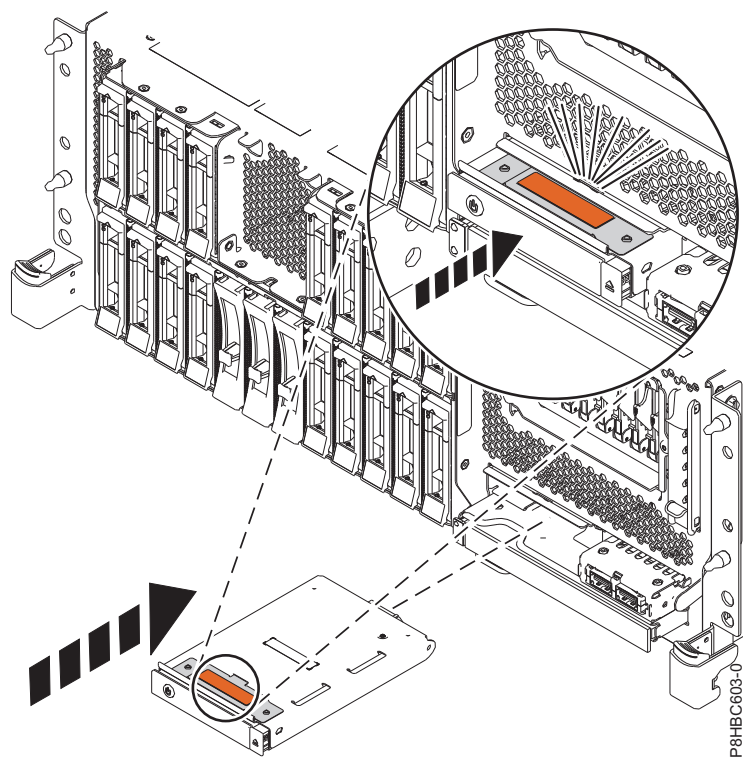
図 8. ラック・マウント型システムのコントロール・パネルの再取り付け
