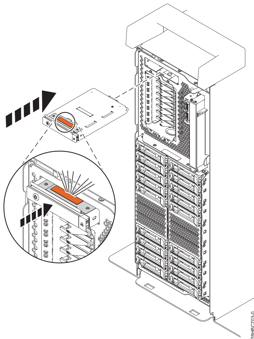
図 9. スタンドアロン・システムのコントロール・パネルの再取り付け
