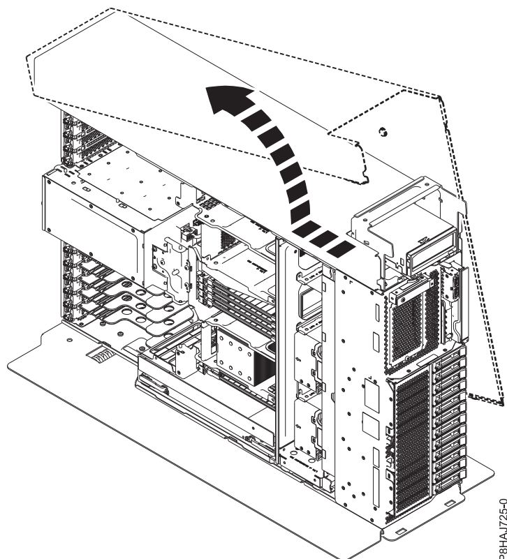
図 18. 8286-41A のサイド・カバーの取り外し
