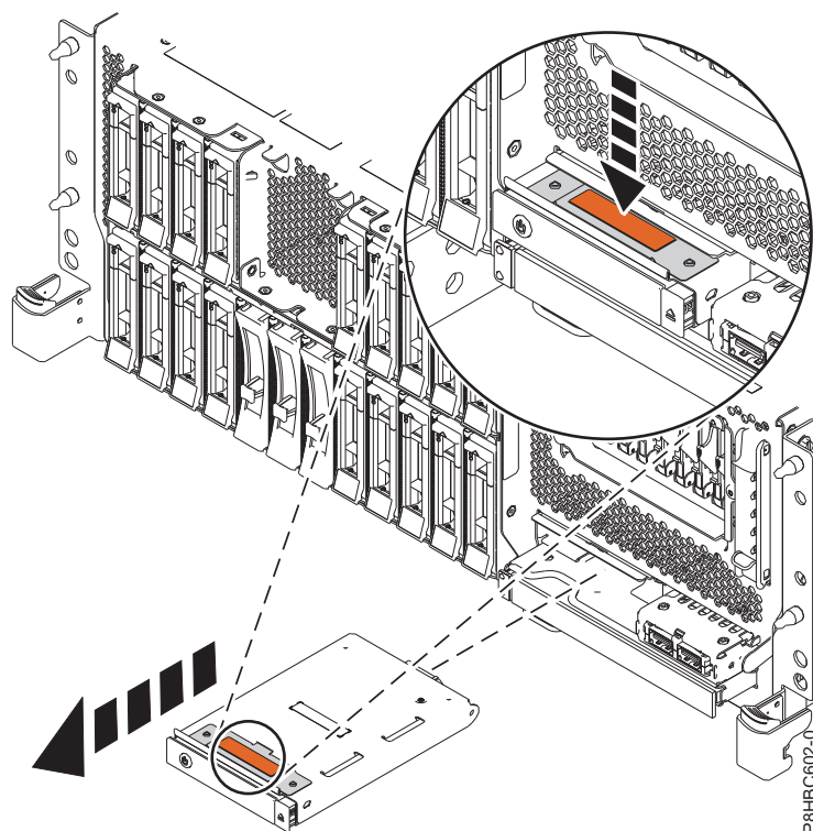
図 6. ラック・マウント型システムのコントロール・パネルの取り外し
