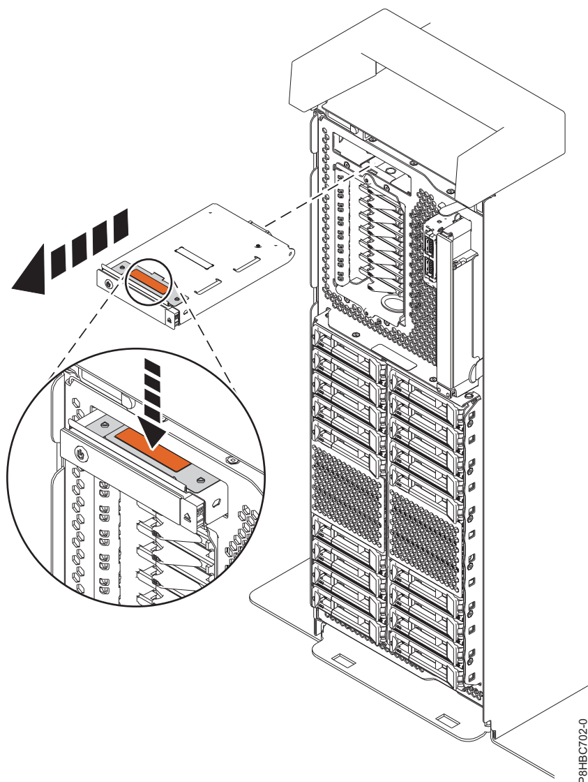
図 7. スタンドアロン型システムのコントロール・パネルの取り外し
