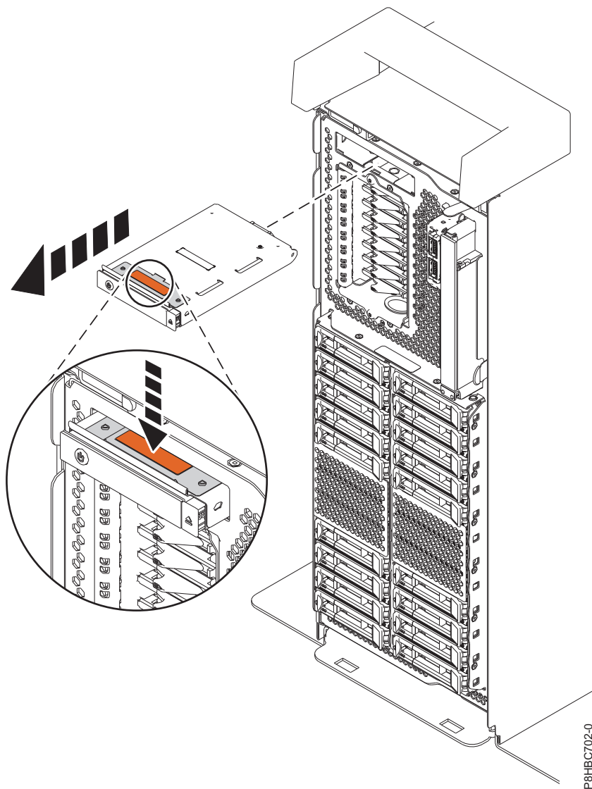
図 2. スタンドアロン型システムのコントロール・パネルの取り外し
