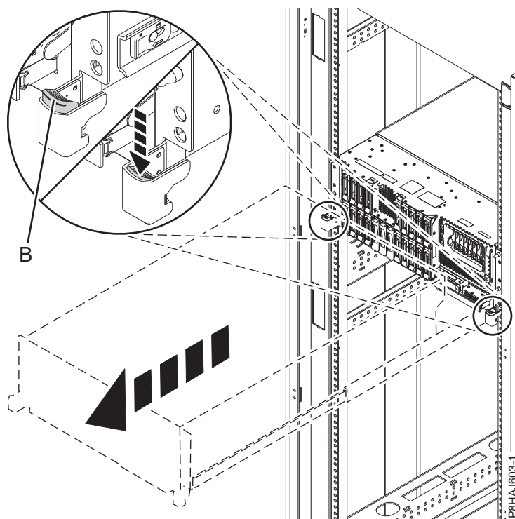
図 36. サイド・ラッチのリリース
