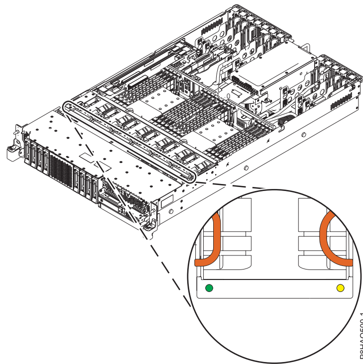
図 1. AMD のファン・ケージ上の LED
