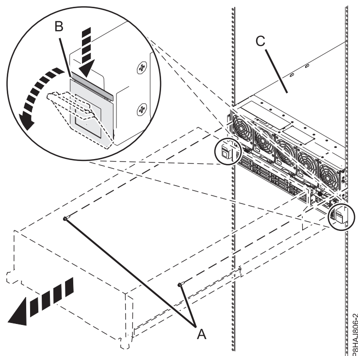
図 46. システムの保守位置への設置
