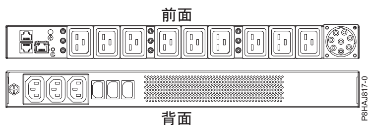
図 56. 8408-44E システムの PDU
