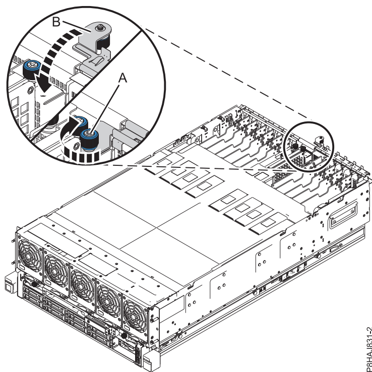
図 38. 入出力ラッチのクローズ
