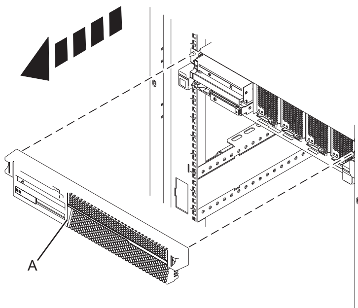
図 40. システム制御装置の前面カバーの取り外し
