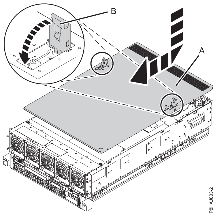
図 34. 保守アクセス・カバーの取り付け
