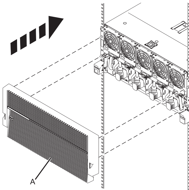
図 41. 前面カバーの取り付け
