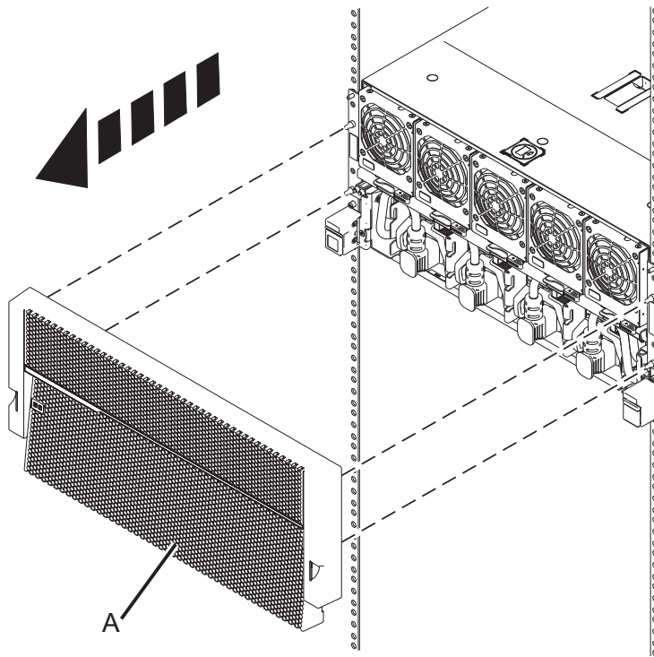
図 39. 前面カバーの取り外し
