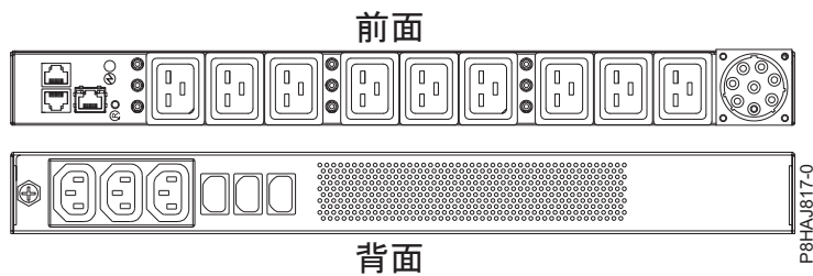
図 50. 8408-44E システムの PDU
