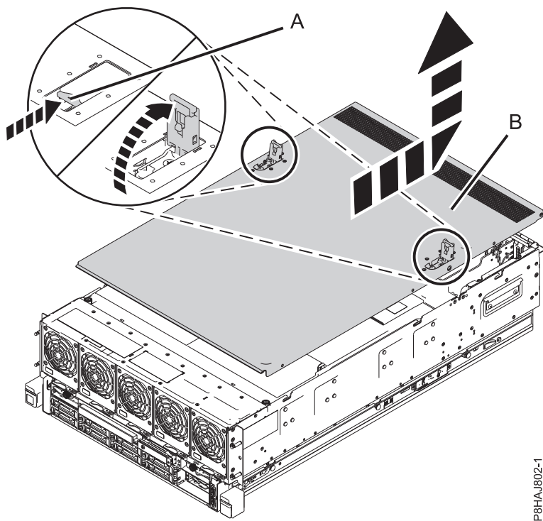
図 33. 保守アクセス・カバーの取り外し
