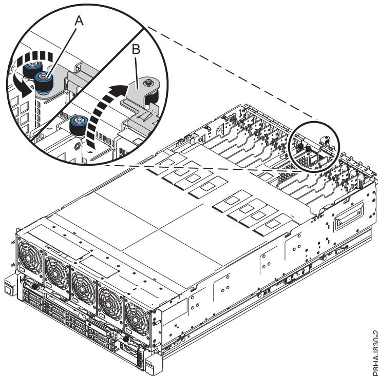
図 37. 入出力ラッチのオープン
