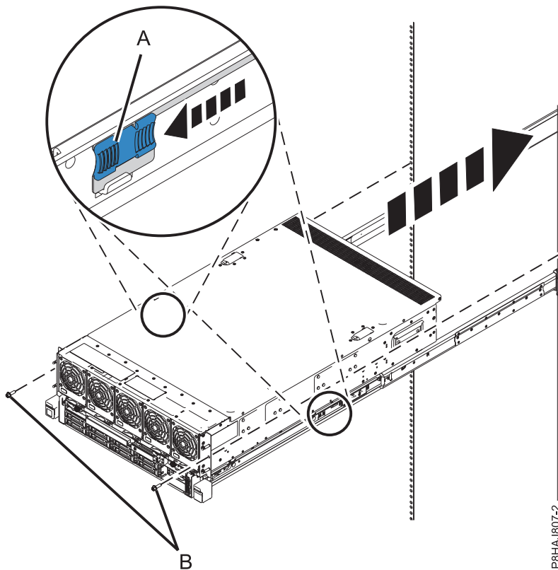
図 47. システムの操作位置への設置
