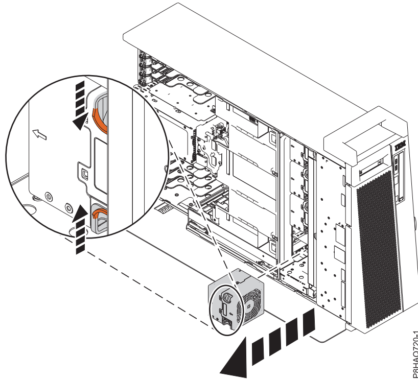
図 4. スタンドアロン型システムからのファンの取り外し
