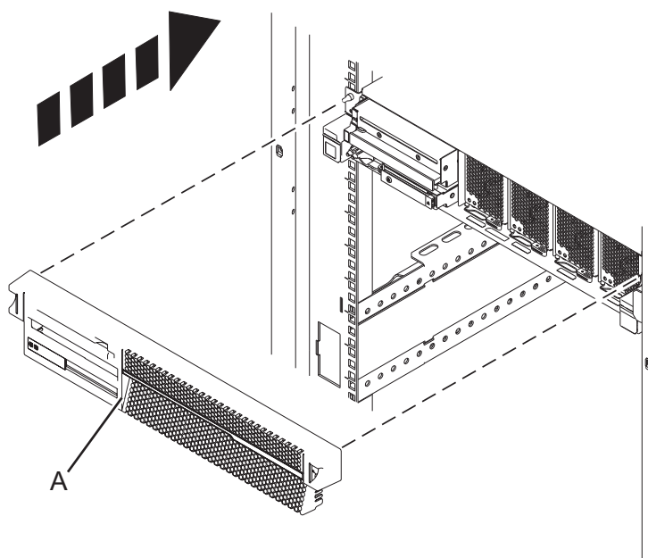
図 47. システム制御装置の前面カバーの取り付け
