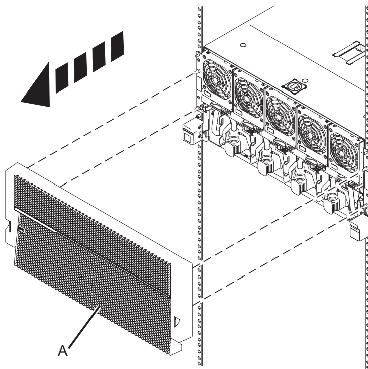
図 44. 前面カバーの取り外し
