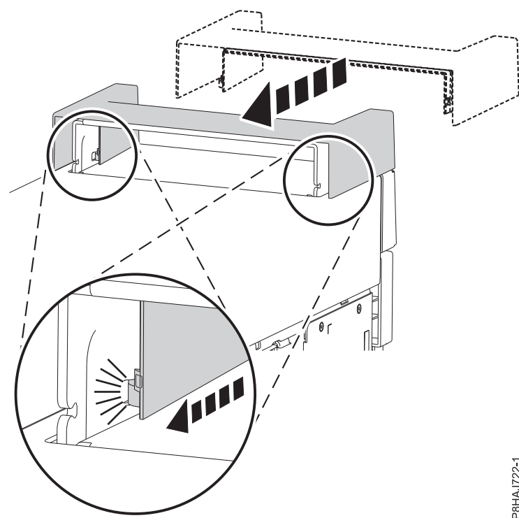
図 24. 8286-41A スタンドアロン・システムへのハンドル・カバーの固定
