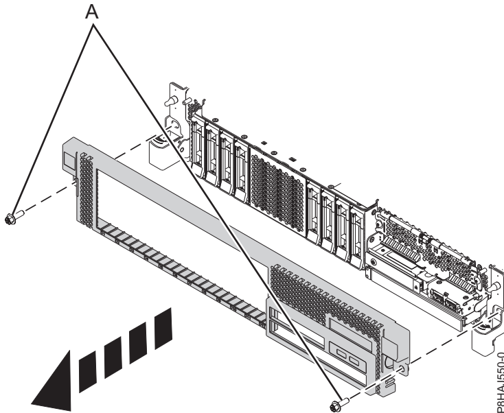
図 13. 前面カバーの取り外し
