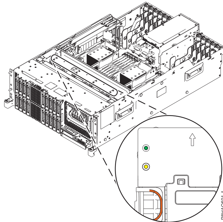
図 1. ラック・マウント型システムでの AMD のファン・ケージ上の LED
