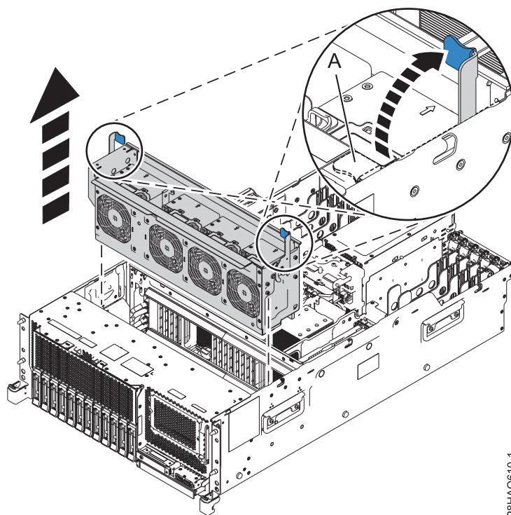
図 7. ラック・マウント型システムからのファン・ケージの取り外し
