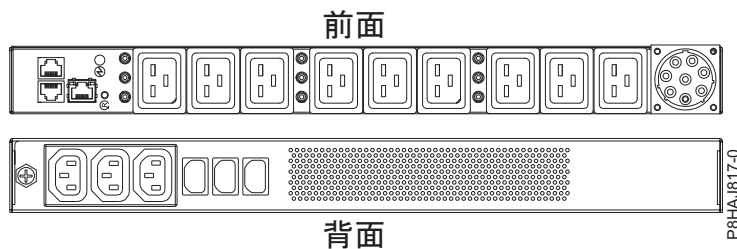
図 55. 8408-44E システムの PDU
