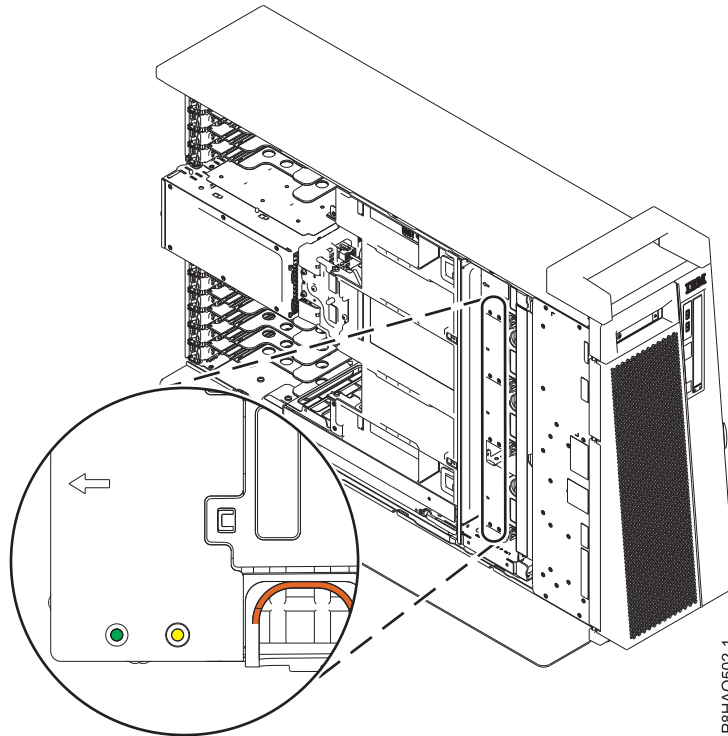
図 2. スタンドアロン型システムでの AMD のファン・ケージ上の LED
