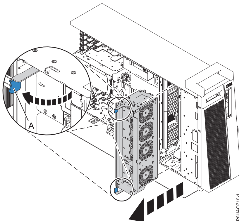
図 8. スタンドアロン型システムからのファン・ケージ・アセンブリーの取り外し
