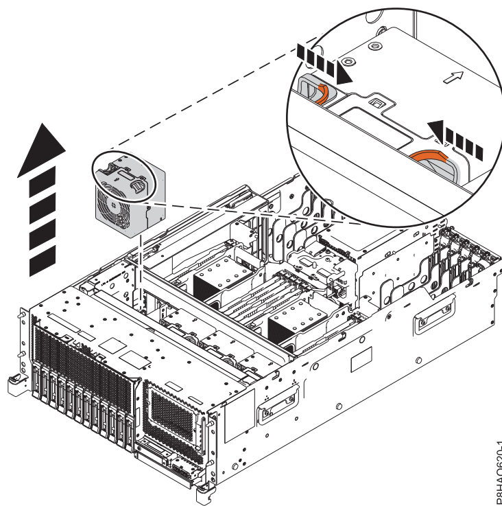
図 3. ラック・マウント型システムからのファンの取り外し
