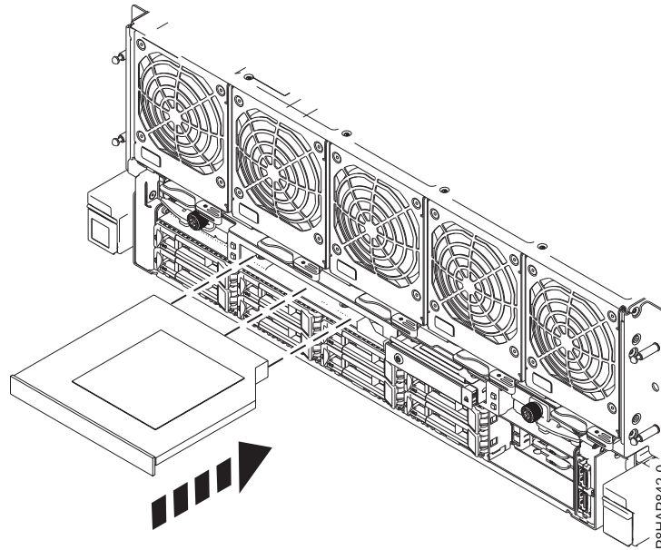
図 2. システムへのDVD ドライブの取り付け
