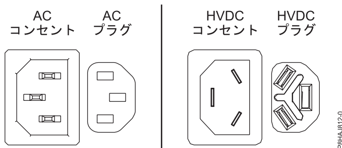
図 32. AC コネクターと HVDC コネクター
