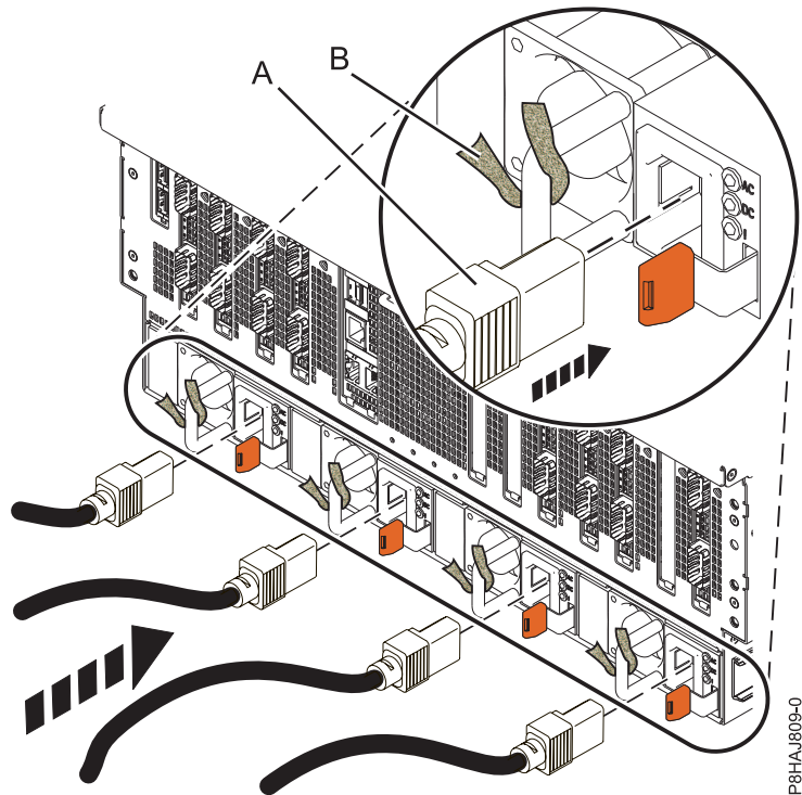
図 37. 8408-44E または 8408-E8E システムへの電源コードの接続
