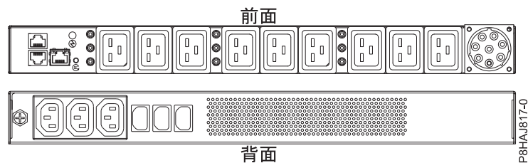
図 28. 8408-44E システムの PDU
