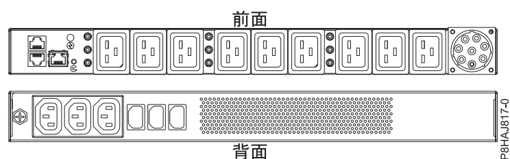
図 34. 8408-44E システムの PDU
