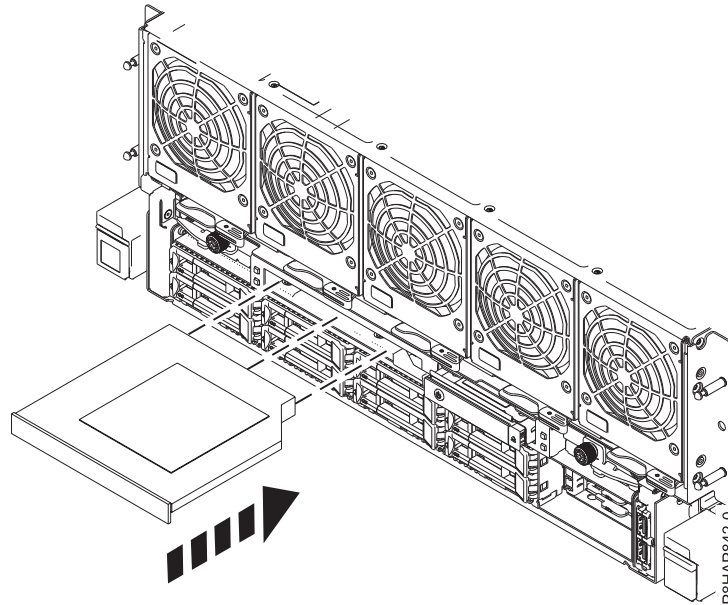
図 6. システムへのDVD ドライブの取り付け
