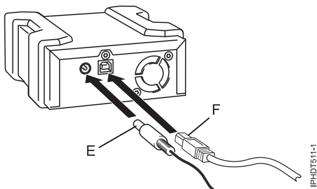
図 13. USB ケーブルおよび電源ケーブルの接続
