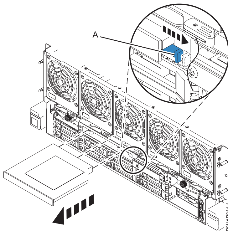
図 7. システムからのDVD ドライブの取り外し
