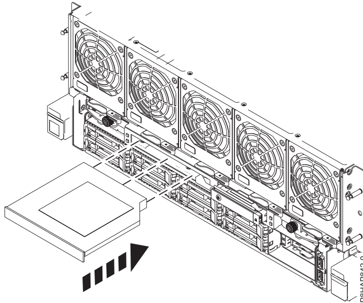
図 12. システムへのDVD ドライブの取り付け
