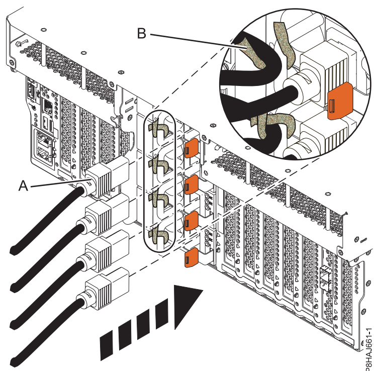
図 35. 8247-42L、8286-41A、または 8286-42A システムへの電源コードの接続
