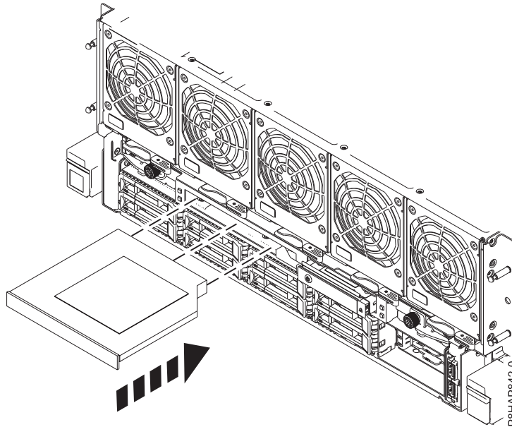
図 8. システムへのDVD ドライブの取り付け
