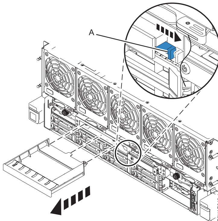
図 1. システムからのメディア・デバイス・フィラーの取り外し
