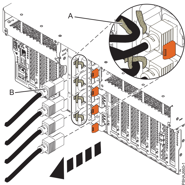
図 29. 8247-42L、8286-41A、または 8286-42A システムからの電源コードの取り外し
