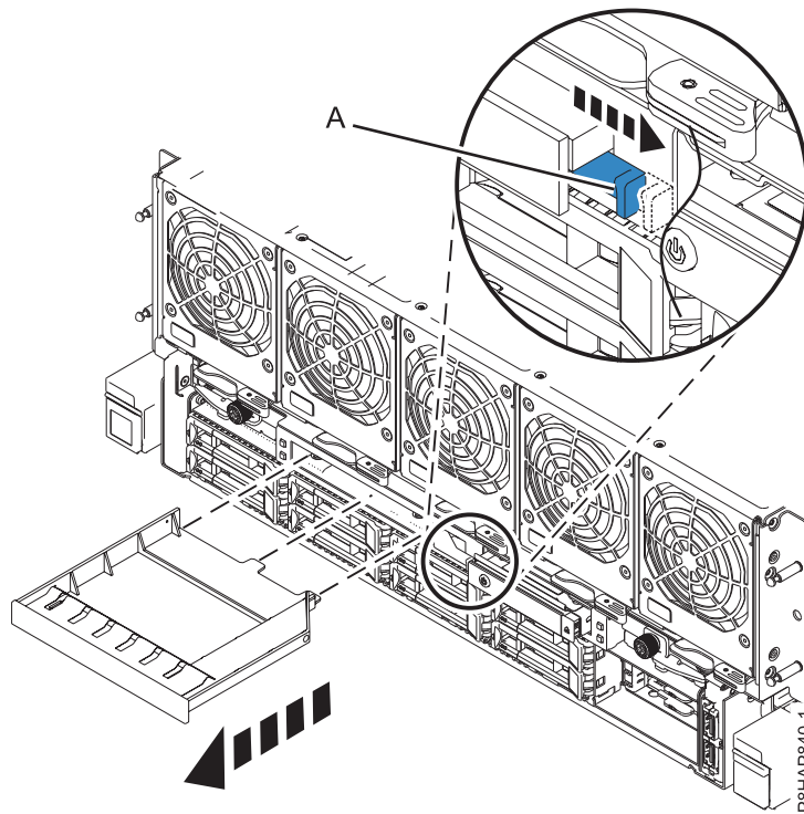
図 3. システムからのメディア・デバイス・フィラーの取り外し
