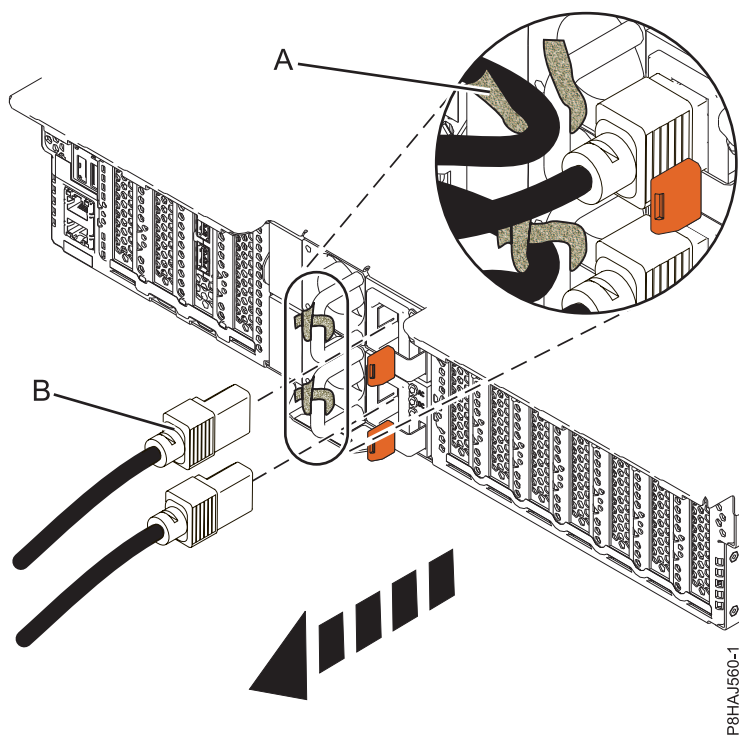
図 30. 5148-21L、5148-22L、8247-21L、8247-22L、8284-21A、または 8284-22A システムからの電源コードの取り外し
