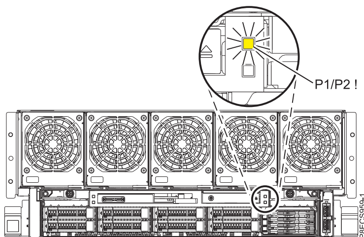
図 2. 8408-44E または 8408-E8E システム上の前面 P1/P2 ! 障害ロールアップ LED
