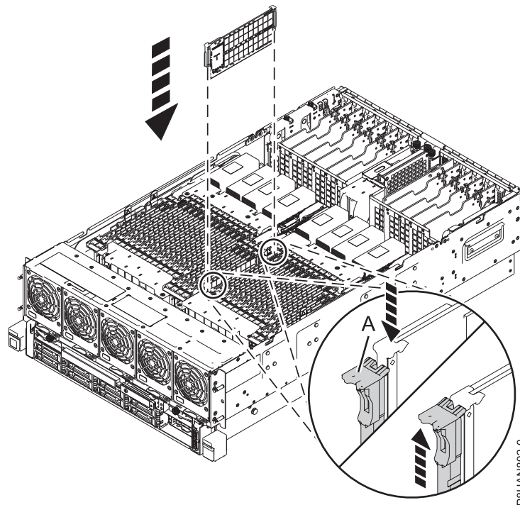
図 11. システムのメモリーの取り替え
