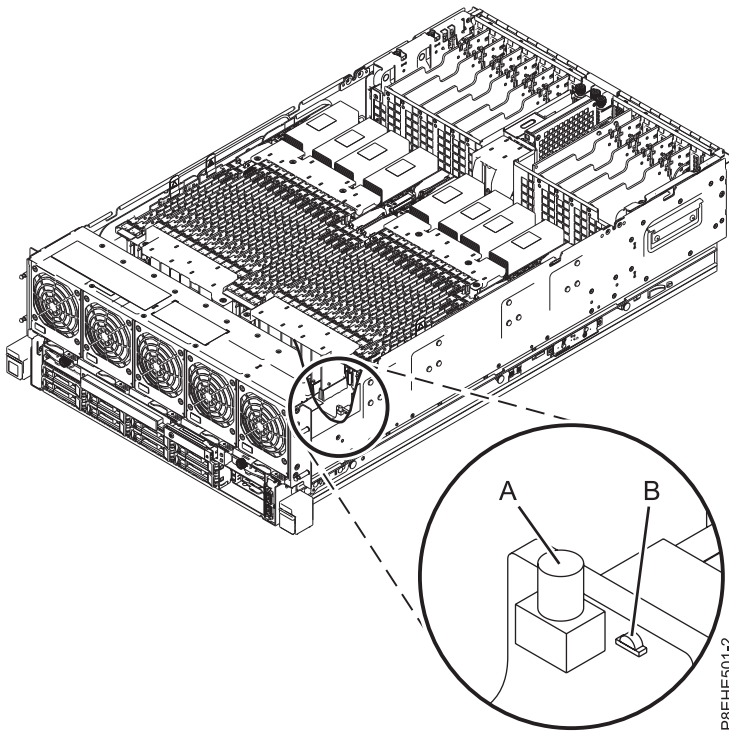
図 8. 識別 LED の活動化
