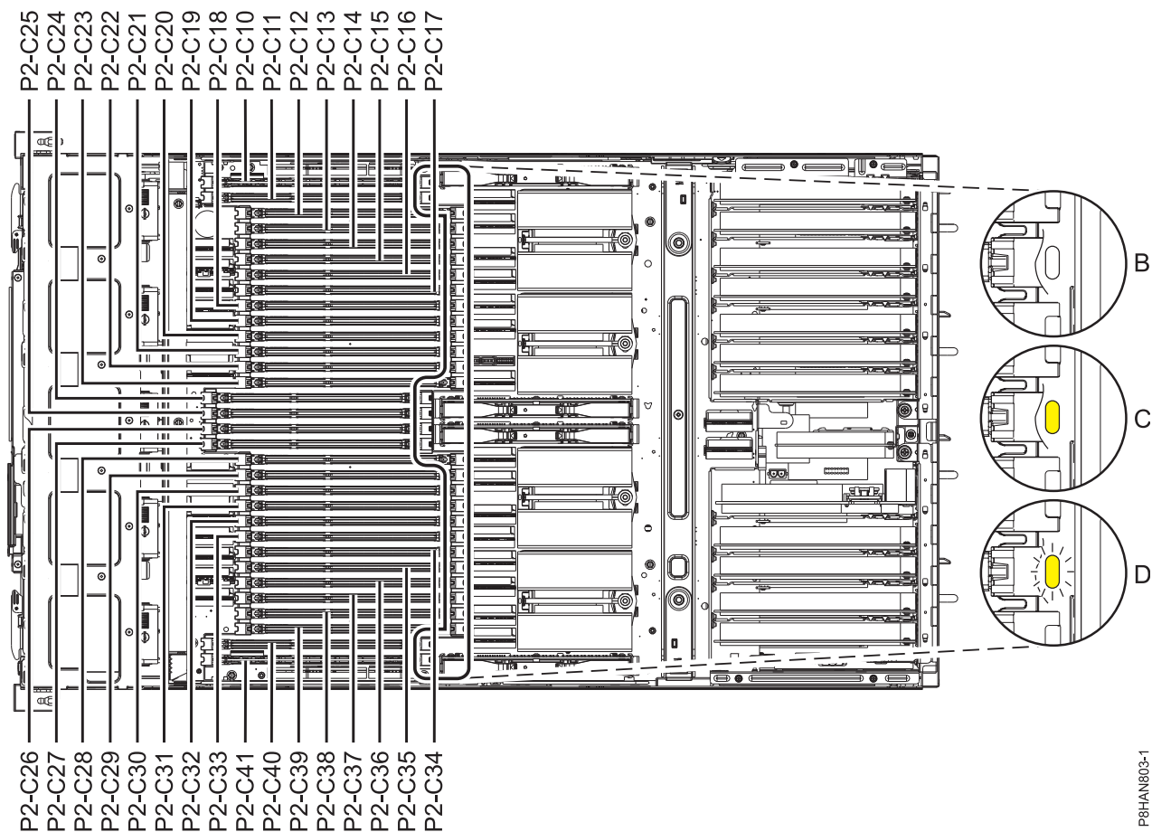
図 4. メモリー・スロットおよび LED の位置
