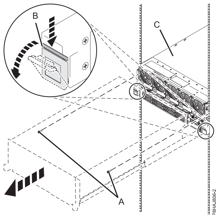
図 35. システムの保守位置への設置
