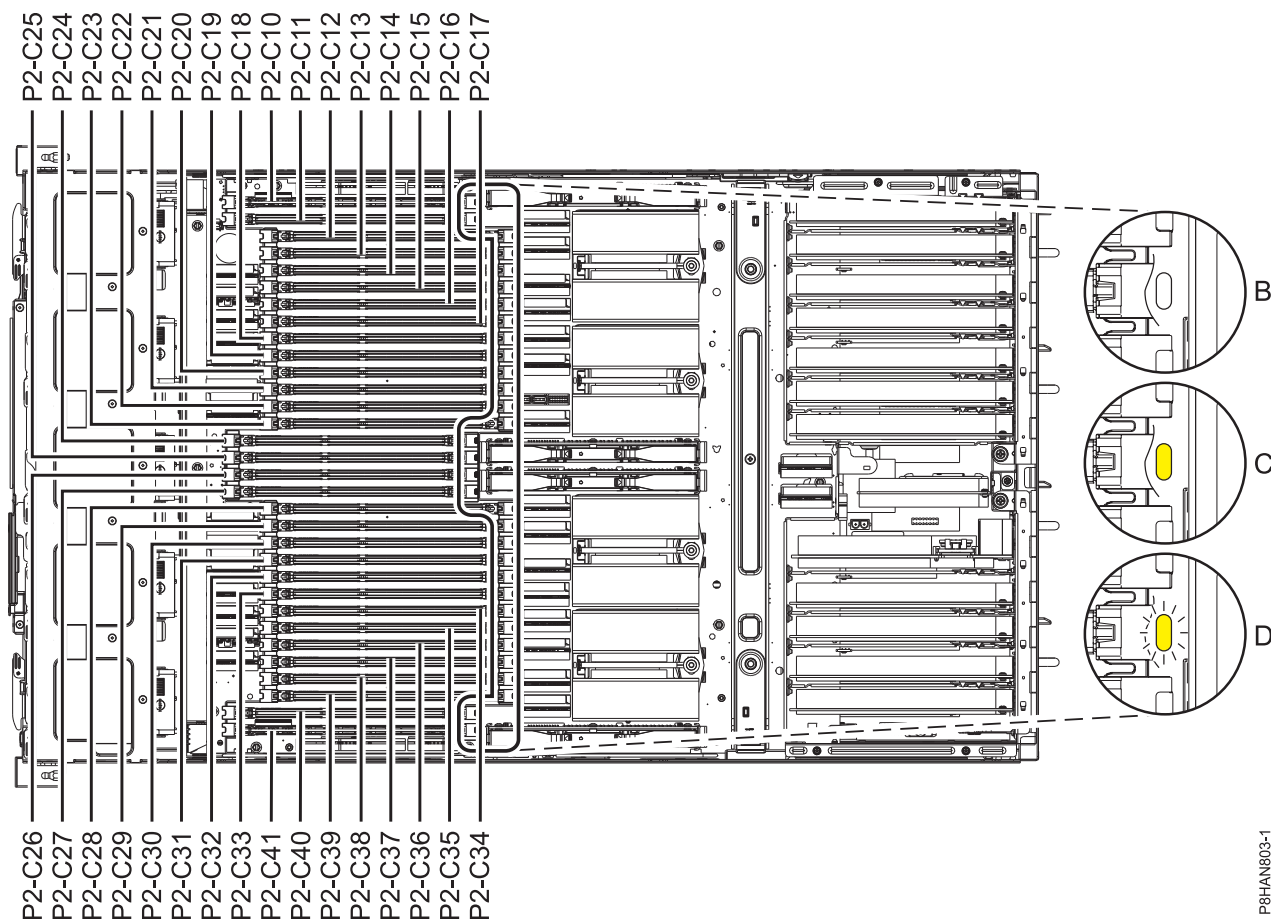
図 9. メモリー・スロットおよび LED の位置
