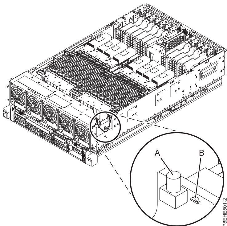
図 3. 識別 LED の活動化
