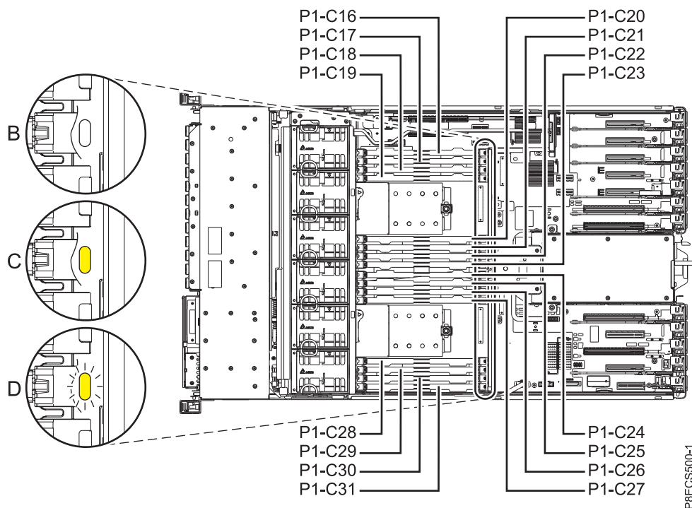
図 4. 5148-21L、5148-22L、8247-21L、8247-22L、8284-21A、または 8284-22A システムのメモリー・モジュールの位置およびサービス・インジケータ
