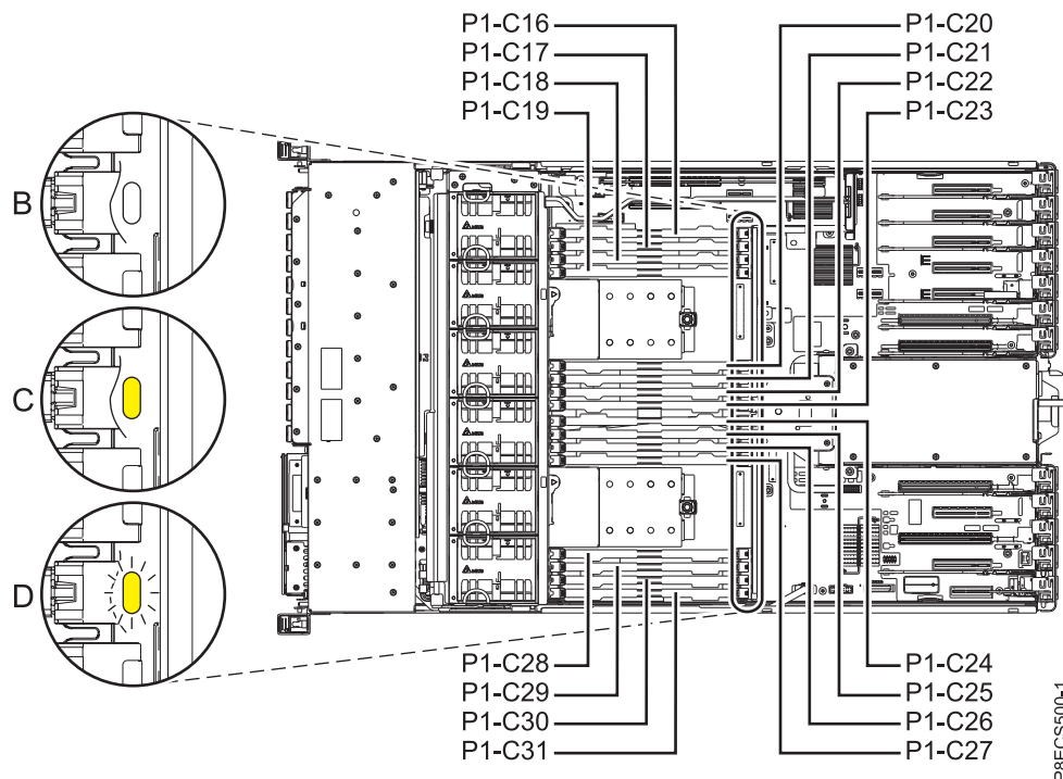
図 1. 5148-21L、5148-22L、8247-21L、8247-22L、8284-21A、または 8284-22A システムのメモリー・モジュールの位置およびサービス・インジケータ
