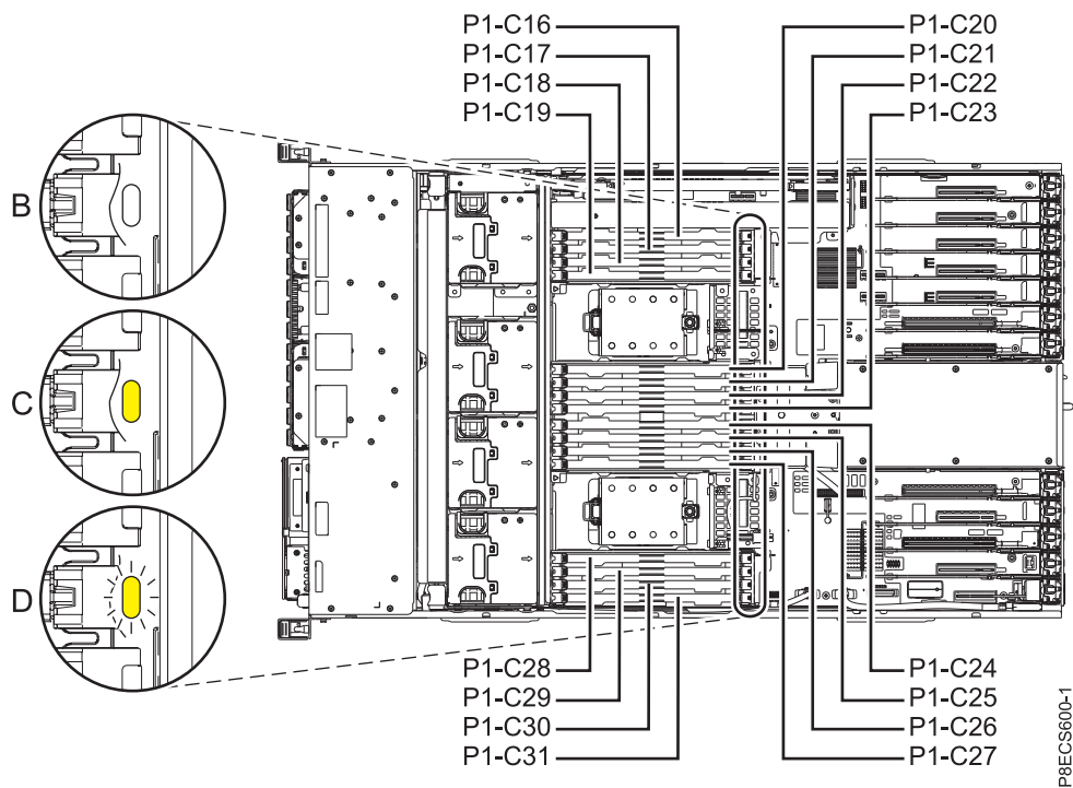
図 5. 動作中であるが、障害が発生したメモリー・モジュールの LED
