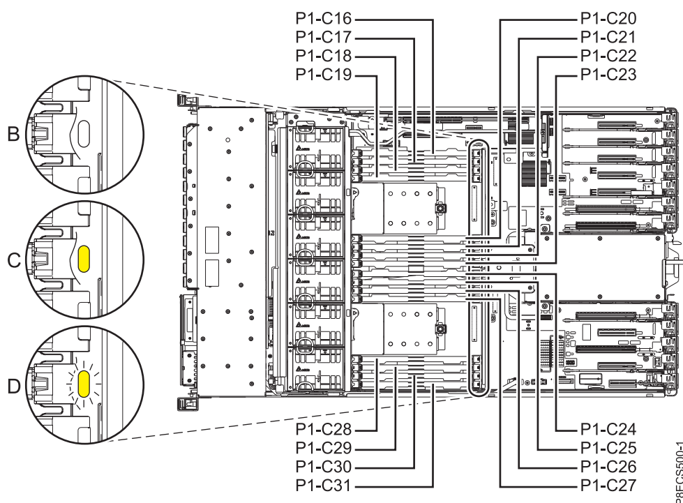
図 10. メモリー・モジュールの差し込み順序
