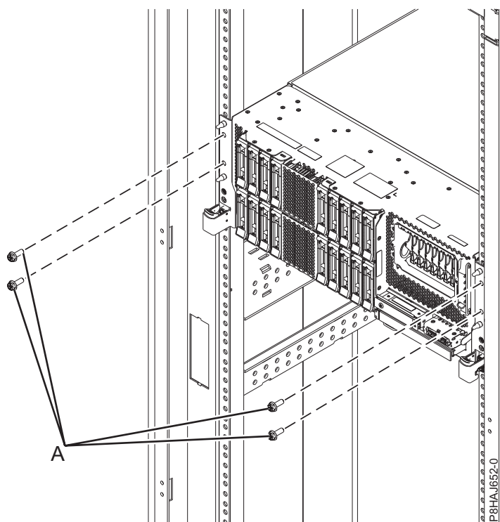
図 48. 前面のねじの取り外し
