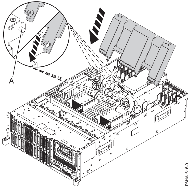
図 47. エア・バッフルの取り替え
