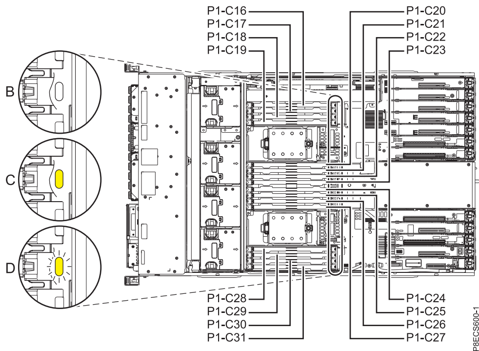
図 1. 8247-42L、8286-41A、または 8286-42A システムのメモリー・モジュールの位置およびサービス・インジケータ
