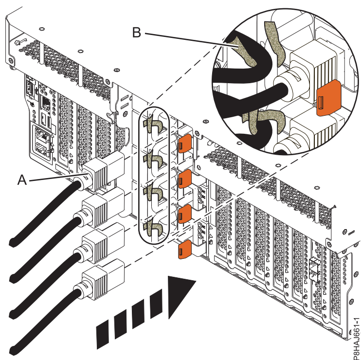
図 22. 8247-42L、8286-41A、または 8286-42A システムへの電源コードの接続
