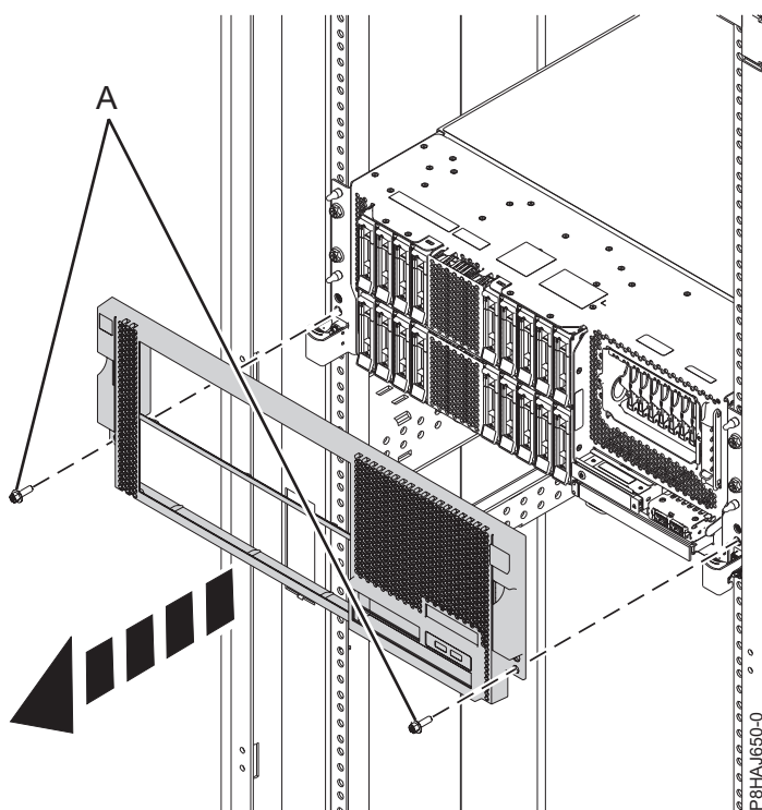
図 26. 前面カバーの取り外し
