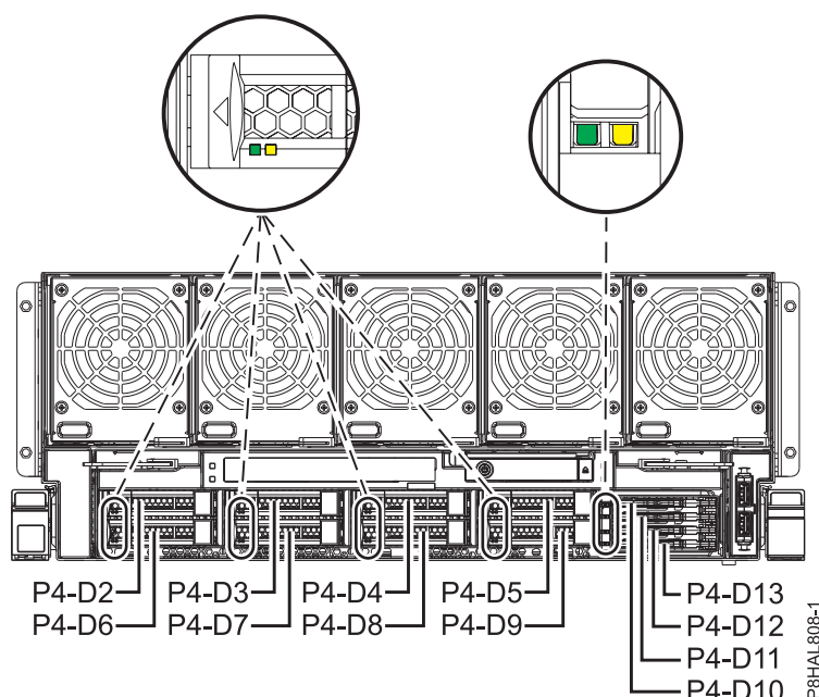
図 26. 8408-44E または 8408-E8E システムのディスク・ドライブとサービス・インジケータの位置
