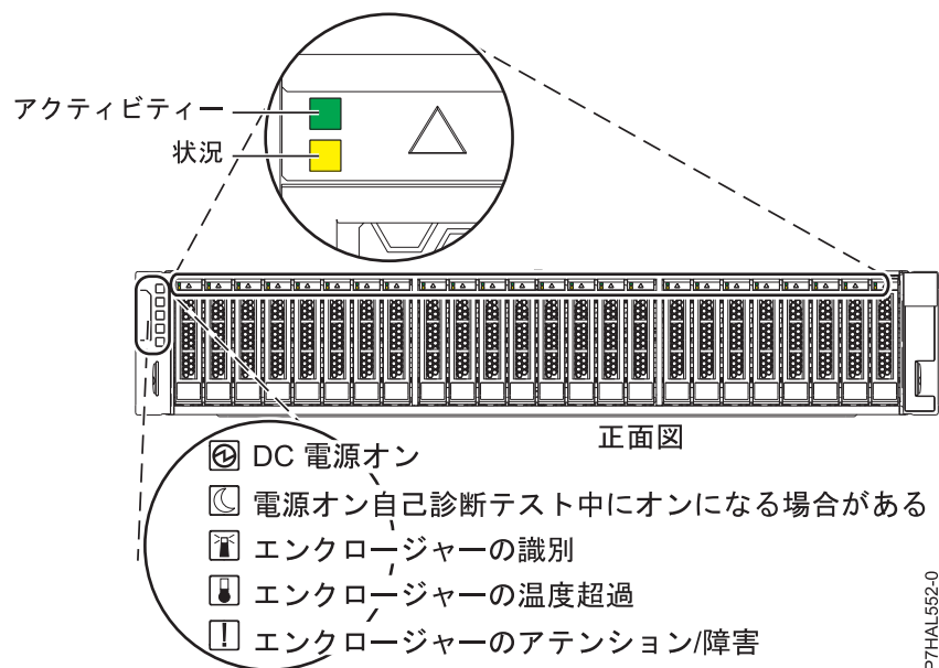
図 44. 5887 ディスク・ドライブ・エンクロージャーの正面図 (サービス・インジケータを示す)
