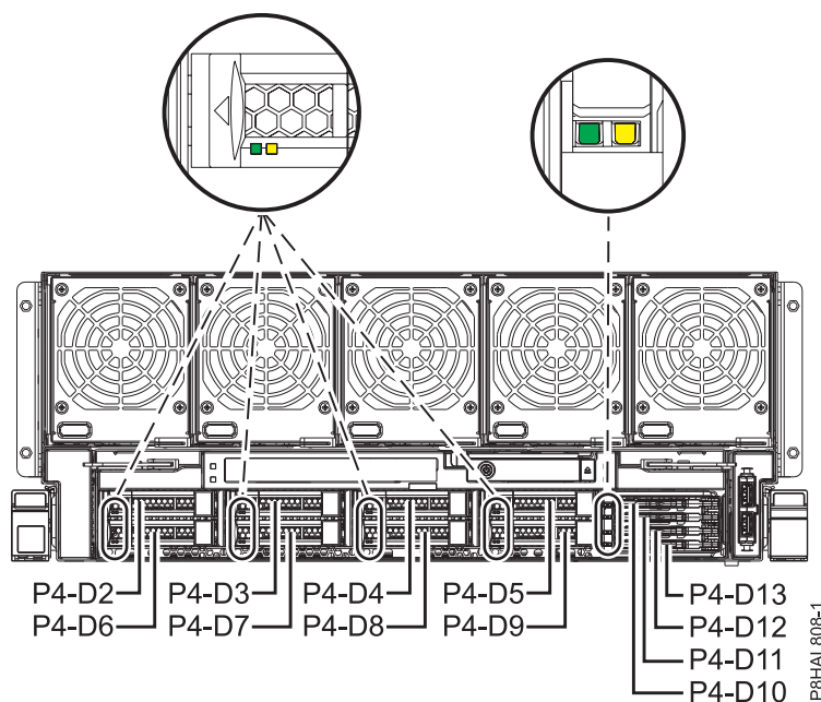
図 10. システムのディスク・ドライブおよびソリッド・ステート・ドライブの位置およびサービス・インジケータ
