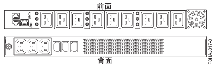
図 61. 8408-44E システムの PDU
