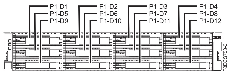
図 45. ESLL ストレージ・エンクロージャーの正面図 (ディスク・ドライブの位置を示す)
