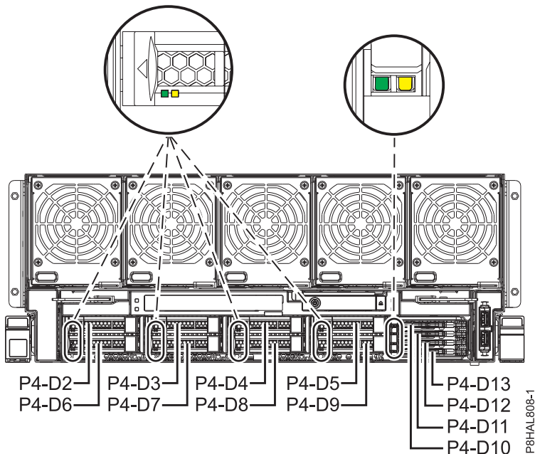
図 16. 8408-44E または 8408-E8E システムのディスク・ドライブとサービス・インジケータの位置
