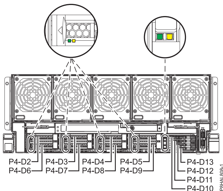
図 41. 8408-44E または 8408-E8E システムのディスク・ドライブと SSD およびサービス・インジケータの位置
