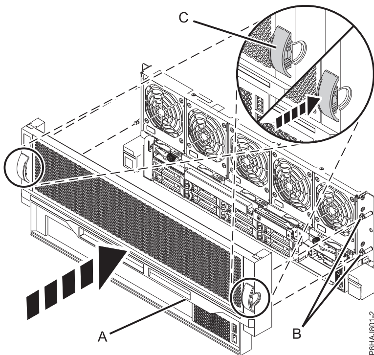
図 66. 前面カバーの取り付け
