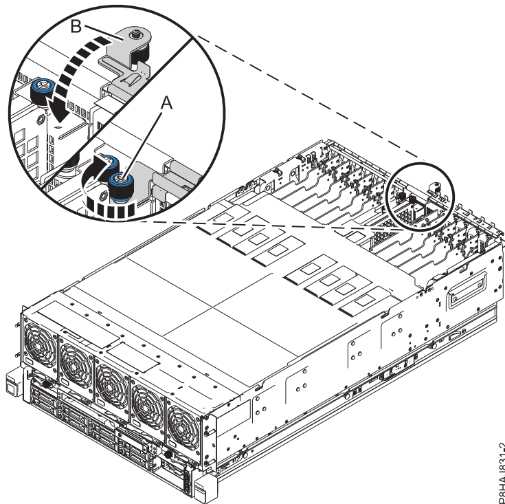
図 72. 入出力ラッチのクローズ
