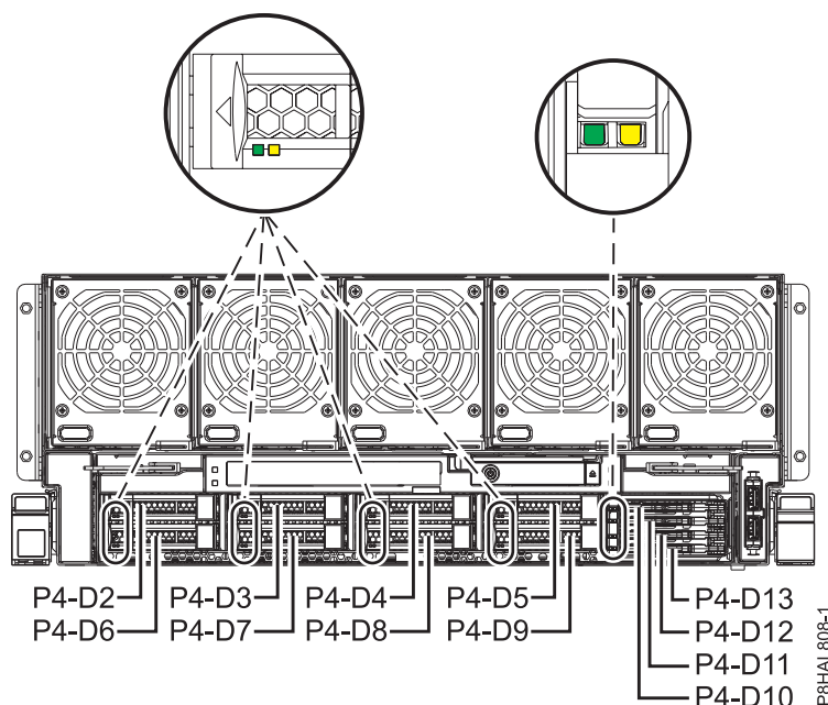
図 6. システムのディスク・ドライブおよびソリッド・ステート・ドライブの位置およびサービス・インジケータ
