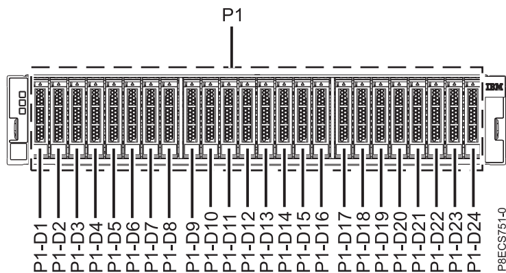
図 46. ESLS ストレージ・エンクロージャーの正面図 (ディスク・ドライブの位置を示す)
