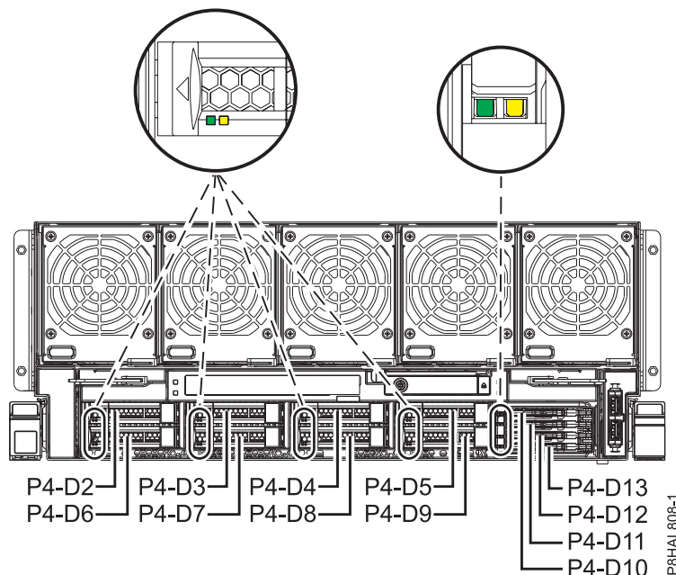
図 1. システムのディスク・ドライブとサービス・インジケータの位置
