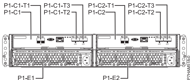
図 43. 5887 ディスク・ドライブ・エンクロージャーの背面図
