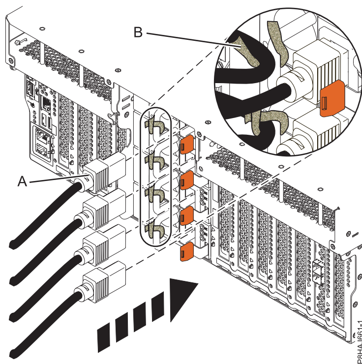
図 62. 8247-42L、8286-41A、または 8286-42A システムへの電源コードの接続
