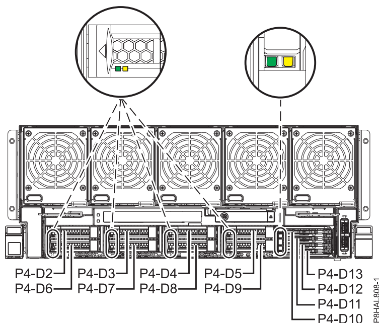
図 4. システムのソリッド・ステート・ドライブの位置およびサービス・インジケータ
