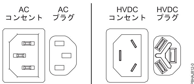
図 53. AC コネクタと HVDC コネクタ
