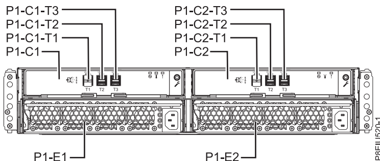
図 47. エンクロージャーの背面図
