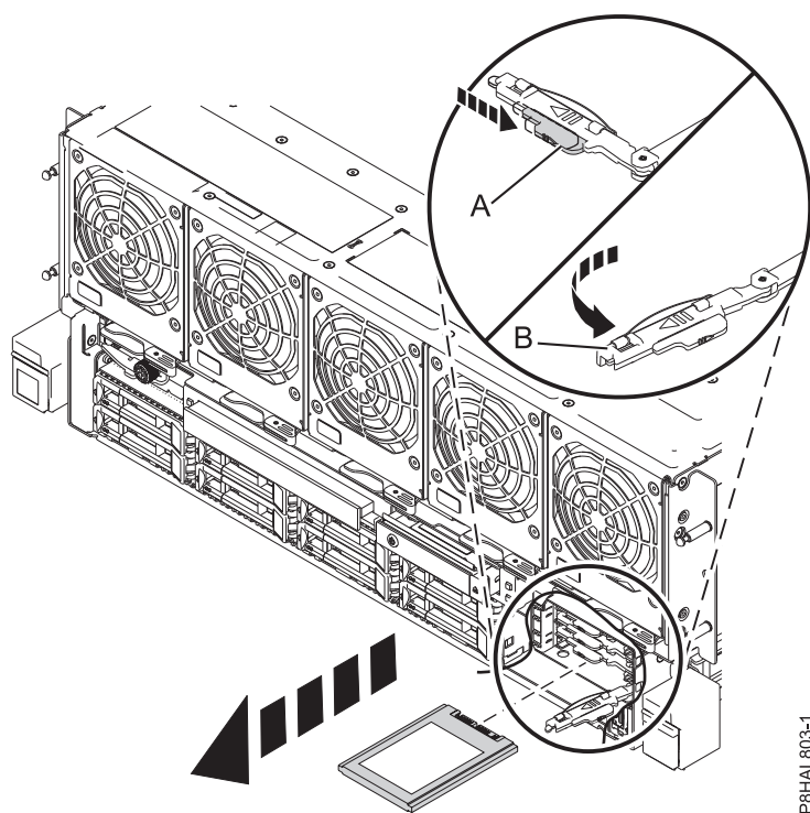
図 23. 8408-44E または 8408-E8E システムからの SSD の取り外し
