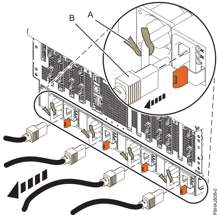
図 58. 8408-44E または 8408-E8E システムからの電源コードの取り外し
