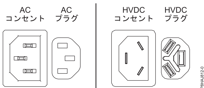
図 59. AC コネクタと HVDC コネクタ
