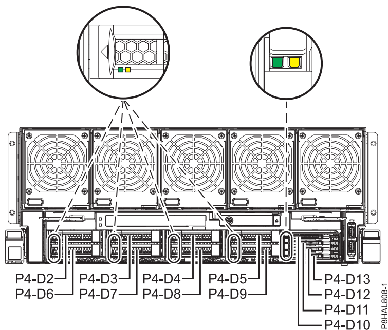
図 63. 8408-44E または 8408-E8E システムのディスク・ドライブと SSD およびサービス・インジケータの位置
