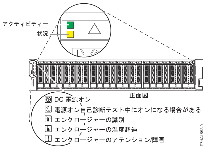
図 17. 5887 ディスク・ドライブ・エンクロージャーの正面図 (サービス・インジケータを示す)
