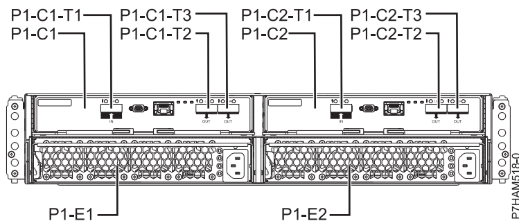
図 39. 5887 ディスク・ドライブ・エンクロージャーの背面図
