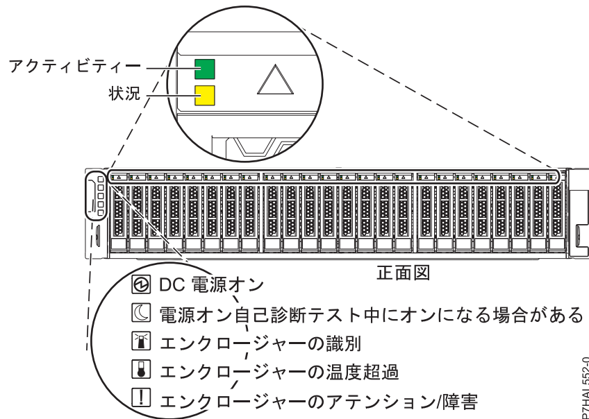
図 3. 5887 ディスク・ドライブ・エンクロージャーの正面図 (サービス・インジケータを示す)
