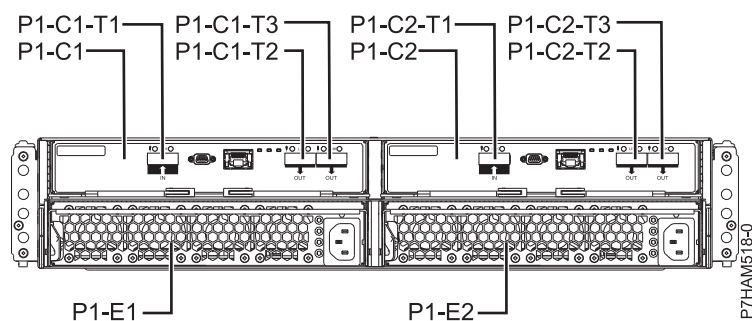
図 2. 5887 ディスク・ドライブ・エンクロージャーの背面図
