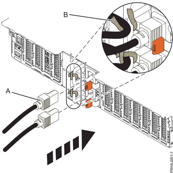
図 81. 5148-21L、5148-22L、8247-21L、8247-22L、8284-21A、または 8284-22A システムへの電源コードの接続
