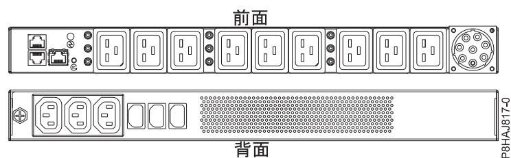
図 73. 8408-44E システムの PDU
