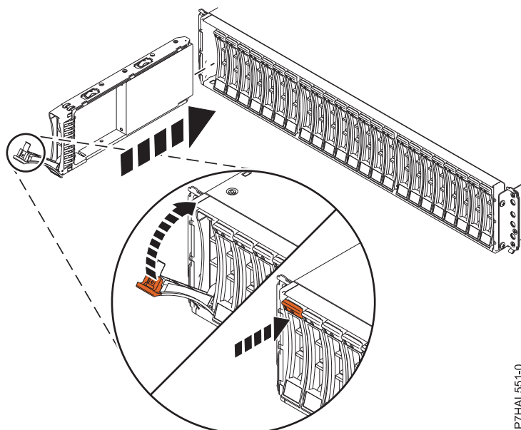
図 44. ディスク・ドライブ・エンクロージャーにおけるディスク・ドライブの取り替え
