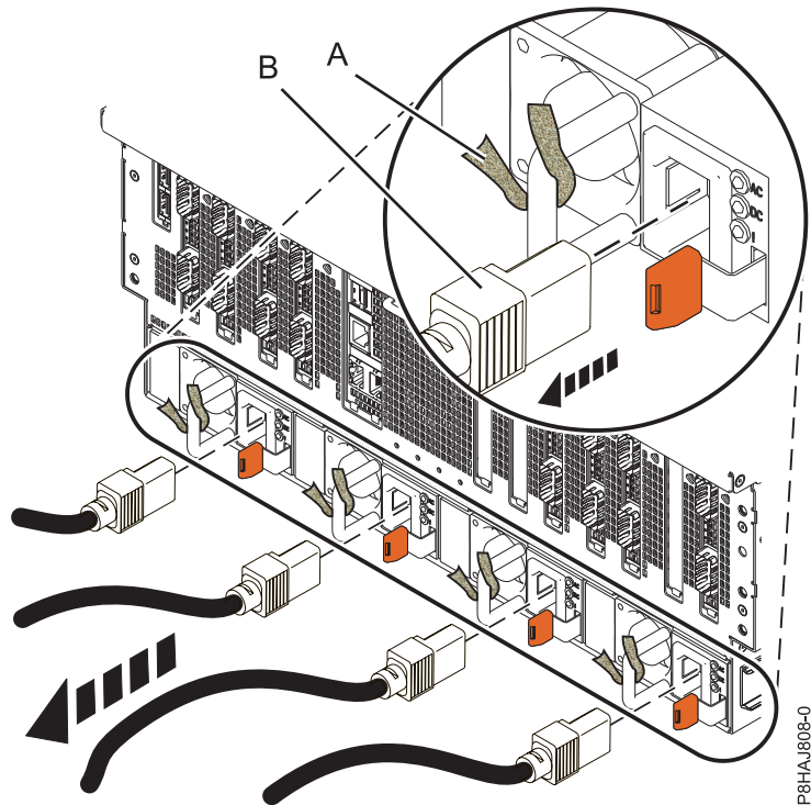
図 76. 8408-44E または 8408-E8E システムからの電源コードの取り外し
