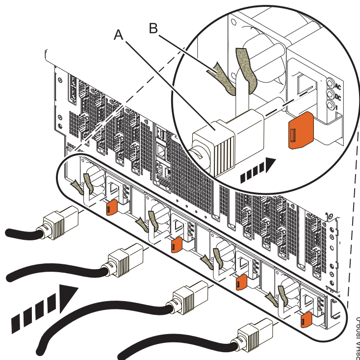
図 82. 8408-44E または 8408-E8E システムへの電源コードの接続
