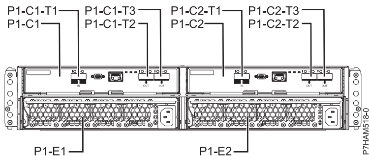
図 16. 5887 ディスク・ドライブ・エンクロージャーの背面図
