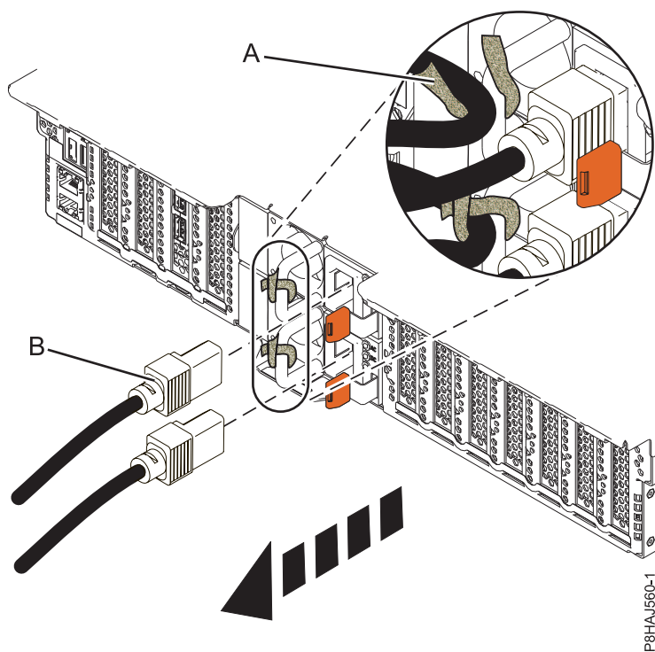
図 75. 5148-21L、5148-22L、8247-21L、8247-22L、8284-21A、または 8284-22A システムからの電源コードの取り外し
