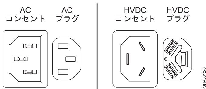
図 77. AC コネクタと HVDC コネクタ
