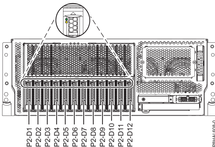
図 59. ラック・マウント型基本機能 8247-42L、8286-41A、または 8286-42A システムのディスク・ドライブまたはソリッド・ステート・ドライブおよびサービス・インジケータの位置
