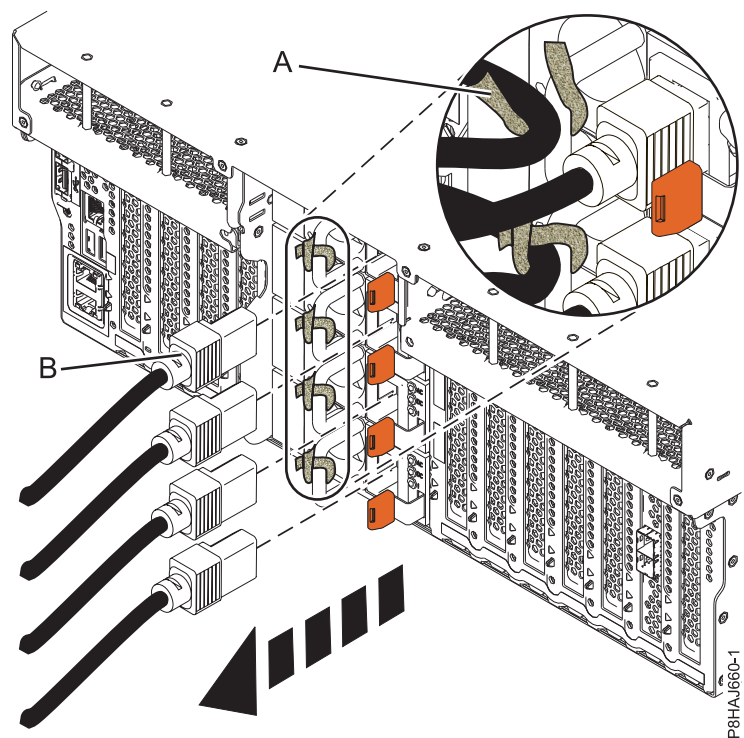
図 74. 8247-42L、8286-41A、または 8286-42A システムからの電源コードの取り外し
