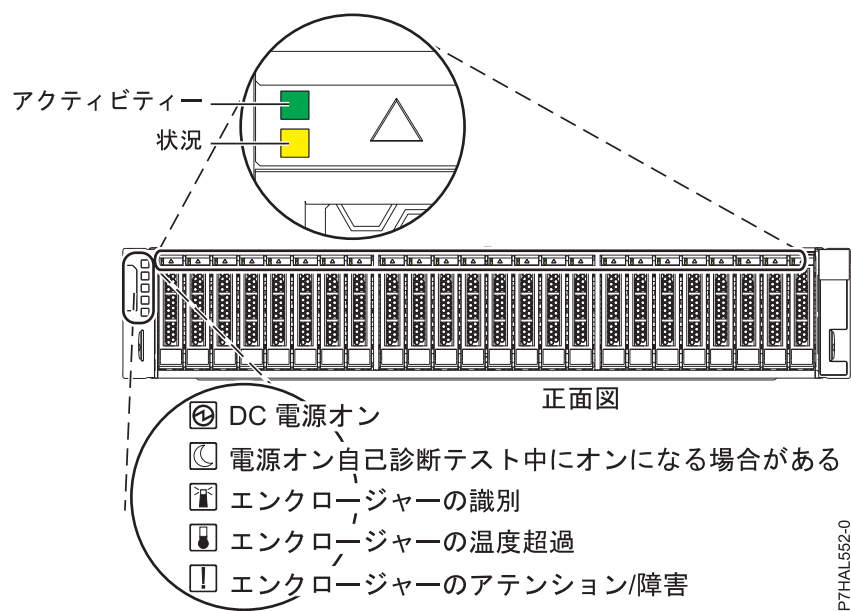
図 11. 5887 ディスク・ドライブ・エンクロージャの正面図 (サービス・インジケータを示す)
