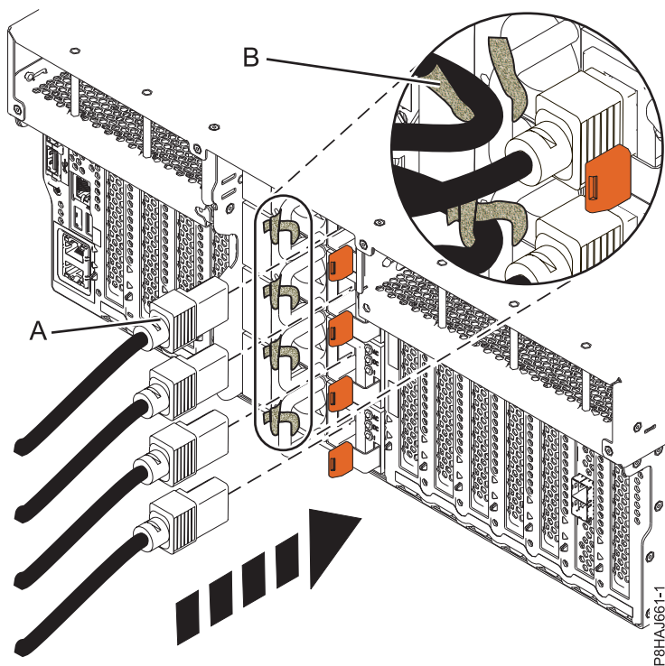
図 80. 8247-42L、8286-41A、または 8286-42A システムへの電源コードの接続
