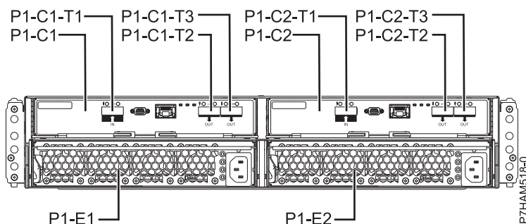
図 27. 5887 ディスク・ドライブ・エンクロージャーの背面図
