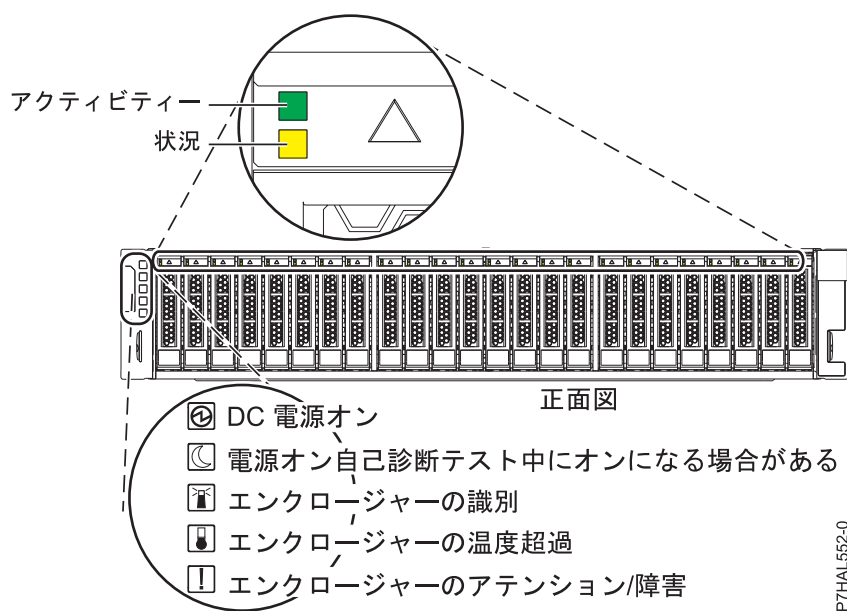
図 47. 5887 ディスク・ドライブ・エンクロージャの正面図 (サービス・インジケータを示す)
