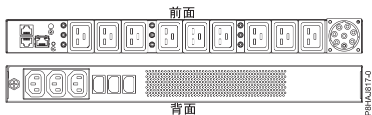
図 79. 8408-44E システムの PDU
