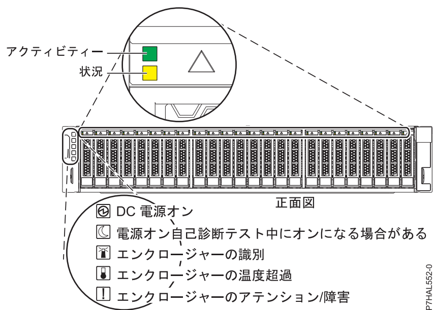
図 66. 5887 ディスク・ドライブ・エンクロージャの正面図 (サービス・インジケータを示す)
