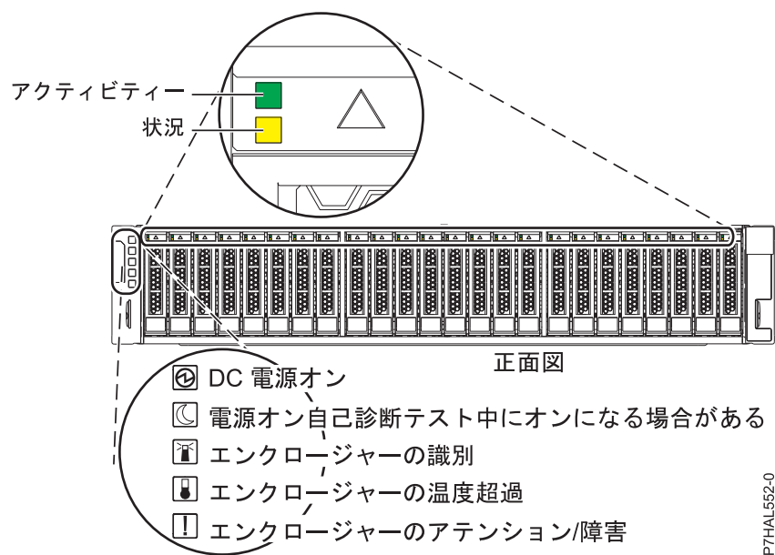
図 40. 5887 ディスク・ドライブ・エンクロージャーの正面図 (サービス・インジケータを示す)
