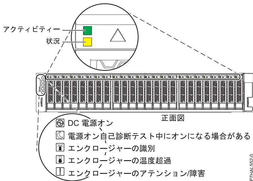
図 7. 5887 ディスク・ドライブ・エンクロージャの正面図 (サービス・インジケータを示す)
