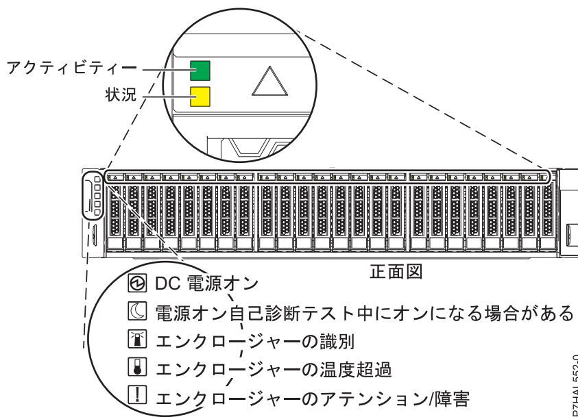
図 33. 5887 ディスク・ドライブ・エンクロージャの正面図 (サービス・インジケータを示す)
