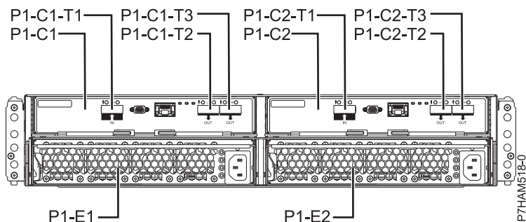
図 22. 5887 ディスク・ドライブ・エンクロージャーの背面図
