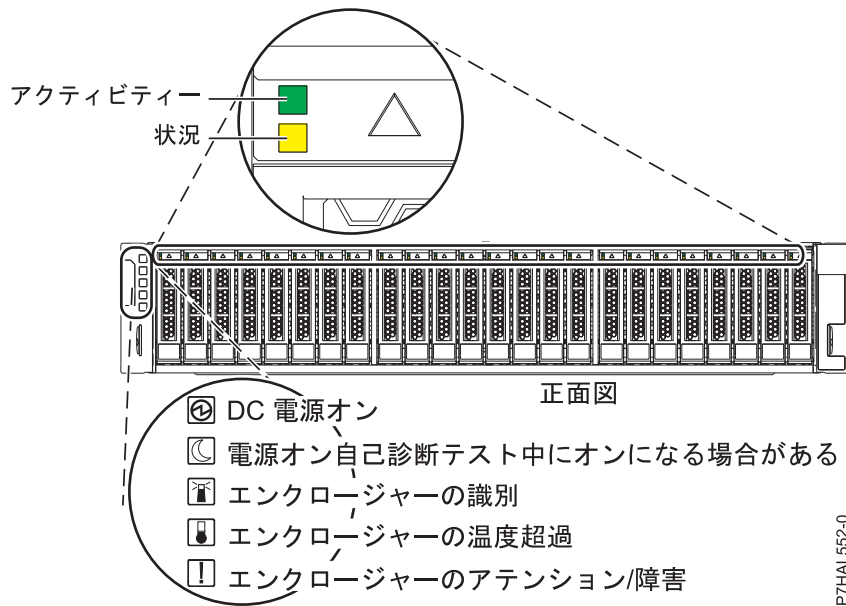
図 28. 5887 ディスク・ドライブ・エンクロージャの正面図 (サービス・インジケータを示す)
