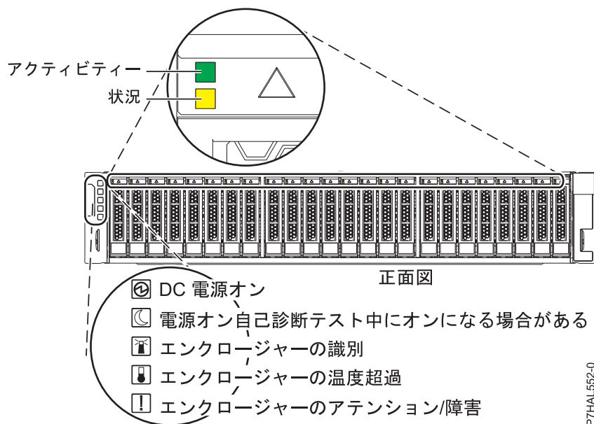
図 23. 5887 ディスク・ドライブ・エンクロージャーの正面図 (サービス・インジケータを示す)
