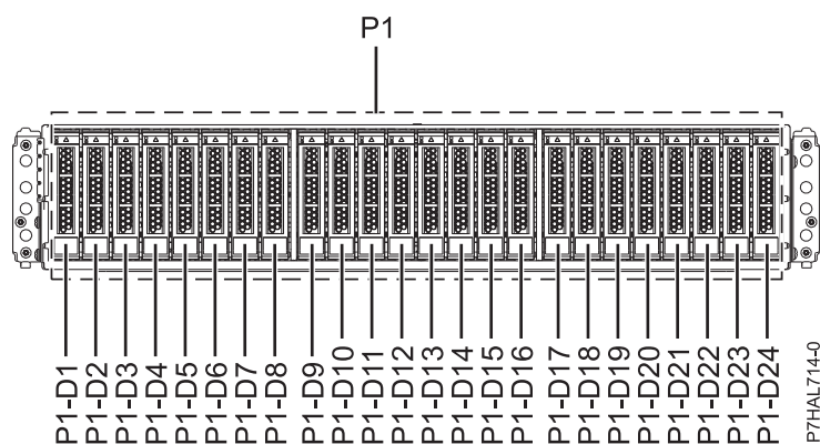
図 64. 5887 ディスク・ドライブ・エンクロージャーの正面図 (ディスク・ドライブの位置を示す)
