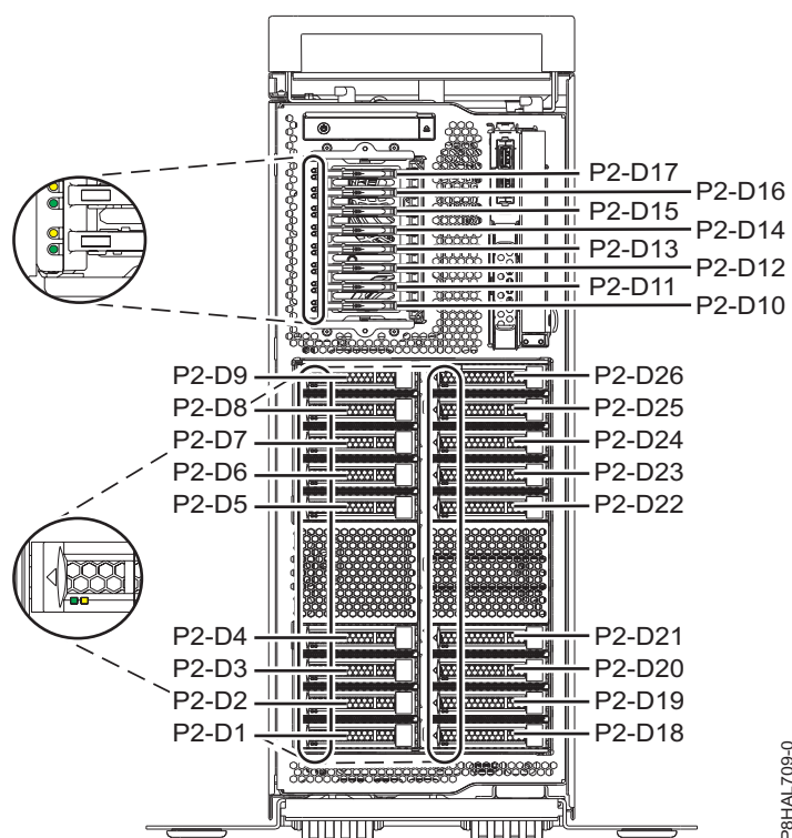
図 62. スタンドアロン型拡張機能 8286-41Aシステムのディスク・ドライブ、ソリッド・ステート・ドライブ、およびサービス・インジケータの位置
