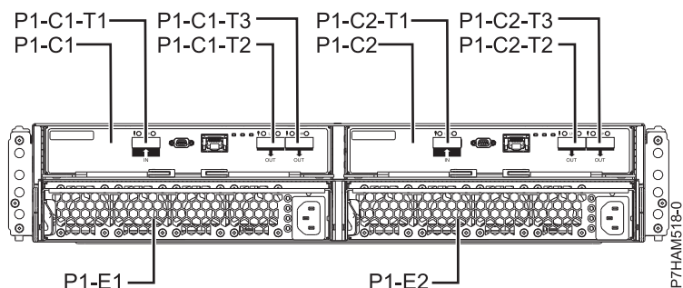
図 65. 5887 ディスク・ドライブ・エンクロージャの背面図
