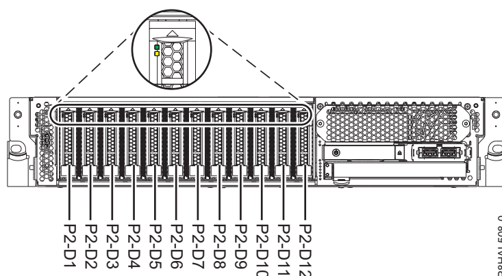
図 57. 基本機能 5148-21L、5148-22L、8247-21L、8247-22L、8284-21A、または 8284-22A システムのディスク・ドライブとサービス・インジケータの位置
