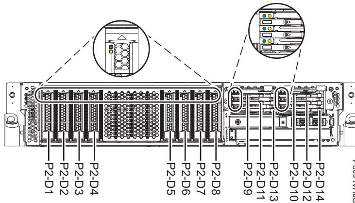
図 58. 拡張機能 5148-21L、5148-22L、8247-21L、8247-22L、8284-21A、または 8284-22A システムのディスク・ドライブ、ソリッド・ステート・ドライブ、およびサービス・インジケータの位置
