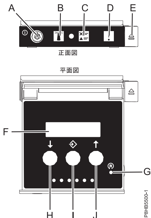
図 69. コントロール・パネルの LED
