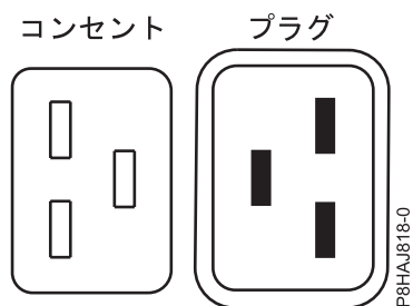
図 72. 8408-44E システムのコネクター
