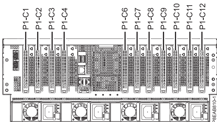
図 5. 8408-44E または 8408-E8E システムの PCIe アダプター・スロットの位置
