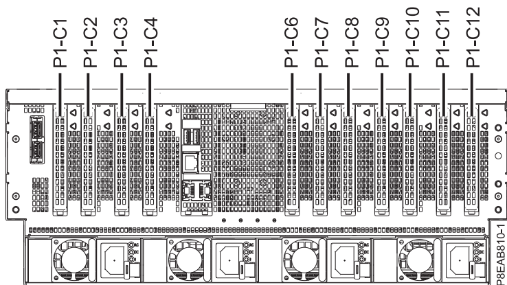
図 1. 8408-44E または 8408-E8E システムの PCIe アダプター・スロットの位置
