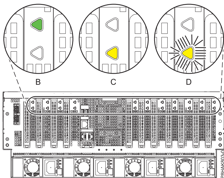
図 14. 8408-44E または 8408-E8E システムでの PCIe アダプター LED の位置
