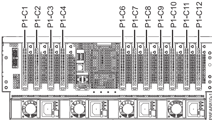
図 9. 8408-44E または 8408-E8E システムの PCIe アダプター・スロットの位置
