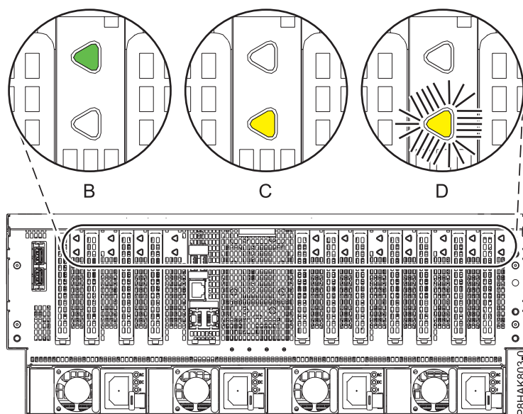
図 25. 8408-44E または 8408-E8E システムでの PCIe アダプター LED の位置
