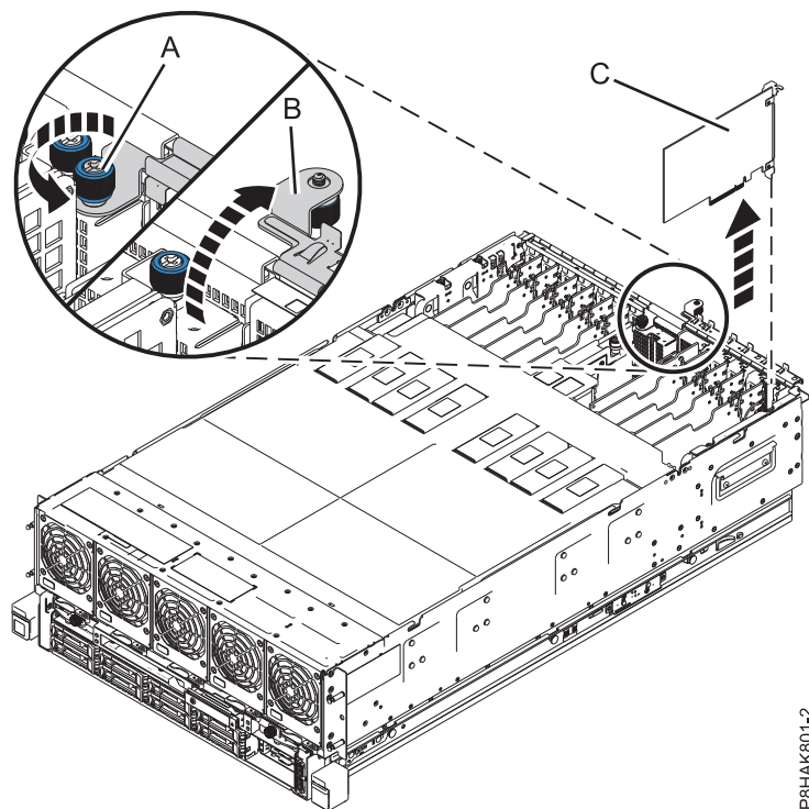
図 26. 8408-44E または 8408-E8E システムからの PCIe アダプターの取り外し
