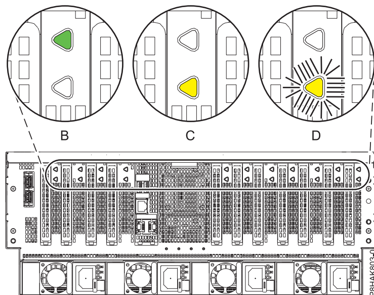
図 6. 8408-44E または 8408-E8E システムでの PCIe アダプター LED の位置
