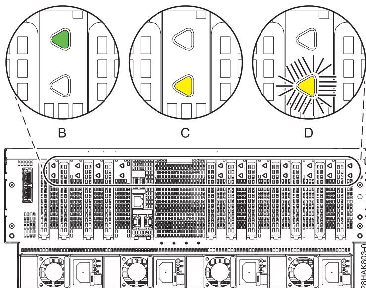
図 20. 8408-44E または 8408-E8E システムでの PCIe アダプター LED の位置
