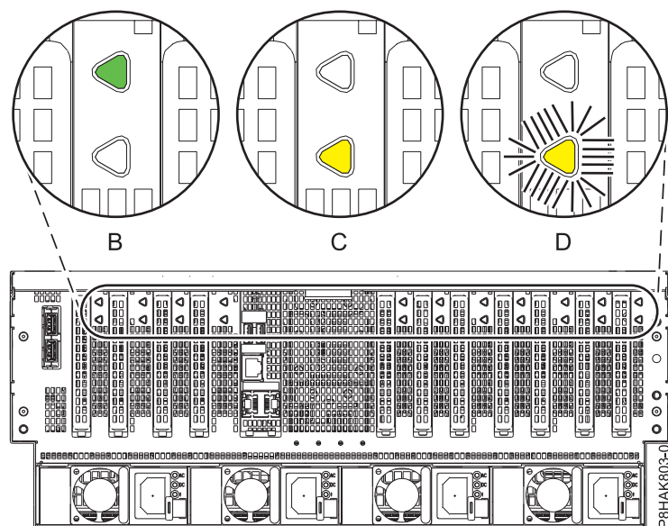
図 10. 8408-44E または 8408-E8E システムでの PCIe アダプター LED の位置
