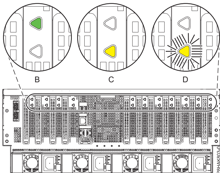
図 2. 8408-44E または 8408-E8E システムでの PCIe アダプター LED の位置
