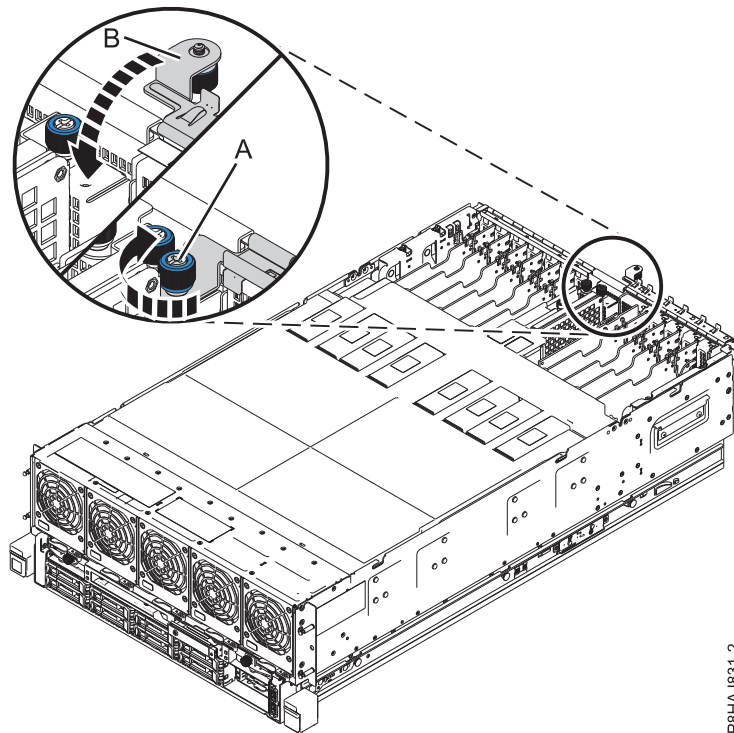
図 43. 入出力ラッチのクローズ
