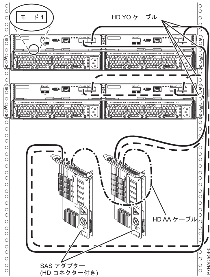
図 82. HD コネクター付きの 2 つの PCIe2 SAS アダプターへの 2 つの 5887 エンクロージャーのモード 1 接続
