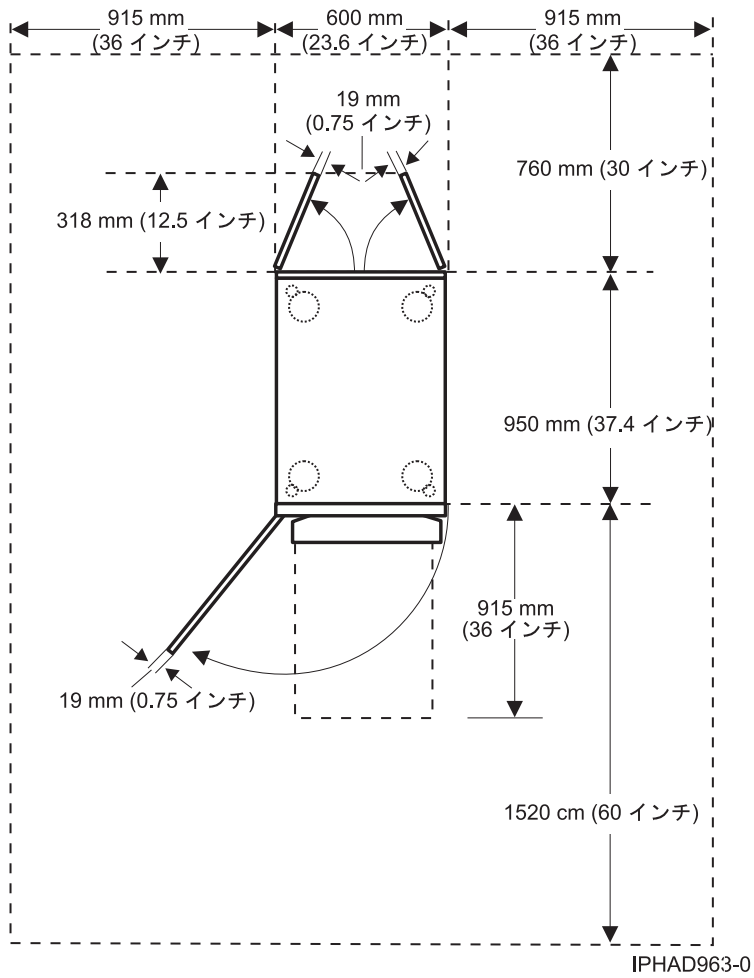
図 19. モデル 0555 および 7014-S25 平面図
