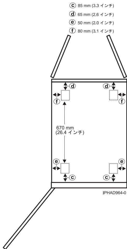
図 20. モデル 0555 および 7014-S25 のキャスト位置
