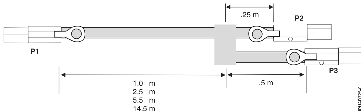
図 54. SAS 外付け Y0 ケーブル・アセンブリのケーブルの長さ
