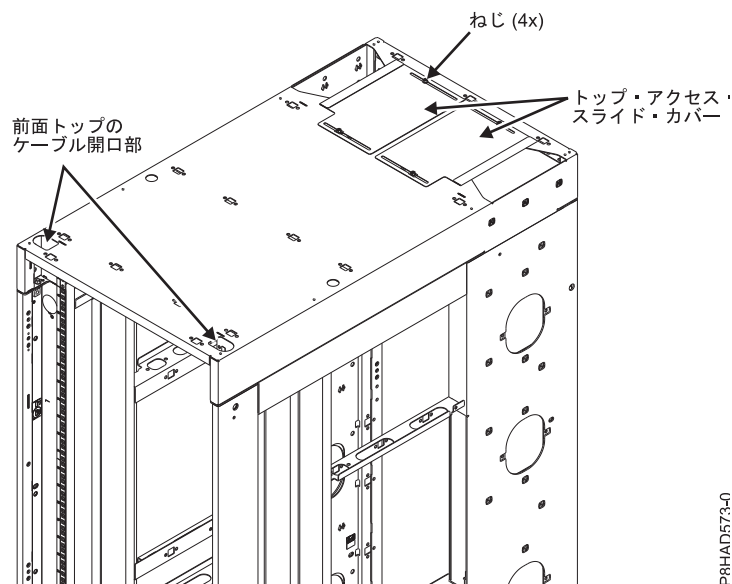
図 51. 上部でのケーブル接続
