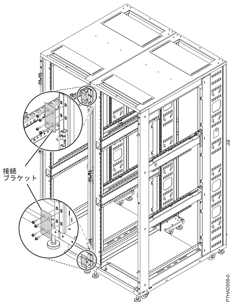
図 36. 接続ブラケット
