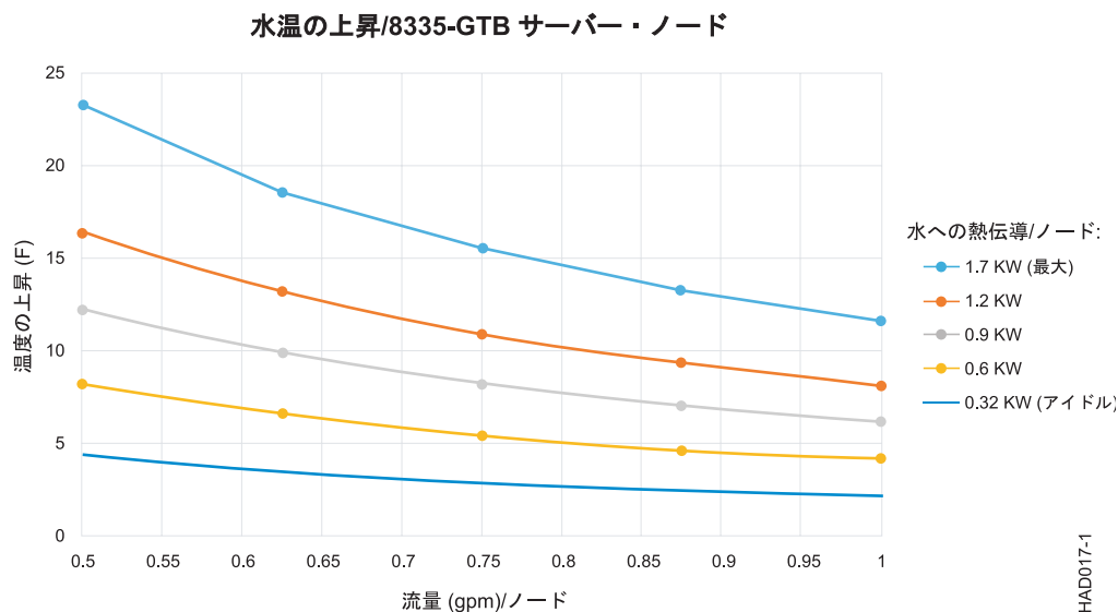
図 4. 水流量対給水温度 (標準法) - 単一サーバー
