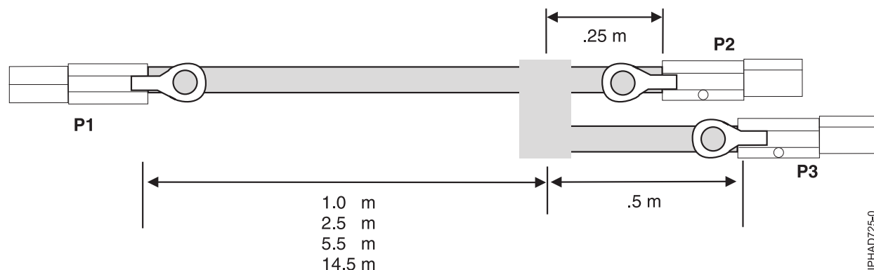
図 67. SAS 外付け YO ケーブル・アセンブリーのケーブルの長さ
