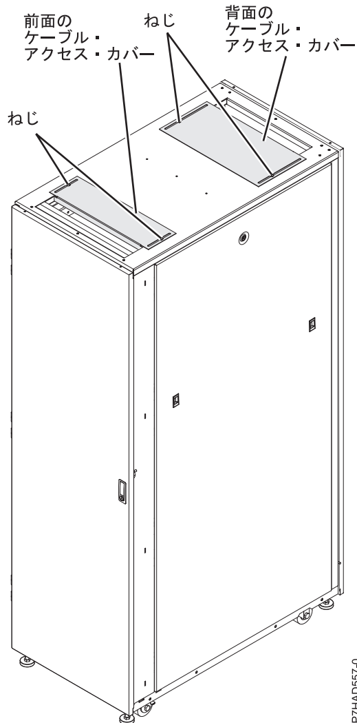
図 34. ケーブル・アクセス・カバー
