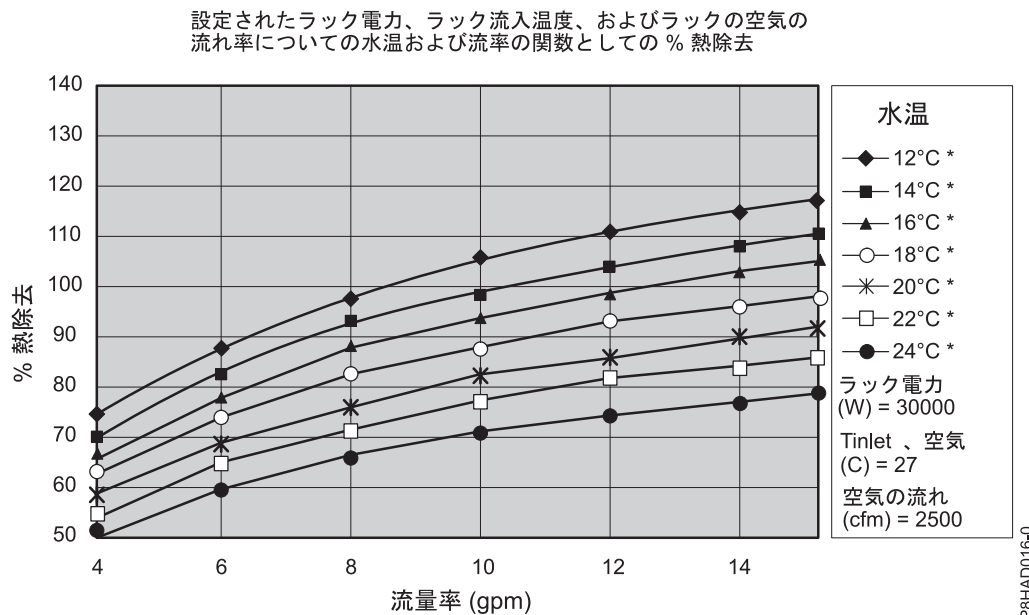
図 54. 熱負荷 30 kW のヒート・エクスチェンジャーの標準的な効率
