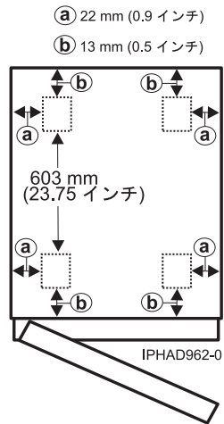
図 22. モデル 0554 および 7014-S11 のキャスター位置
