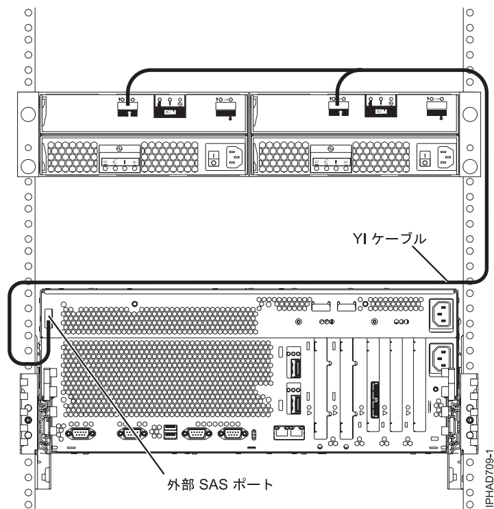
図 75. システム外部 SAS アダプター・ポートとディスク拡張ドロワー間
