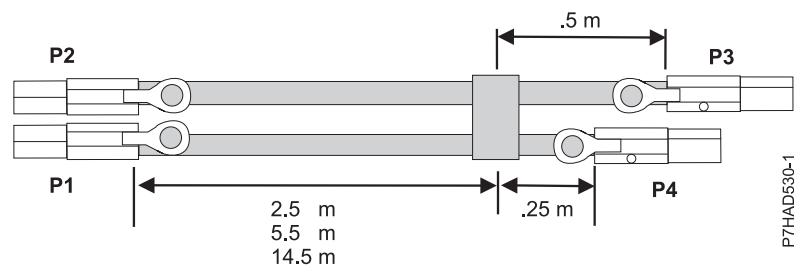
図 66. SAS 外付け X ケーブル・アセンブリのケーブルの長さ
