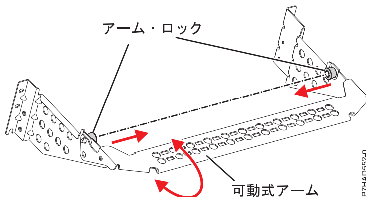
図 65. ケーブル管理ブラケット
