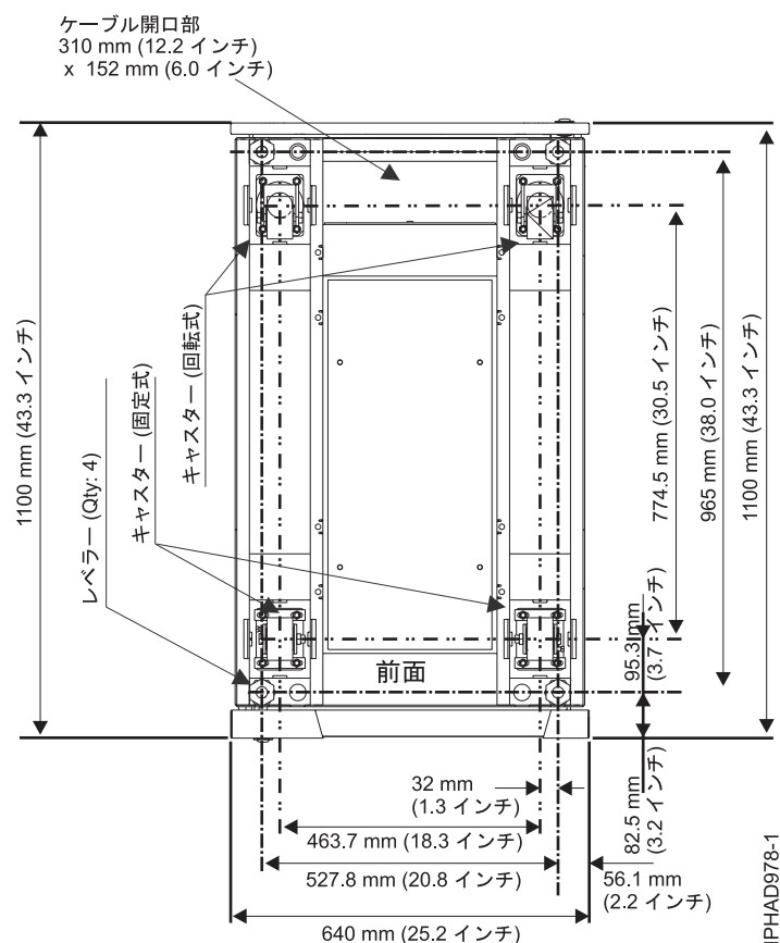
図 9. キャスターおよびレベラーの位置
