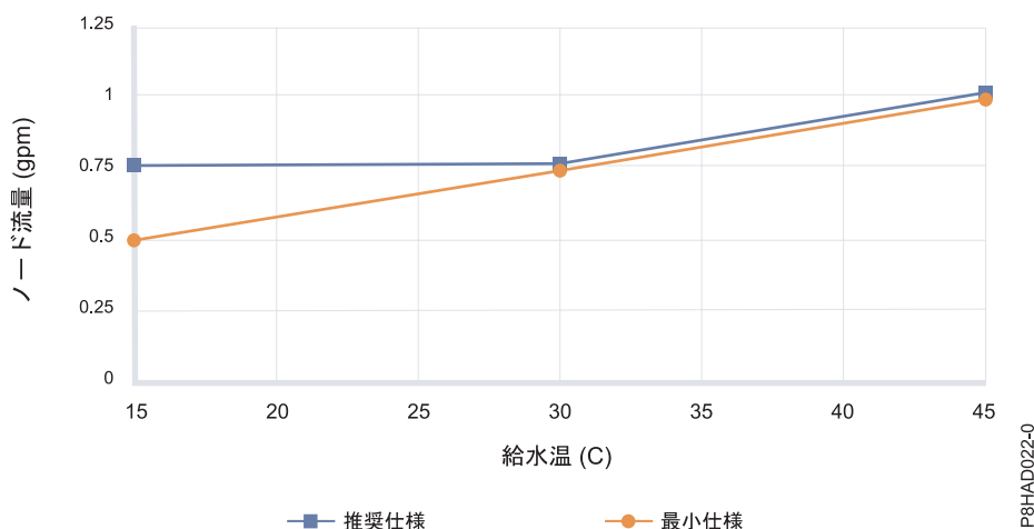
図 2. 水冷却水流量対給水の要件 (標準単位)
