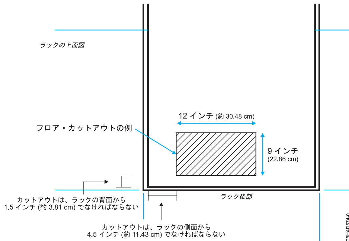
図 48. フロア・カットアウト
