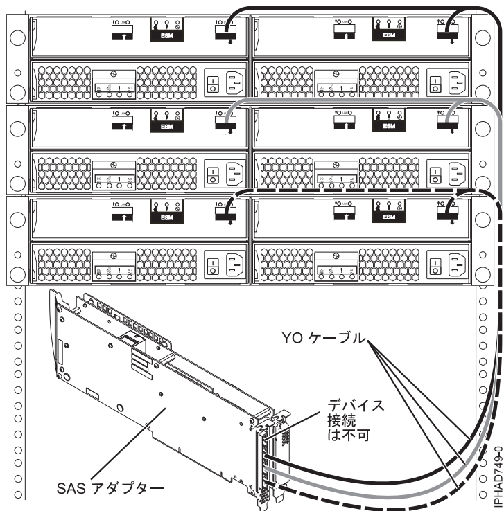
図 72. トライ・ポート SAS アダプターとディスク拡張ドロワー間
