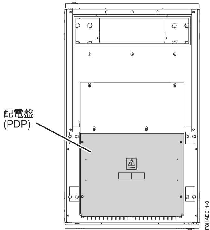
図 27. FC EPB8 - 配電盤 (上から見た図)
