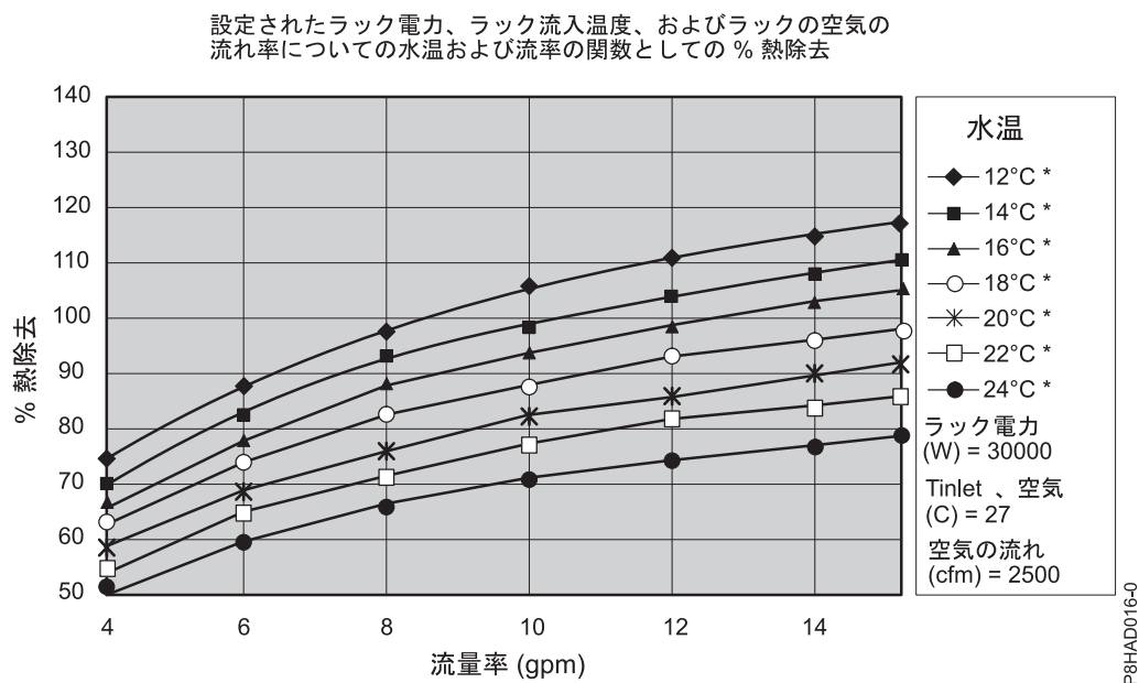
図 38. 熱負荷 30 kW のヒート・エクスチェンジャーの標準的な効率
