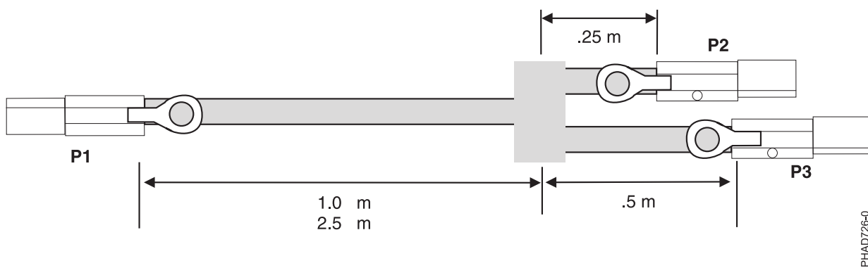
図 68. SAS 外付け YI ケーブル・アセンブリーのケーブルの長さ
