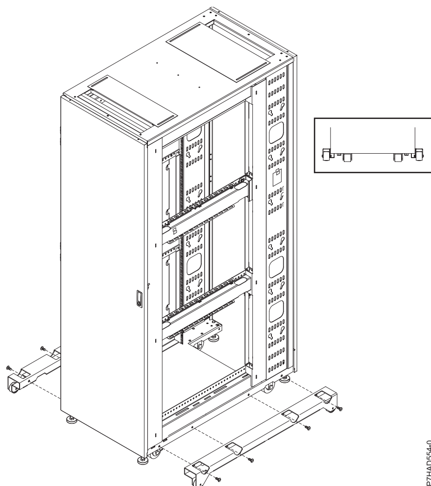
図 35. アウトリガーの位置
