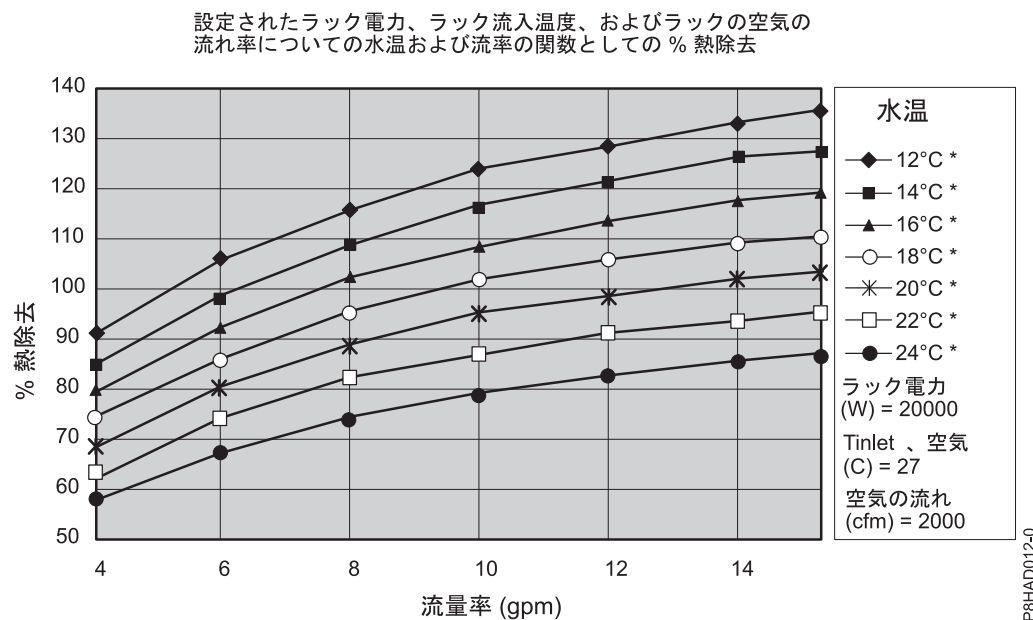
図 37. 熱負荷 20 kW のヒート・エクスチェンジャーの標準的な効率
