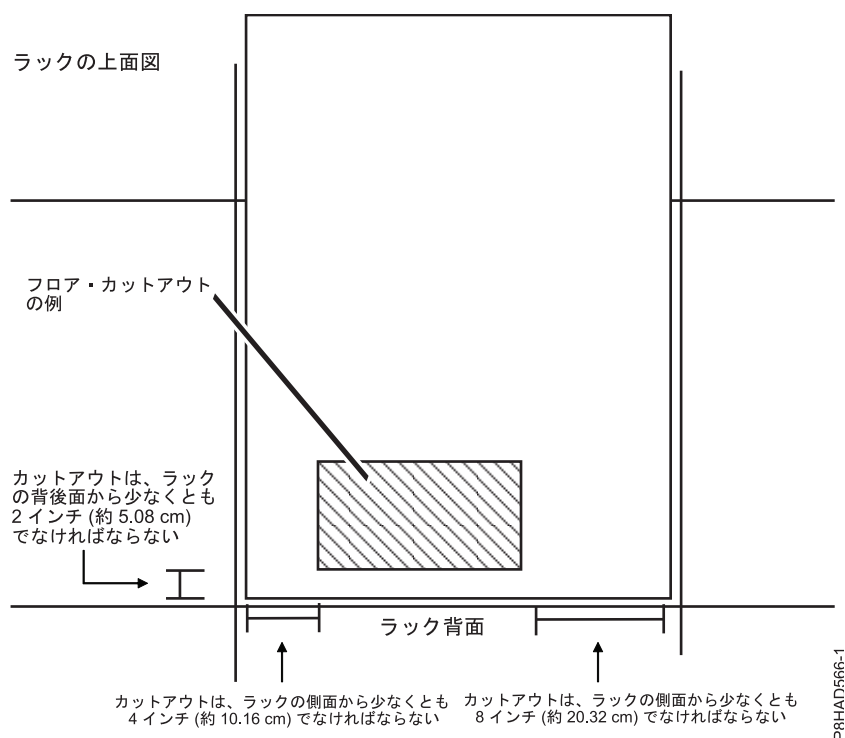
図 47. フロア・カットアウト
