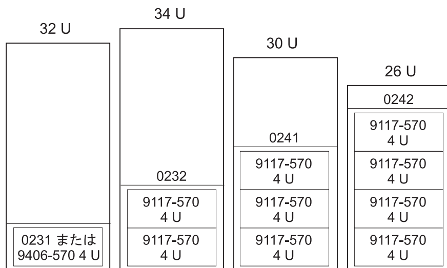
図 12. 570 のラック搭載
