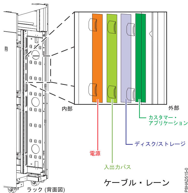
図 63. ケーブル管理ブリッジのレーン
