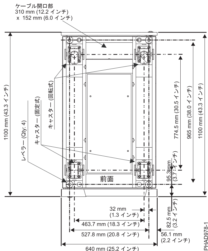
図 28. キャスターおよびレベラーの位置
