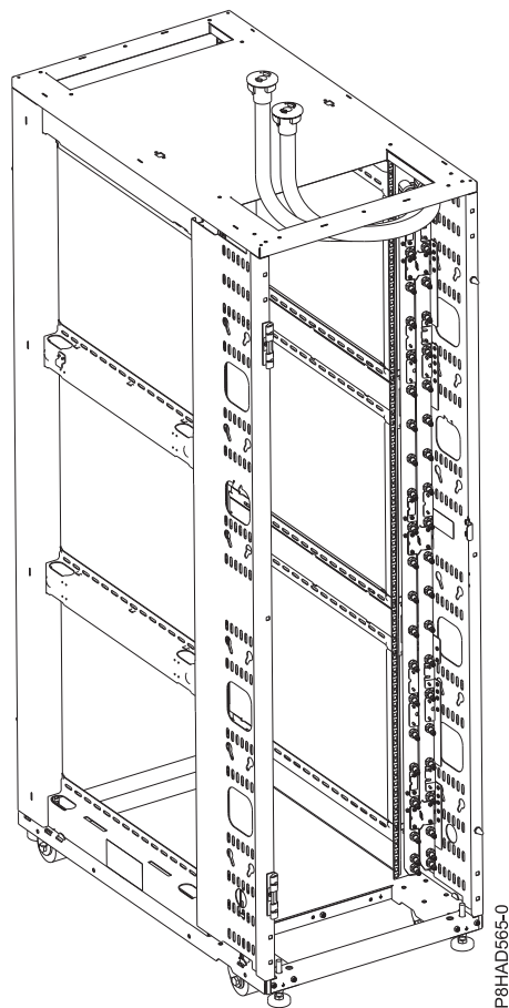
図 40. ラック、および供給ホースと返送ホースがラックの上部から出る連結管
