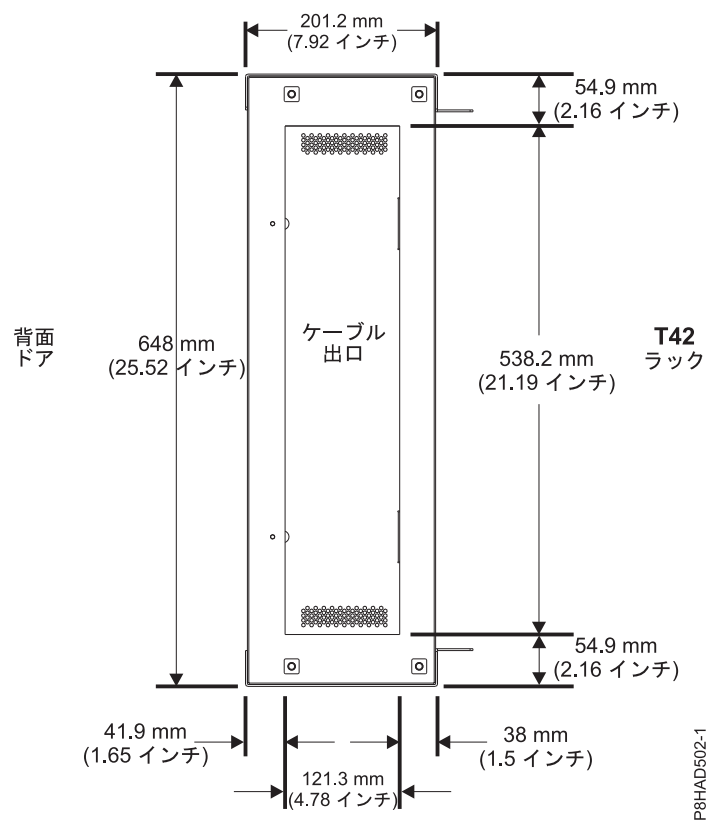
図 29. FC ERG0 背面ラック・エクステンダー (上から見た図)
