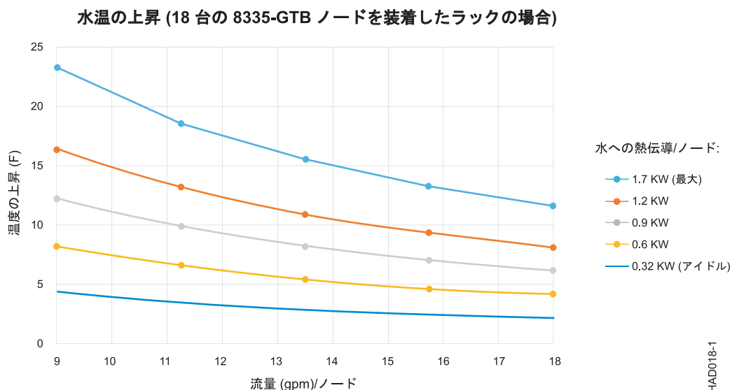
図 5. 水流量対給水温度 - フル・ラックの 18 台のサーバー
