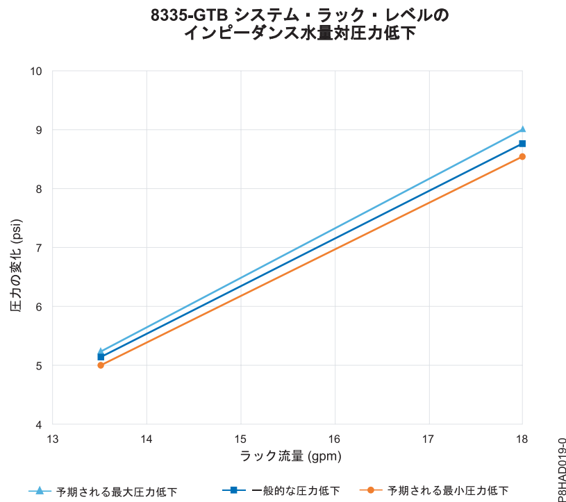
図 3. 流量対圧力低下 (標準法) - フル・ラックの 18 台のサーバー
