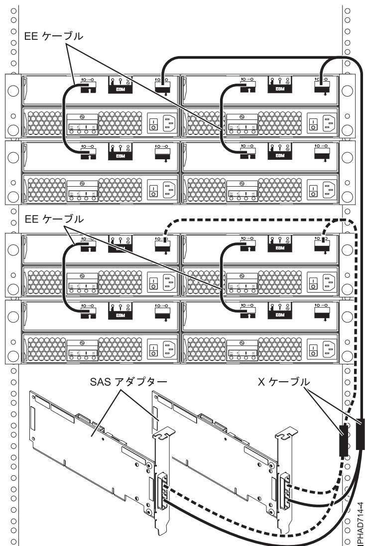
図 80. 2 つの SAS RAID アダプターと 4 つのディスク拡張ドロワー間 (マルチ・イニシエーター HA RAID 構成)
