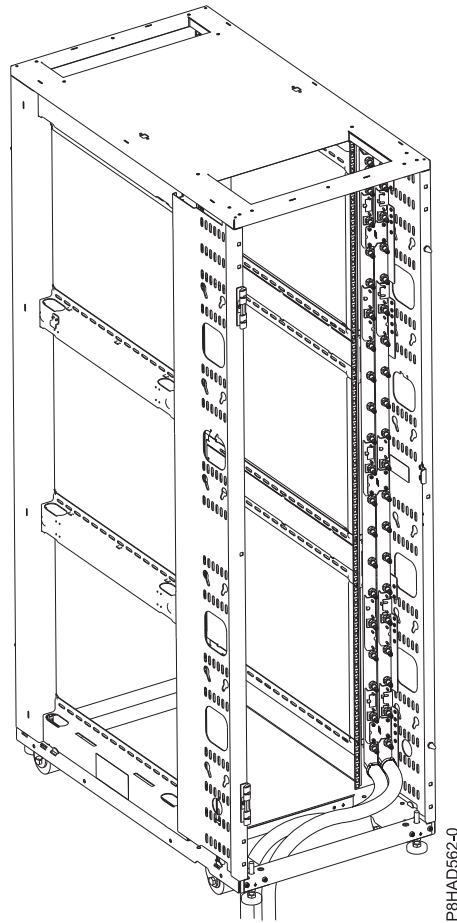
図 41. ラック、および供給ホースと返送ホースがラックの下部から出る連結管 上部ホース出口の位置
