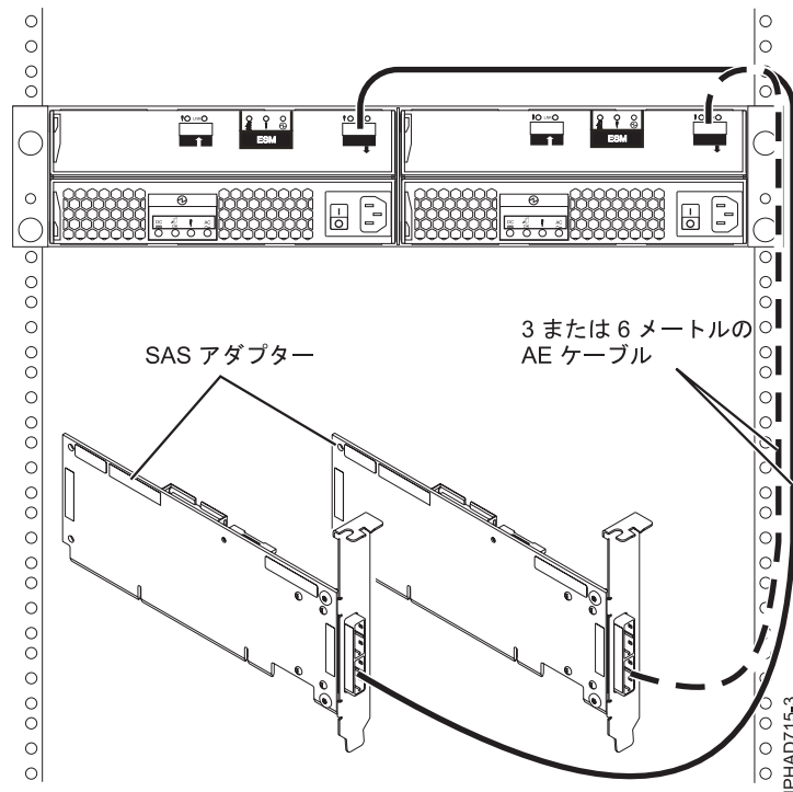
図 86. 2 つの RAID SAS アダプターと 1 つのディスク拡張ドロワー間 (マルチ・イニシエーター HA JBOD 構成)
