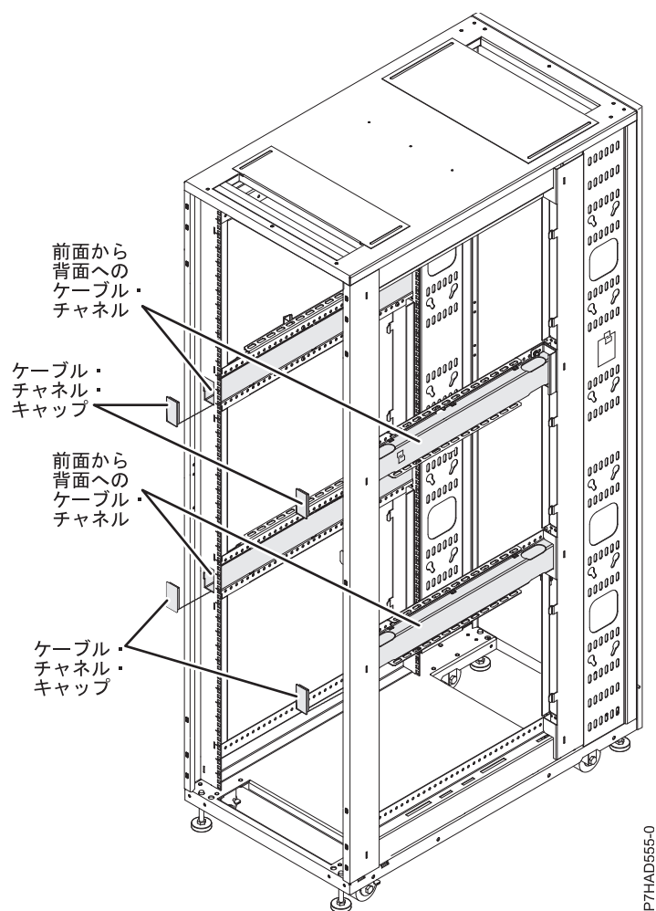
図 32. ラック内ケーブル接続
