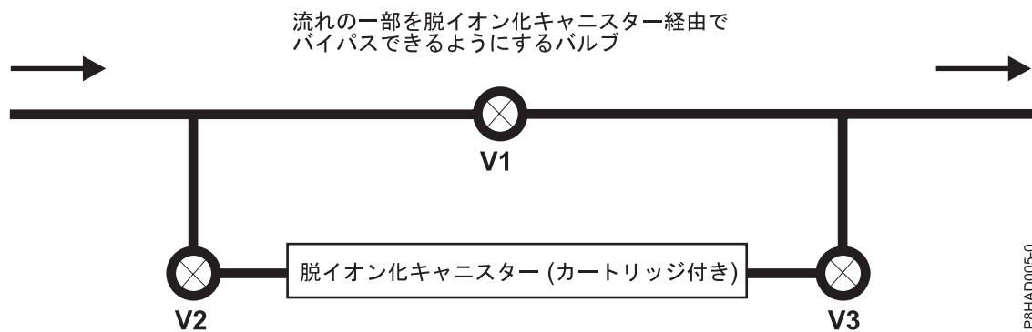
図 88. 冷却ループに取り付けられた脱イオン化カートリッジを使用した水の脱イオン化
