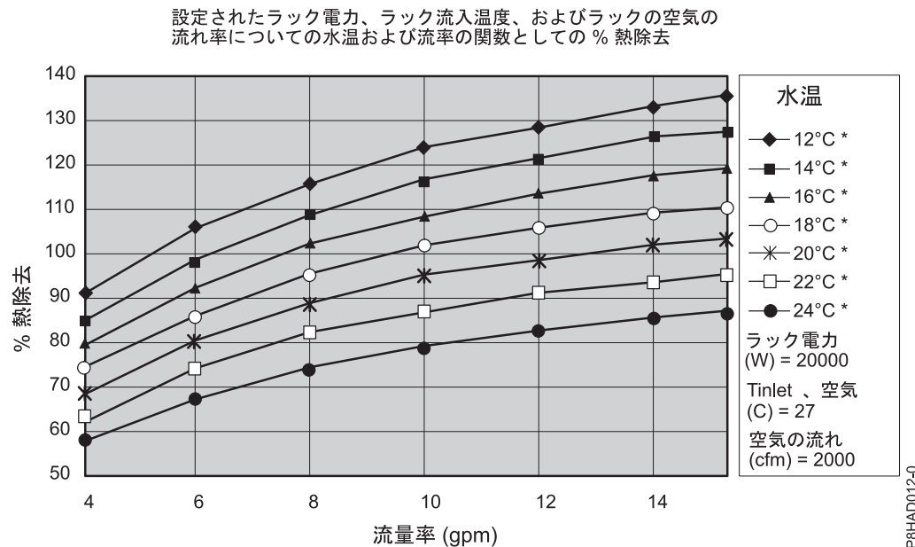
図 53. 熱負荷 20 kW のヒート・エクスチェンジャーの標準的な効率
