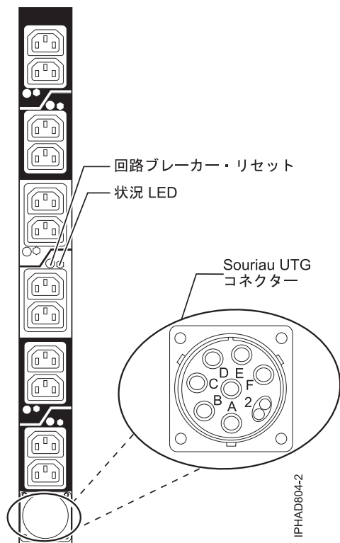
図 60. PDU コンセントの図
