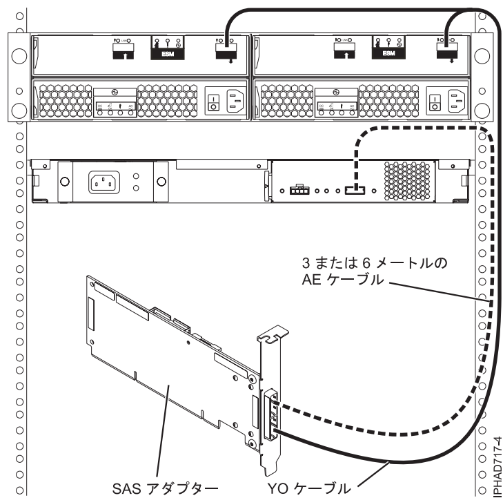
図 74. ディスク拡張ドロワーとメディア拡張ドロワーの両方と SAS アダプター間
