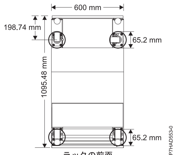
図 31. キャスターの位置
