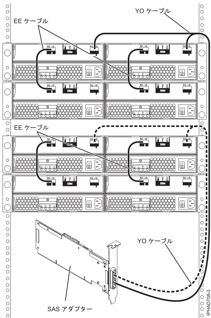
図 71. SAS アダプターと 4 つのディスク拡張ドロワー間
