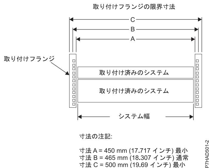
図 56. 取り付けフランジの限界寸法
