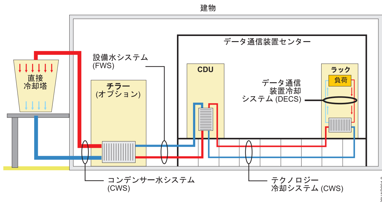
図 87. データ・センター内の液体冷却システムおよびループの例
