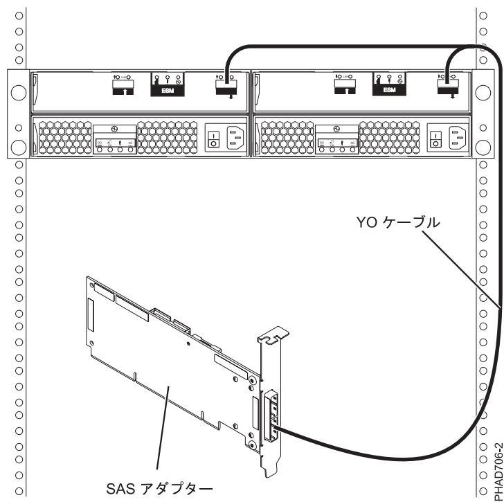
図 69. SAS アダプターとディスク拡張ドロワー間
