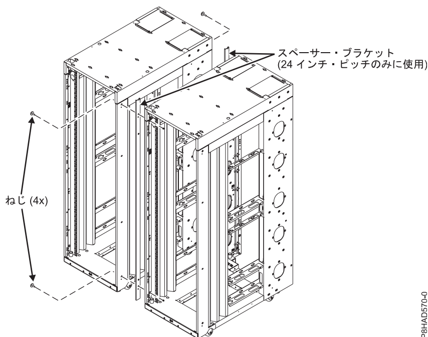
図 52. 複数のラックの接続
