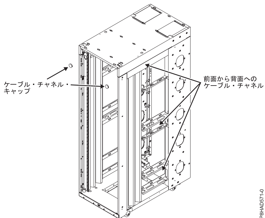
図 49. ラック内ケーブル接続
