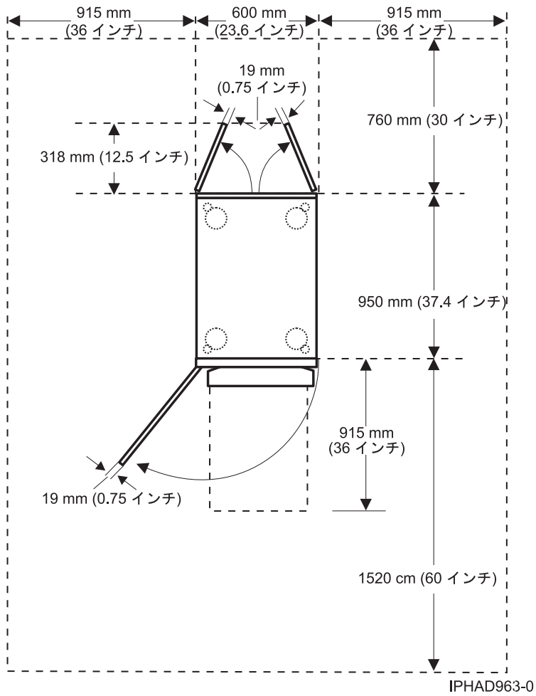
図 24. モデル 0555 および 7014-S25 平面図
