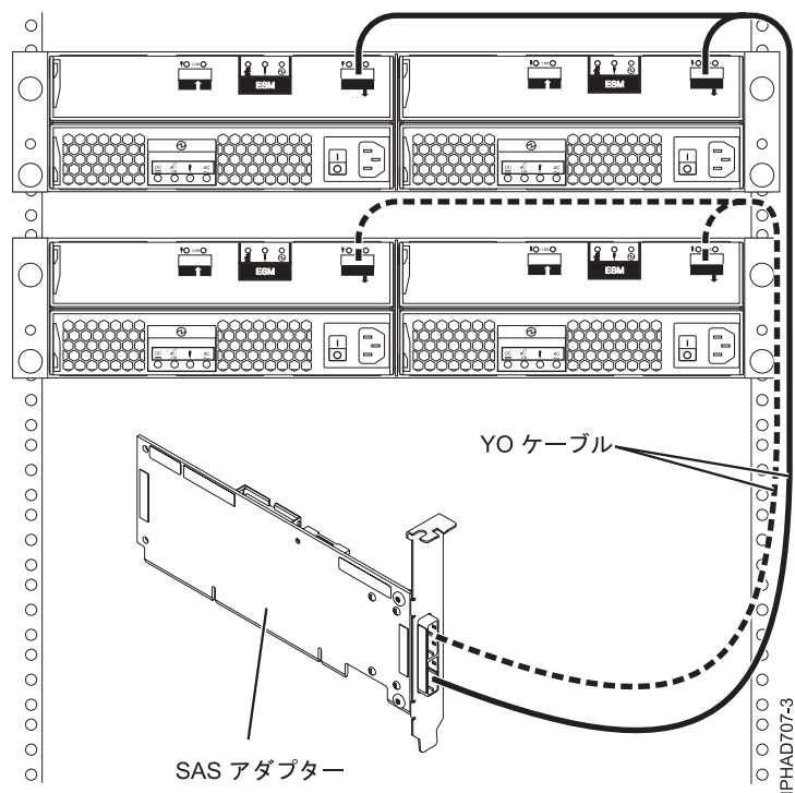
図 70. SAS アダプターと 2 つのディスク拡張ドロワー間
