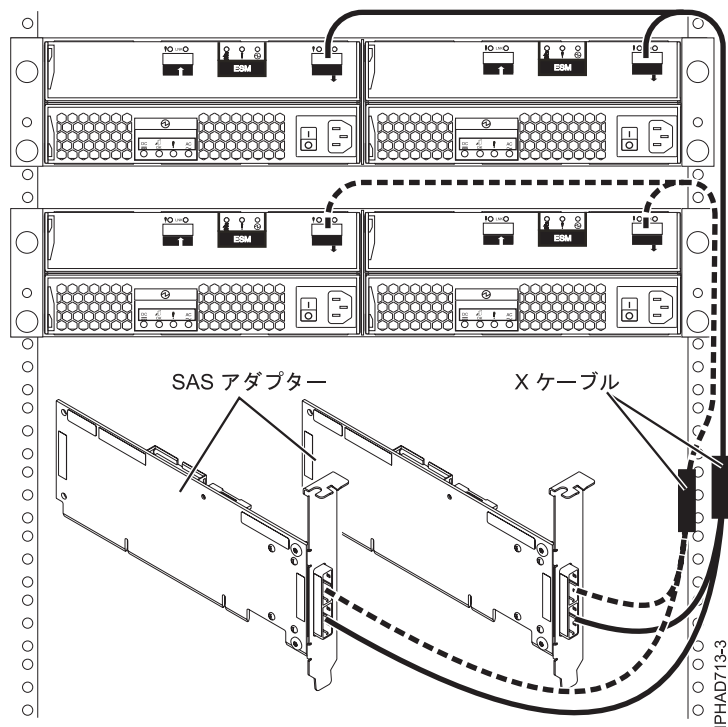
図 79. 2 つの SAS RAID アダプターと 2 つのディスク拡張ドロワー間 (マルチ・イニシエーター HA RAID 構成)
