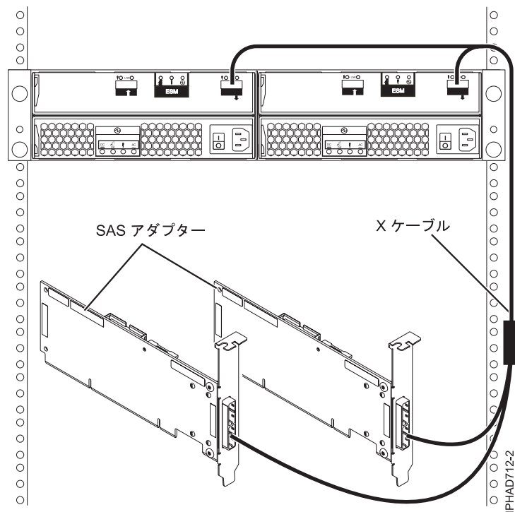
図 78. 2 つの SAS RAID アダプターと 1 つのディスク拡張ドロワー間 (マルチ・イニシエーター HA RAID 構成)
