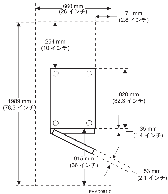
図 21. モデル 0554 および 7014-S11 平面図
