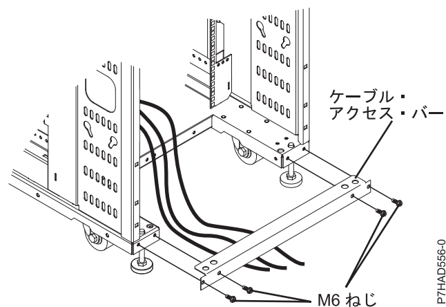
図 33. ケーブル・アクセス・バー
