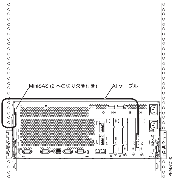
図 76. SAS アダプターと内部 SAS ディスク・スロット間 (システム外部 SAS ポートを使用)
