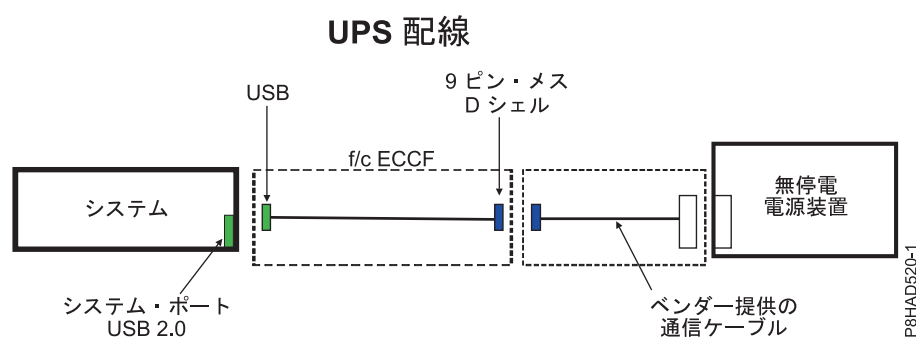
図 58. 5148-21L、5148-22L、8247-21L、8247-21L、8247-22L、8247-42L、8284-22A、8286-41A、および 8286-42A の UPS 配線
