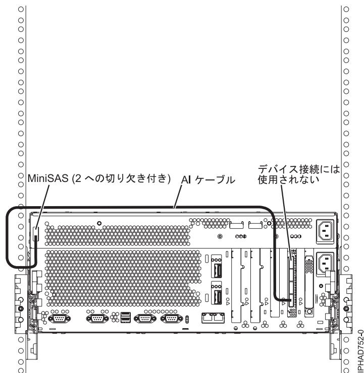
図 77. ディスク拡張ドロワーに接続された FC5904 または FC5908 アダプター
