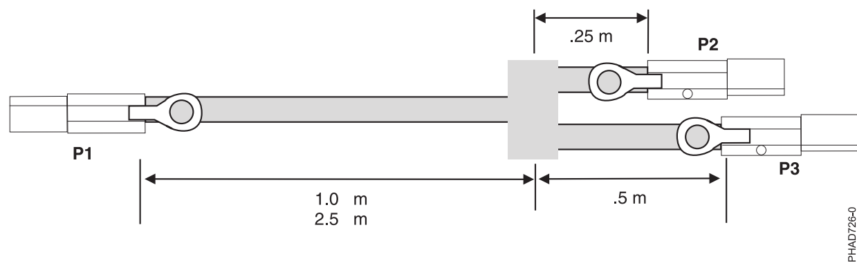
図 55. SAS 外付け Y1 ケーブル・アセンブリのケーブルの長さ
