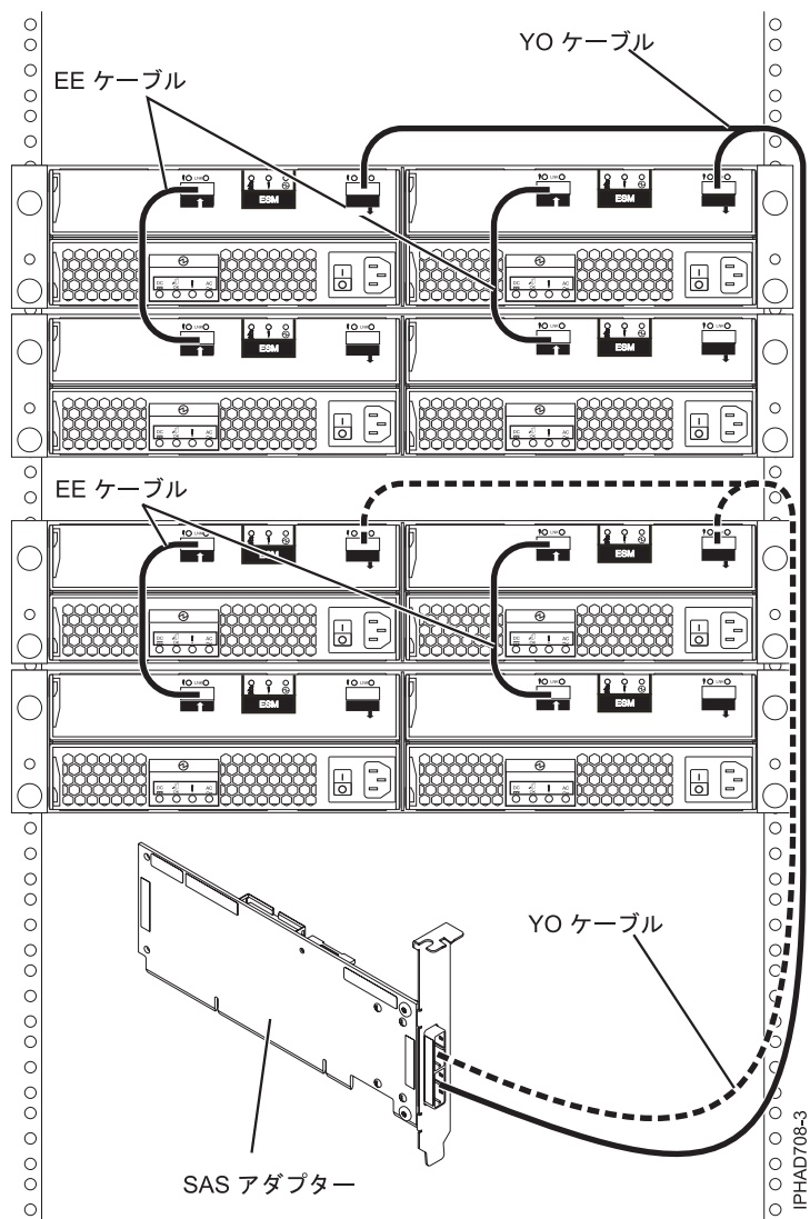
図 58. SAS アダプターと 4 つのディスク拡張ドロー間
