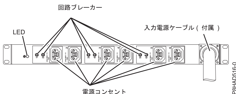
図 49. HVDC PDU
