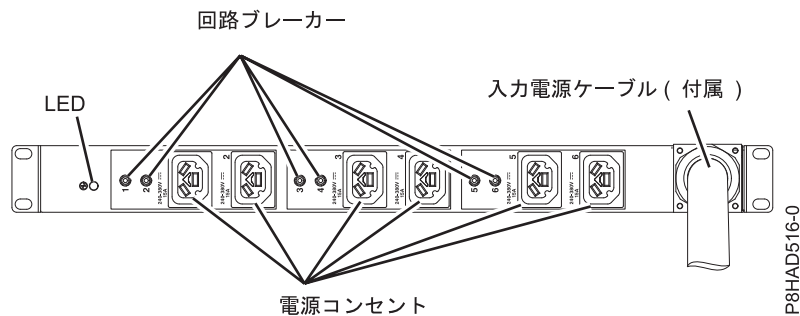
図 49. HVDC PDU
