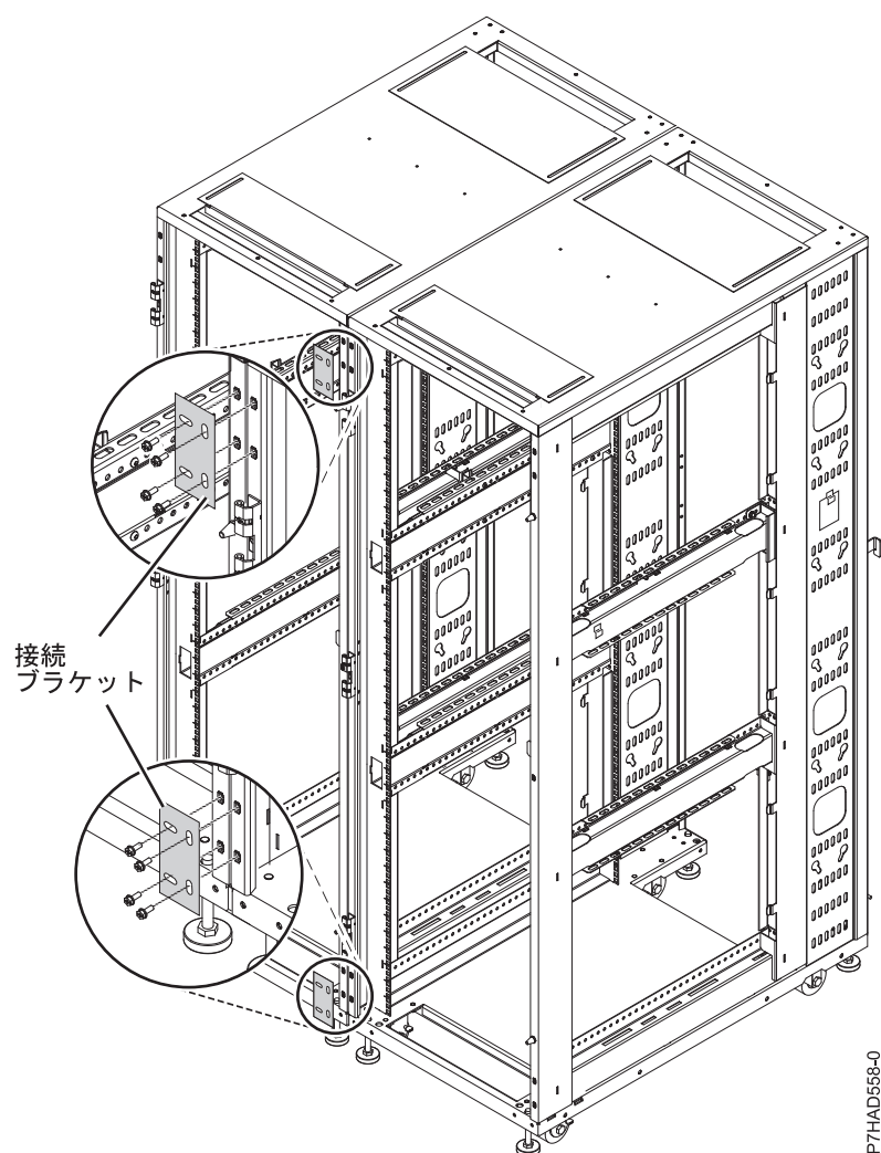
図 31. 接続ブラケット
