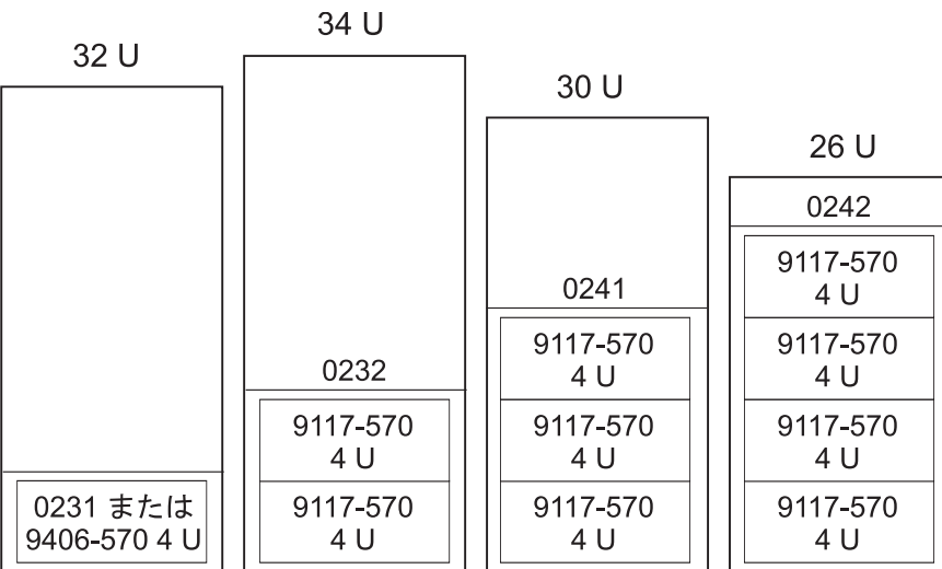
図 7. 570 のラック搭載
