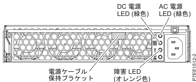
図 4. 電源装置の背面図
