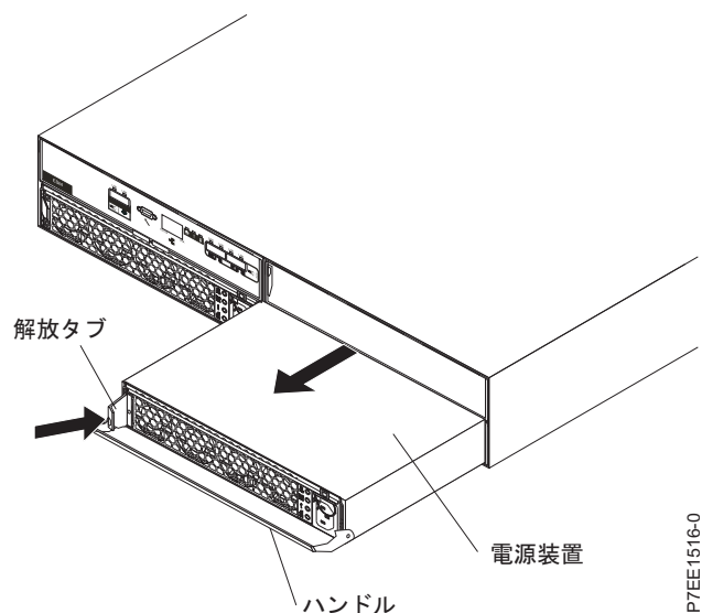
図 5. 電源装置の取り外し
