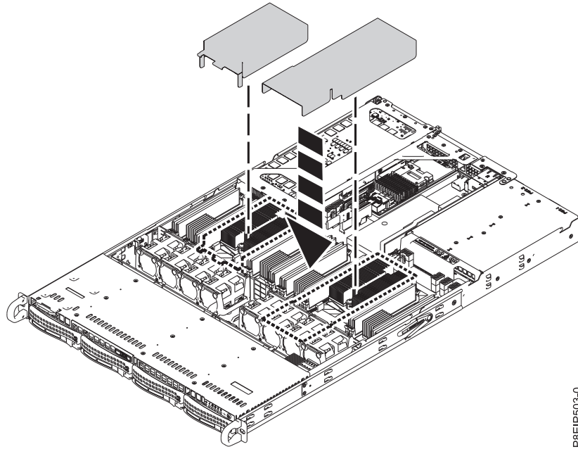
図 61. プロセッサ・エア・バックルの取り付け
