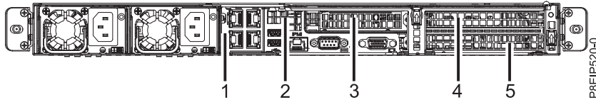
図 88. 8001-12C PCIe アダプターの位置
