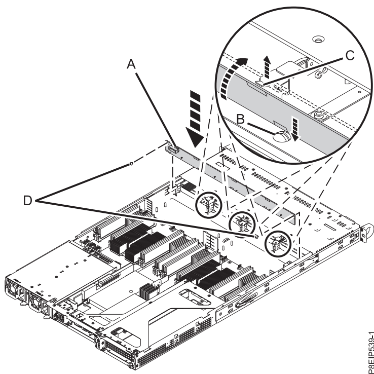
図 14. ディスク・ドライブ・バックプレーン の取り付け
