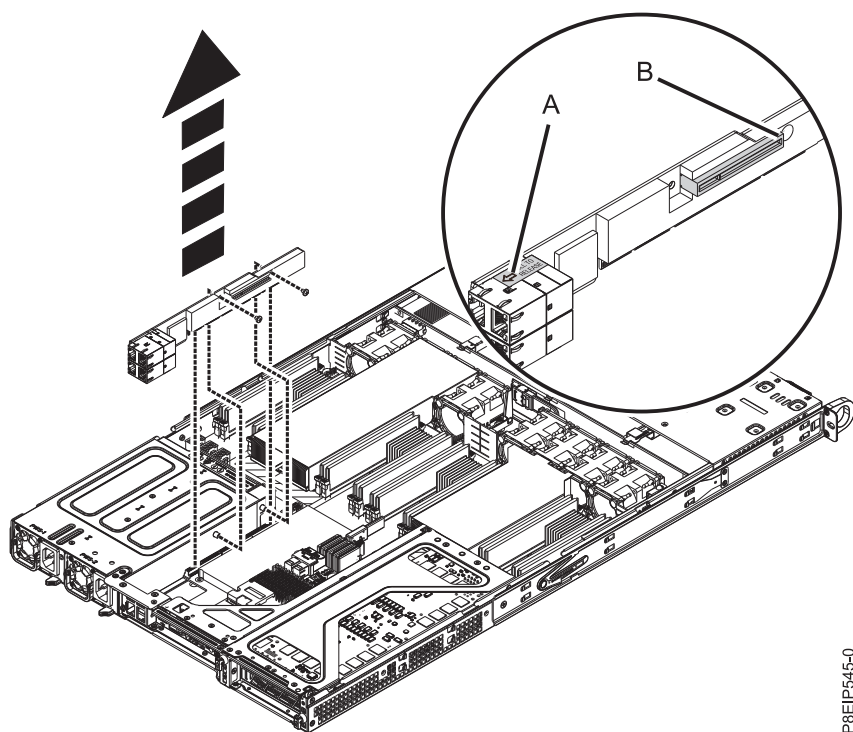
図 33. PCIe ライザーのねじの取り外し
