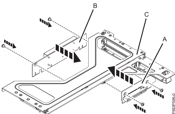
図 41. アダプター・ケージへの PCIe ライザー・カードの再取り付け
