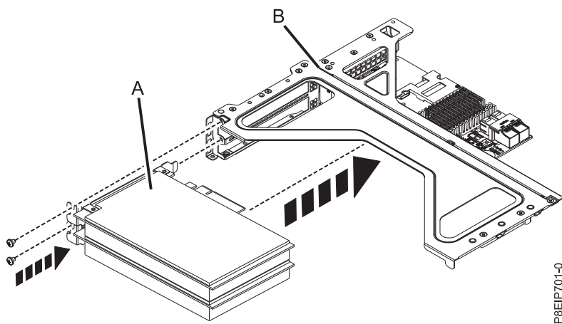
図 43. ライザーの位置 4 または位置 5 へのアダプターの挿入
