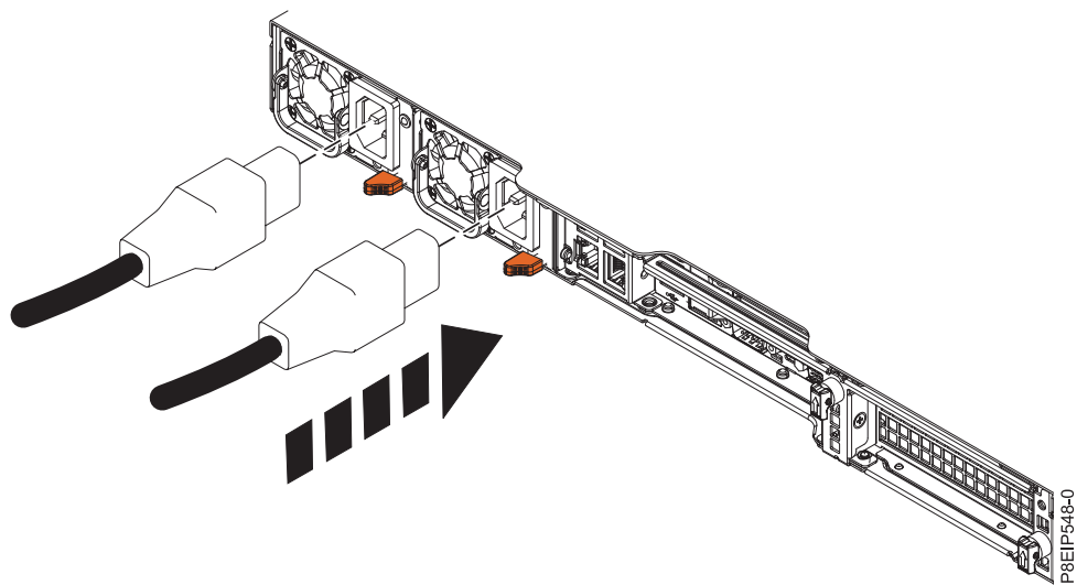
図 87. システムへの電源コードの接続
