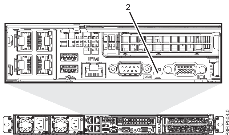
図 77. システムの背面の LED
