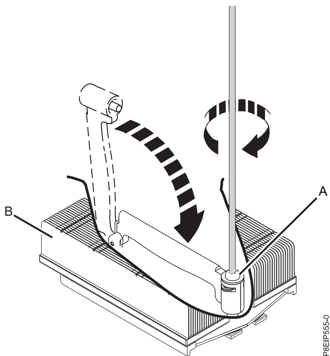
図 72. ロード・アームのねじを締める
