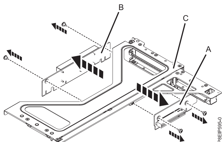
図 38. アダプター・ケージからの PCIe ライザー・カードの取り外し
