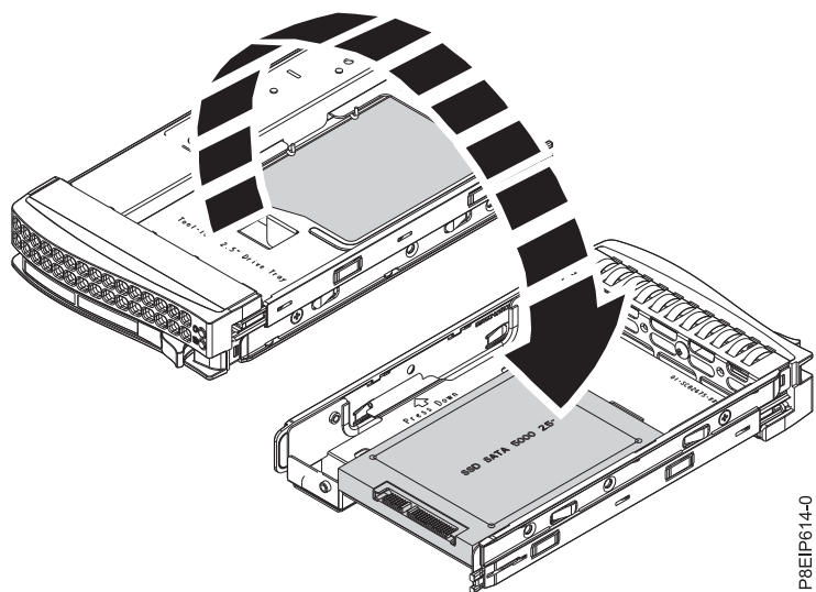
図 3. 2.5 型トレイを裏返しにする
