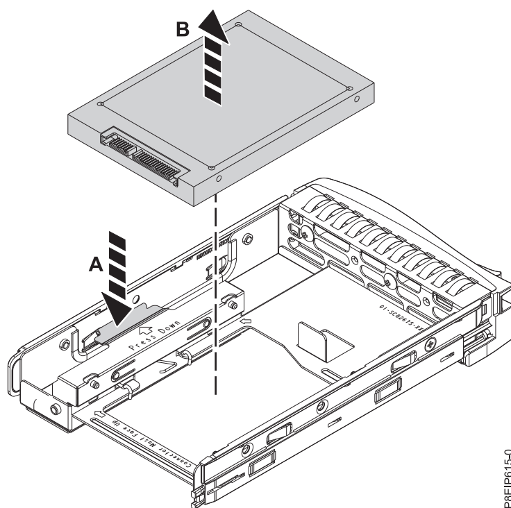
図 4. トレイからの 2.5 型ドライブの取り外し
