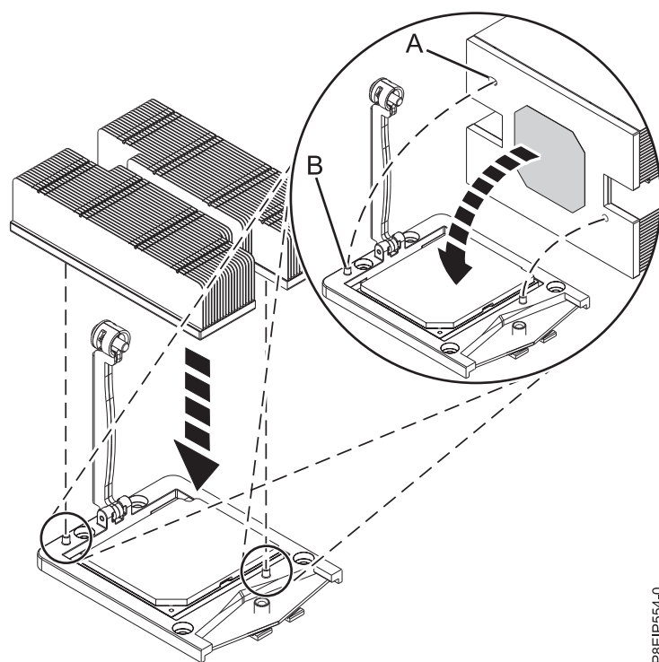
図 71. ヒート・シンクの取り付け
