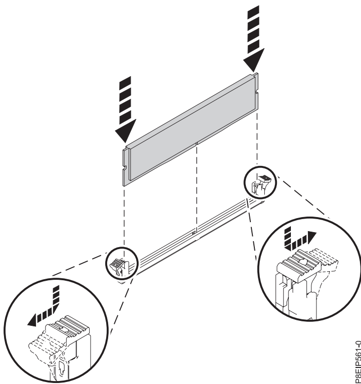
図 30. メモリー DIMM の挿入
