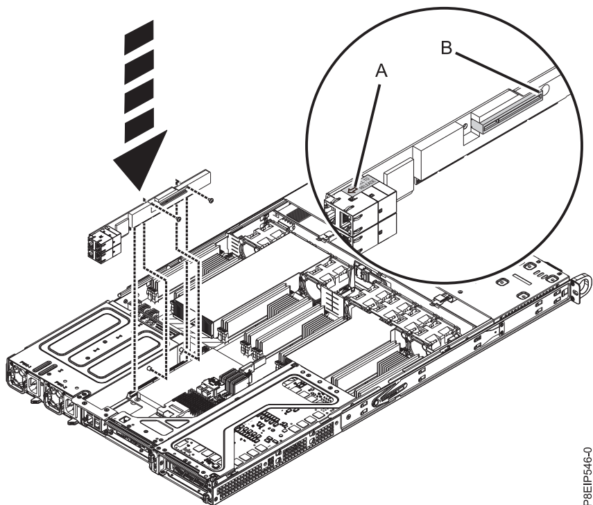
図 40. PCIe ライザーのねじの再取り付け
