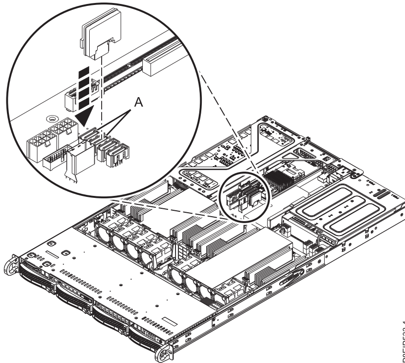
図 10. DOM の取り付け
