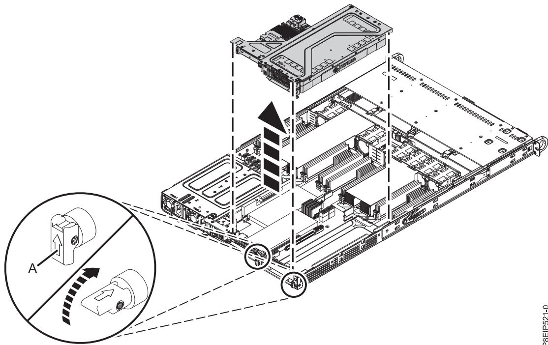
図 34. PCIe ライザーの取り外し
