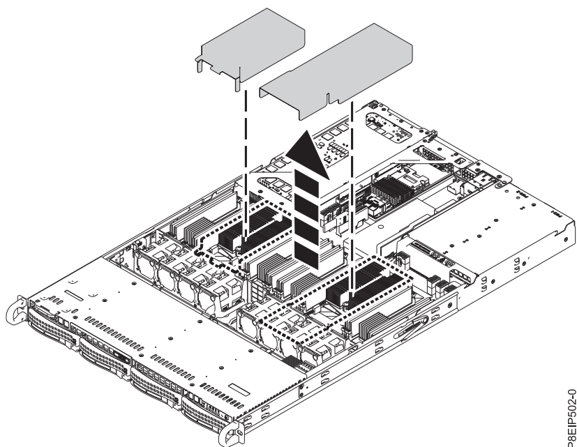
図 28. プロセッサ・エア・バッフルの取り外し
