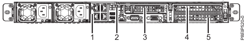
図 39. 8001-12C PCIe アダプターの位置
