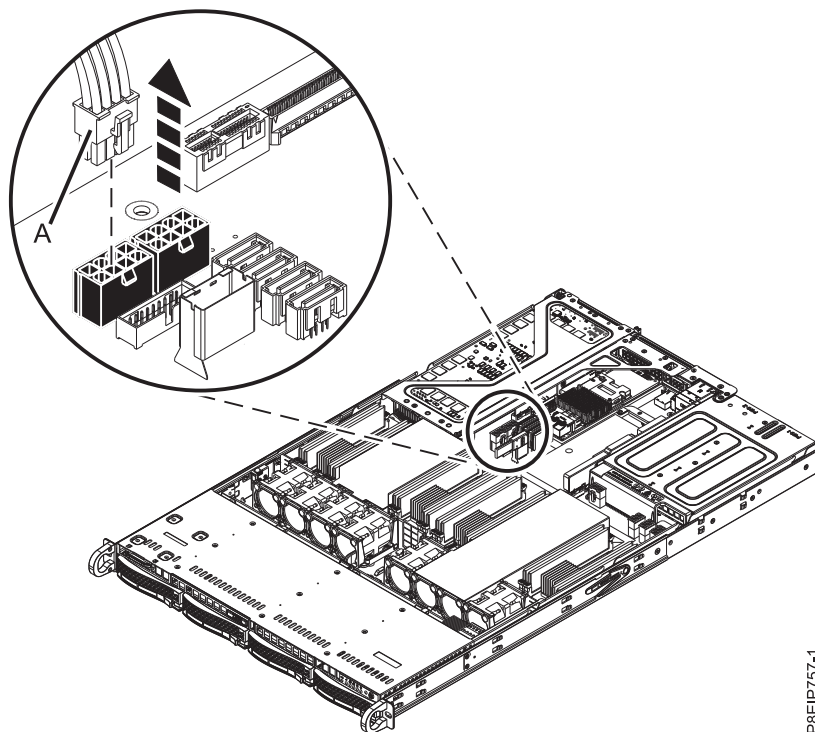
図 22. GPU 電源ケーブルのプラグを抜く
