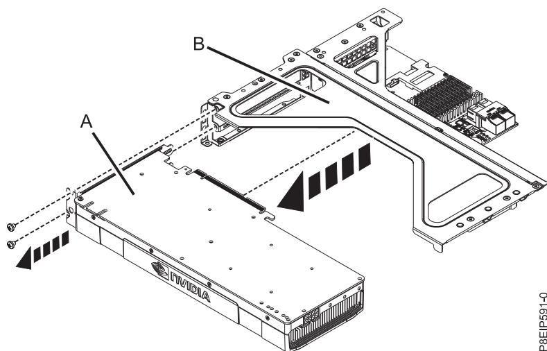
図 24. ライザーからの GPU の取り外し
