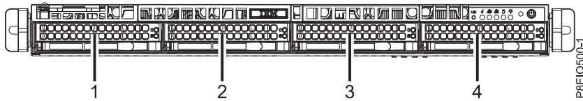
図 89. NVMe ドライブの位置
