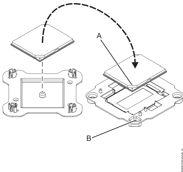
図 74. 配送用トレイへのシステム・プロセッサ・モジュールの取り付け
