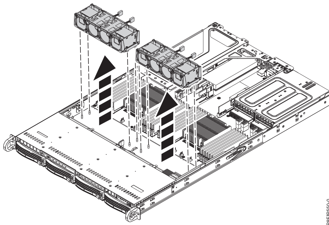
図 16. ファン・ホルダーの取り外し
