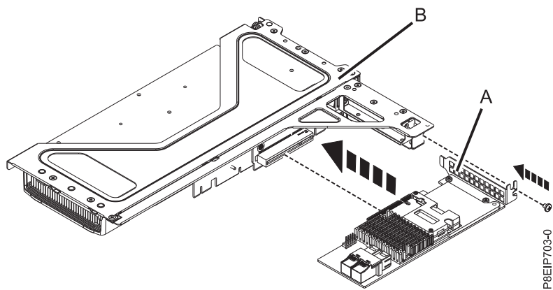
図 42. ライザーの位置 3 へのアダプターの挿入
