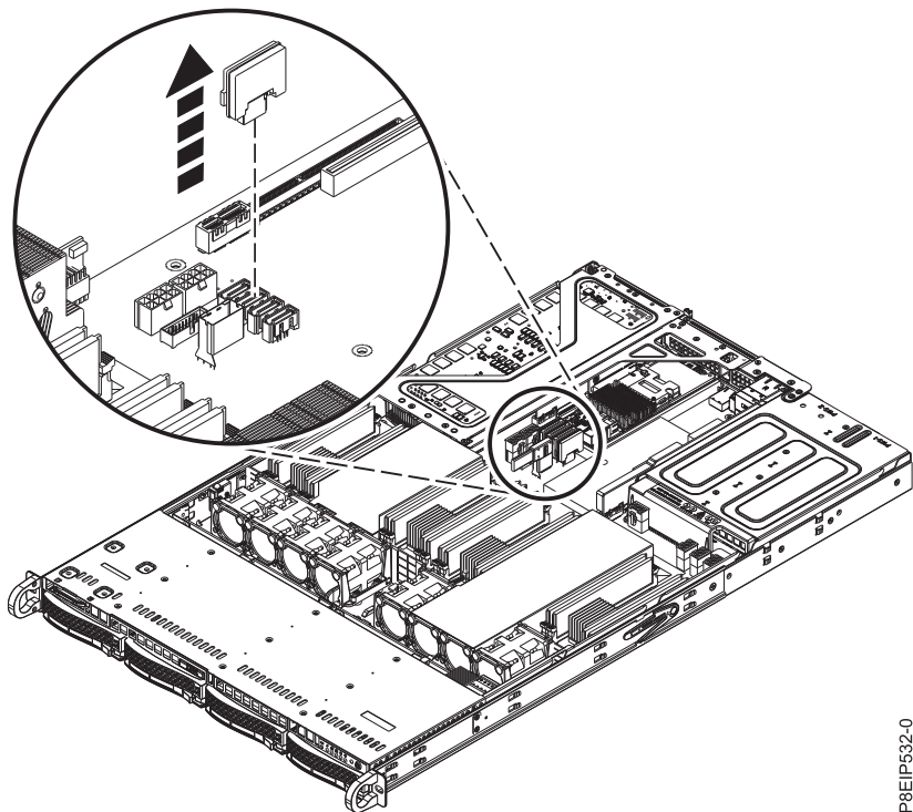
図 9. DOM の取り外し
