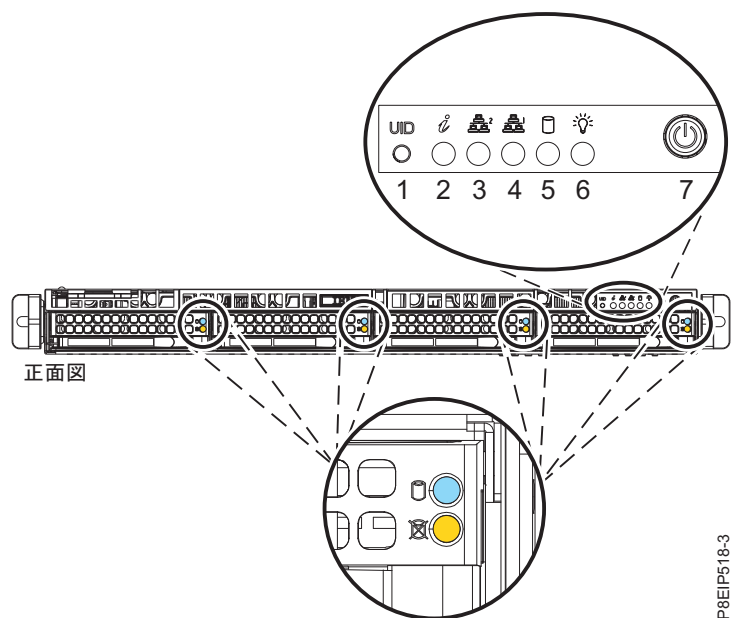
図 76. システムの前面の LED
