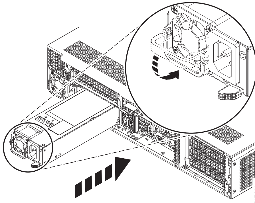
図 81. システムの電源装置の取り替え
