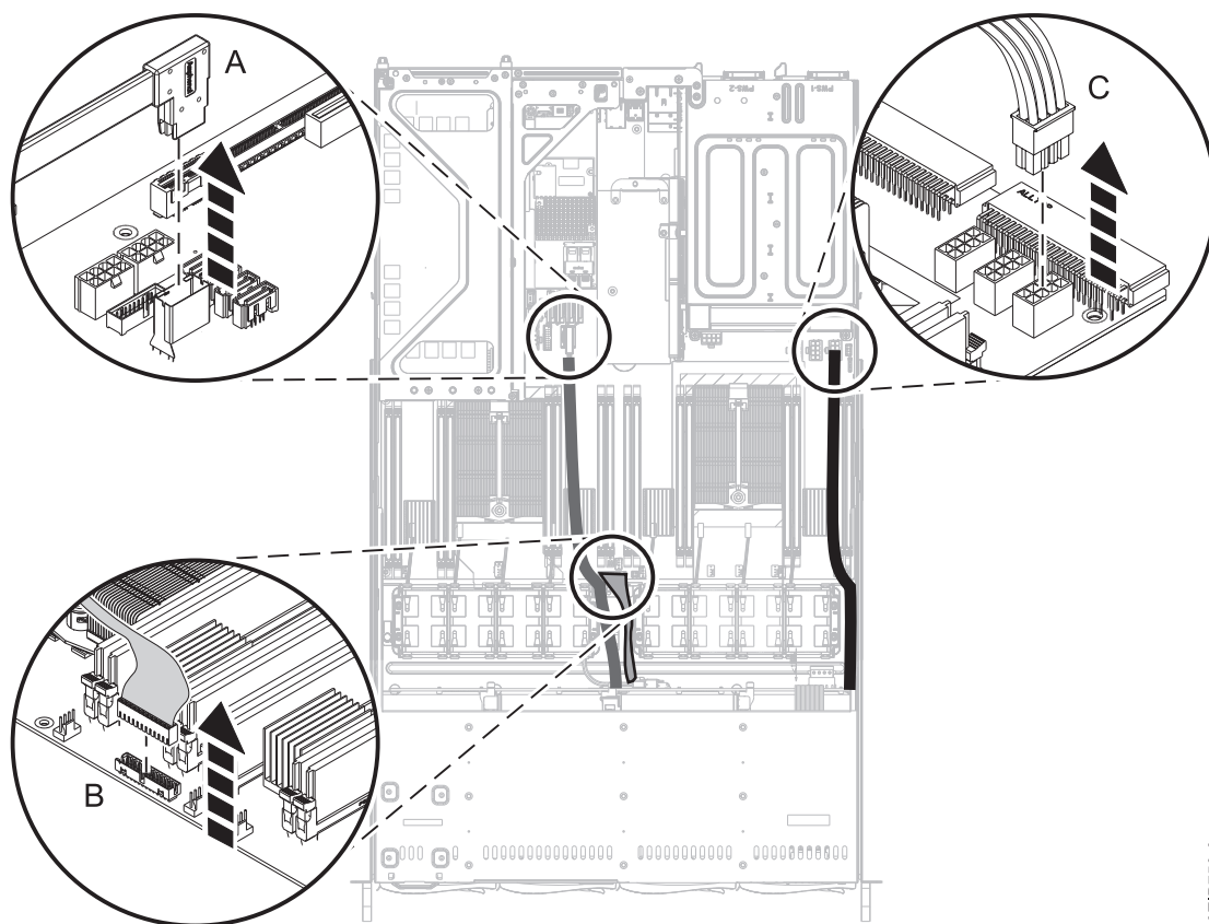
図 11. ドライブの信号ケーブルと電源ケーブルの切り離し
