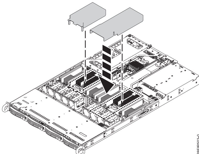
図 31. プロセッサ・エア・バッフルの取り付け
