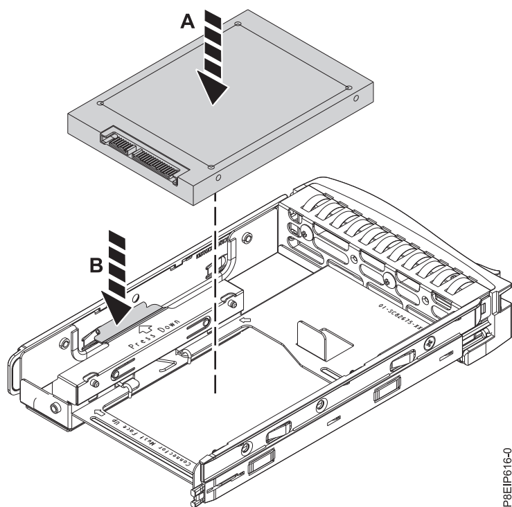
図 7. トレイへの 2.5 型ドライブの取り付け
