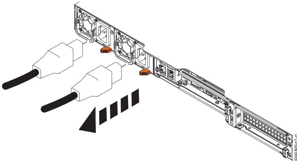
図 86. システムからの電源コードの取り外し
