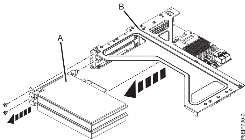
図 37. ライザーの位置 4 または位置 5 からの PCIe アダプターの取り外し
