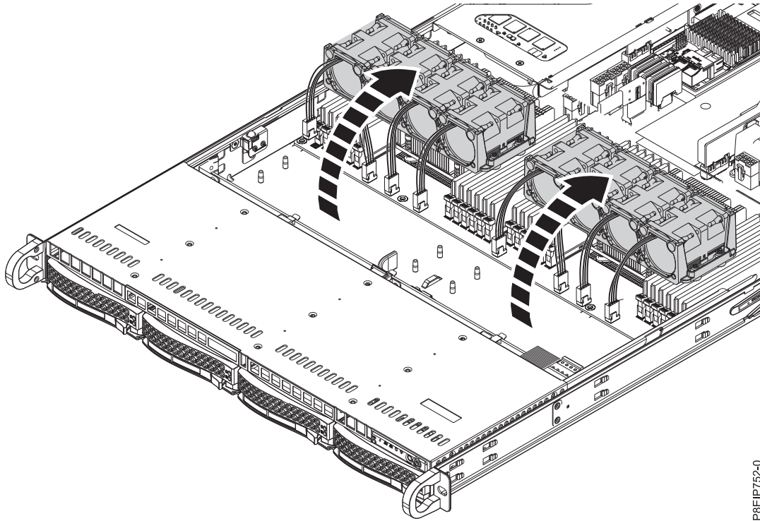
図 12. ファンの移動
