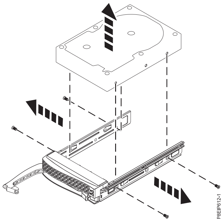
図 2. トレイからの 3.5 型ドライブの取り外し
