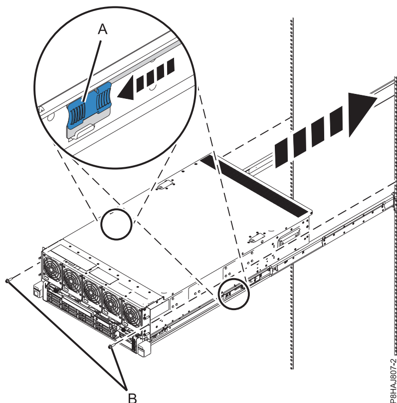
図 25. システムの操作位置への設置
