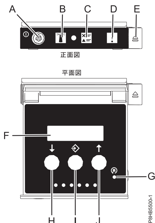
図 14. コントロール・パネルの LED
