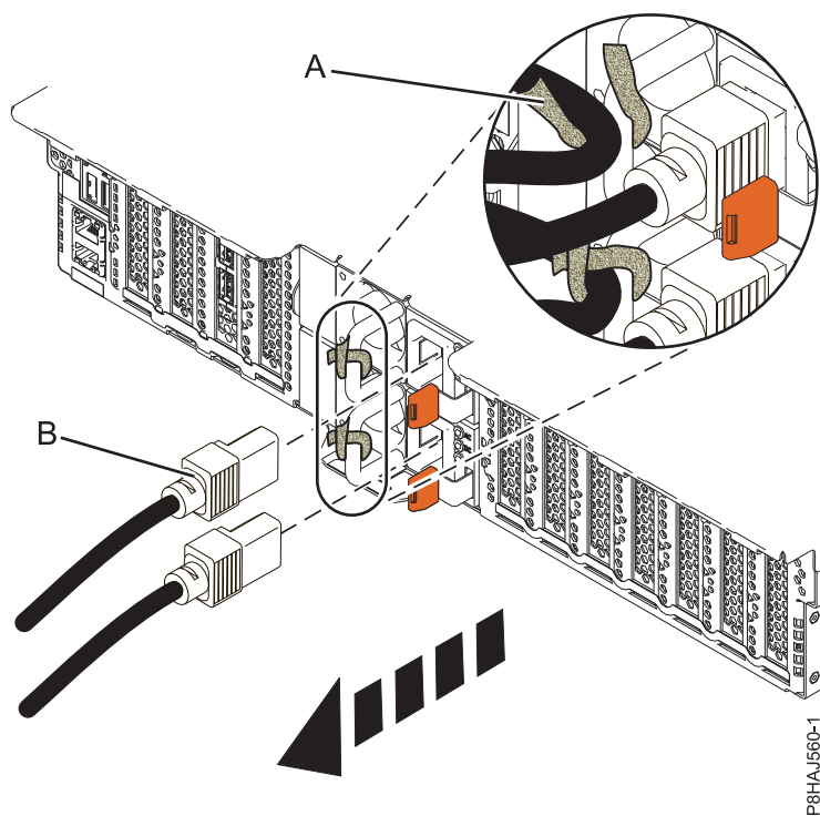
図 28. 8247-21L、8247-22L、または 8284-22A システムからの電源コードの取り外し
