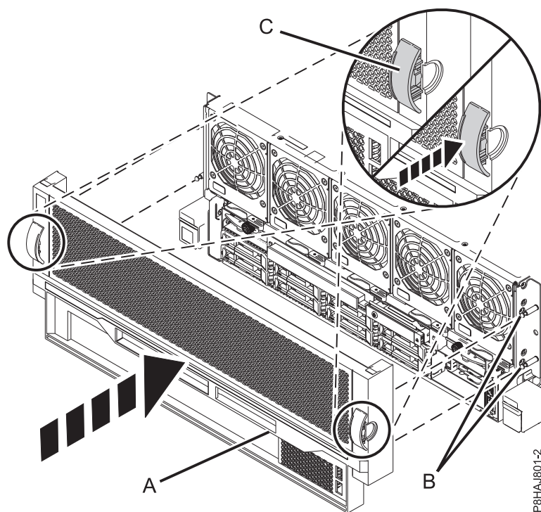
図 17. 前面カバーの取り付け
