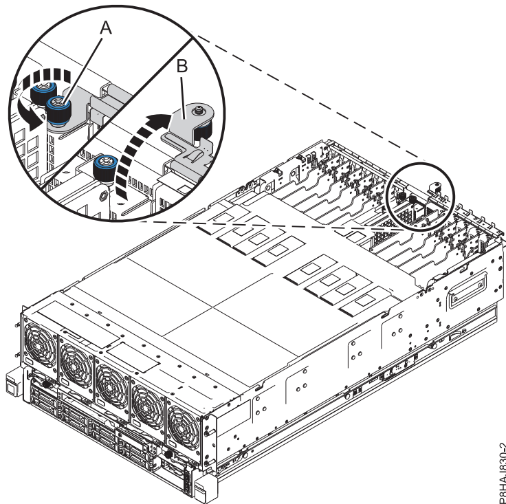
図 22. 入出力ラッチのオープン
