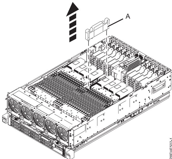
図4. システムからのプロセッサ電圧調節モジュール・フィルターの取り外し
