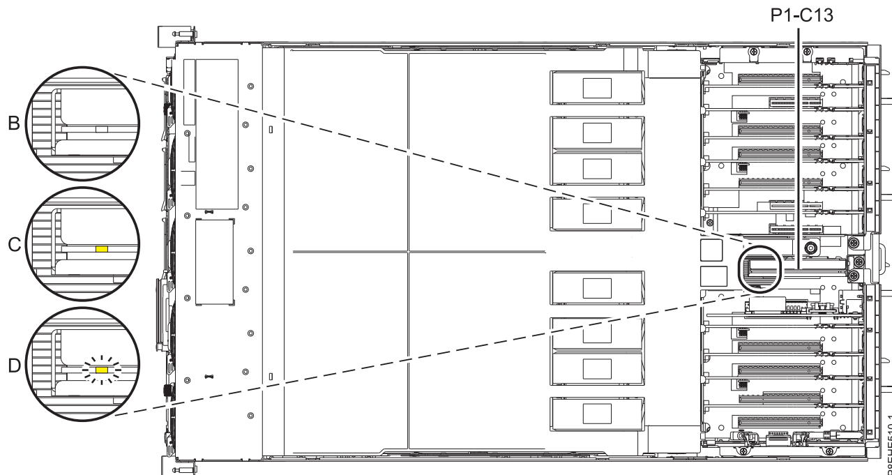
図 6. 8408-E8Eシステムでの入出力電圧調節モジュールおよび LED の位置
