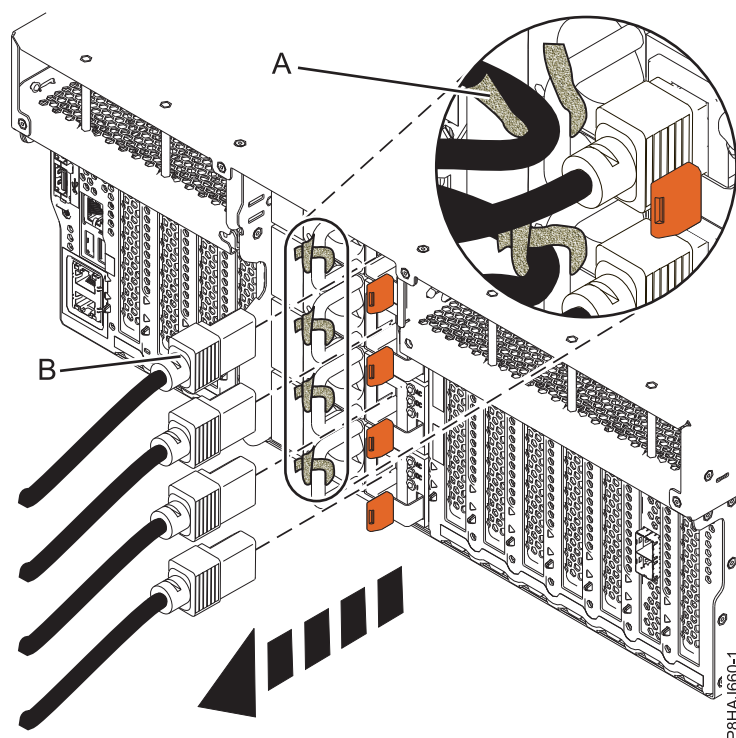
図 27. 8247-42L、8286-41A、または 8286-42A システムからの電源コードの取り外し
