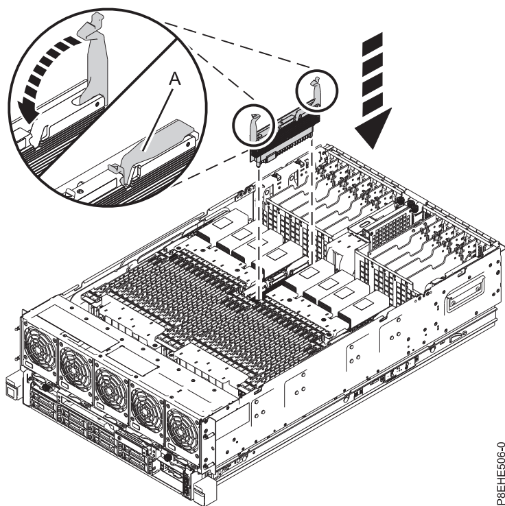
図 13. システムへのプロセッサ電圧調節モジュールの再取り付け
