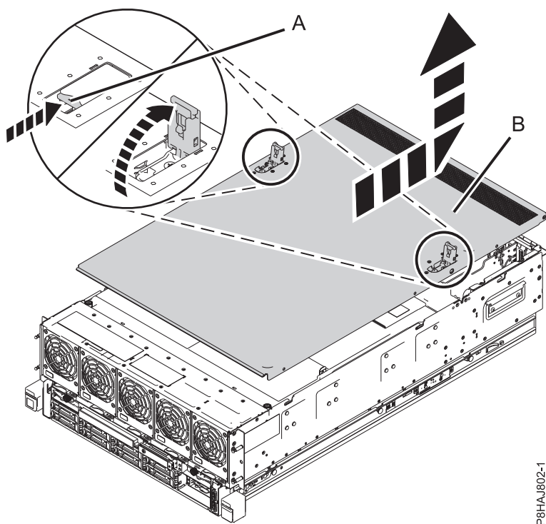
図 18. 保守アクセス・カバーの取り外し
