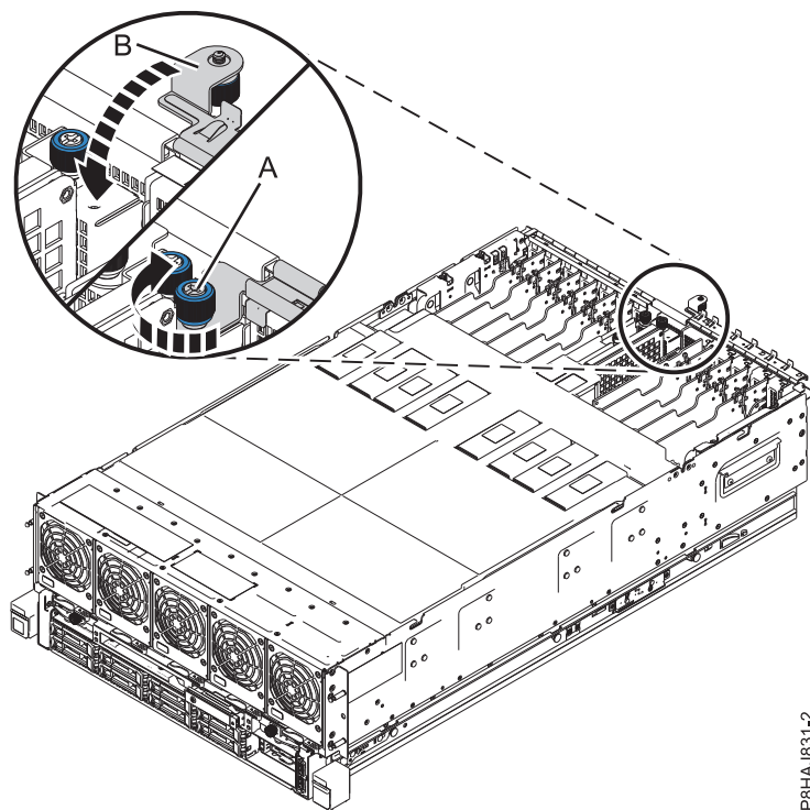
図 23. 入出力ラッチのクローズ
