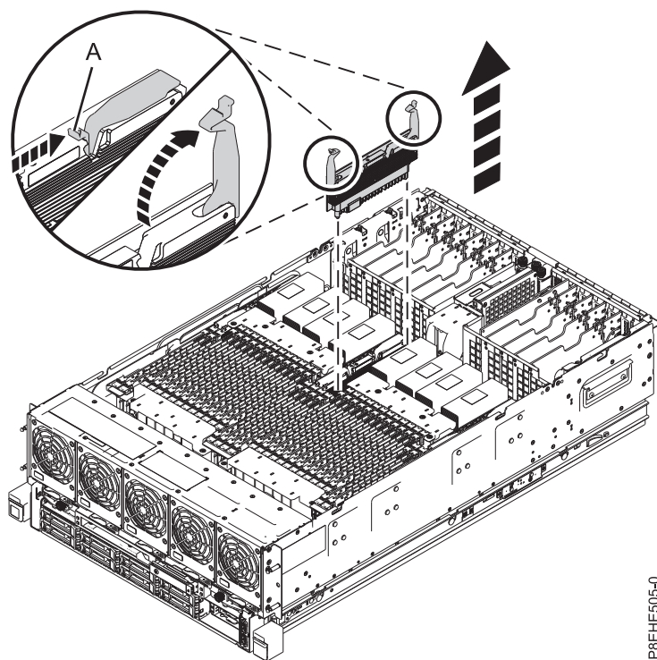
図 12. システムからのプロセッサ電圧調節モジュールの取り外し
