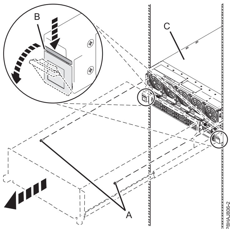
図 24. システムの保守位置への設置
