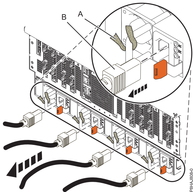
図 29. 8408-E8E システムからの電源コードの取り外し
