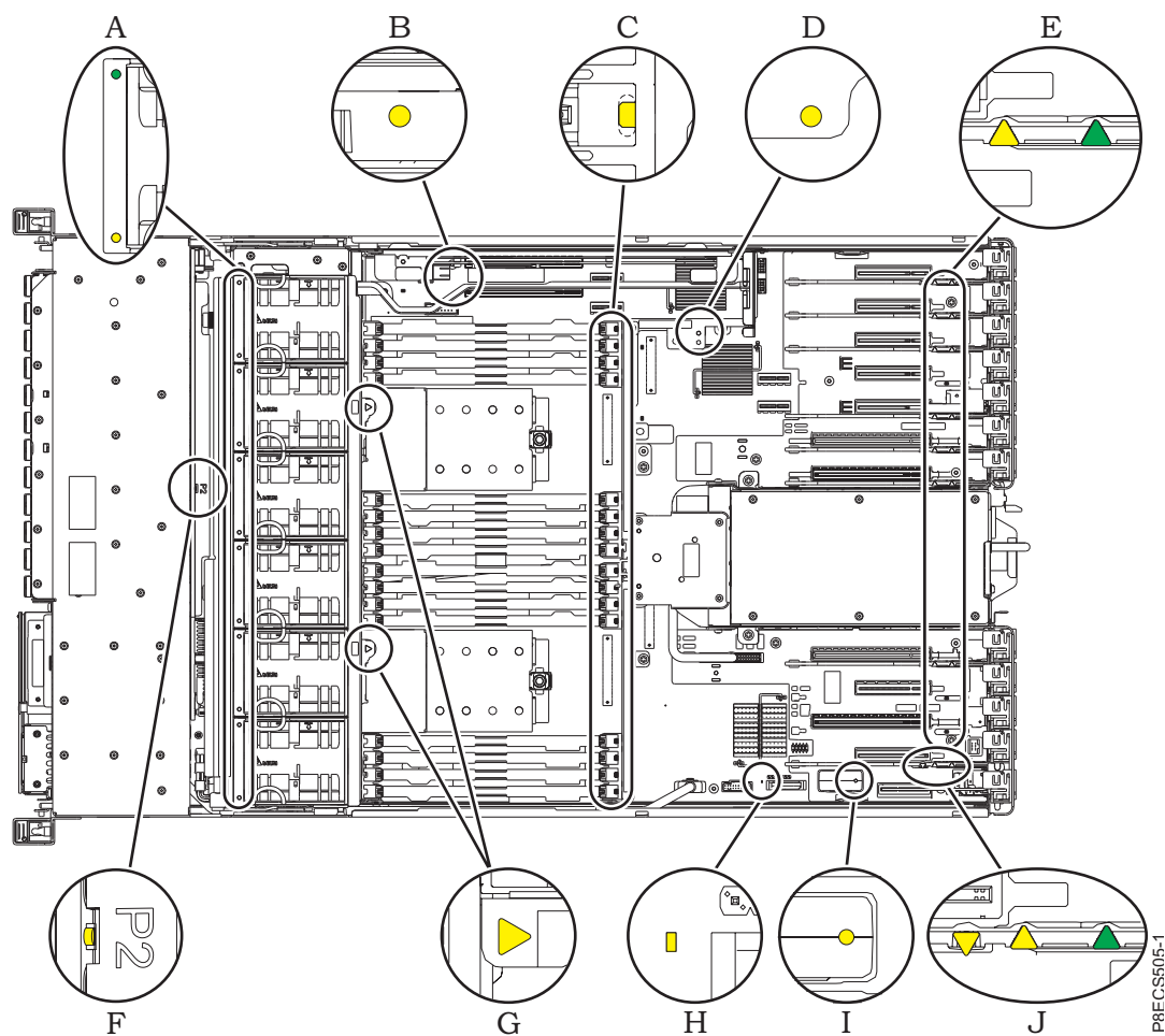
図 9. サービス・インジケータ LED
