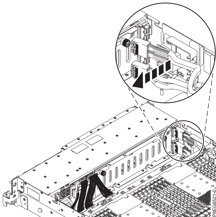
図 11. 前面 SAS ケーブルのガイド・ブロックからの取り外し
