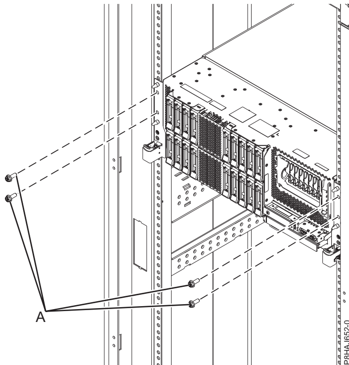
図 43. 前面のねじの取り外し
