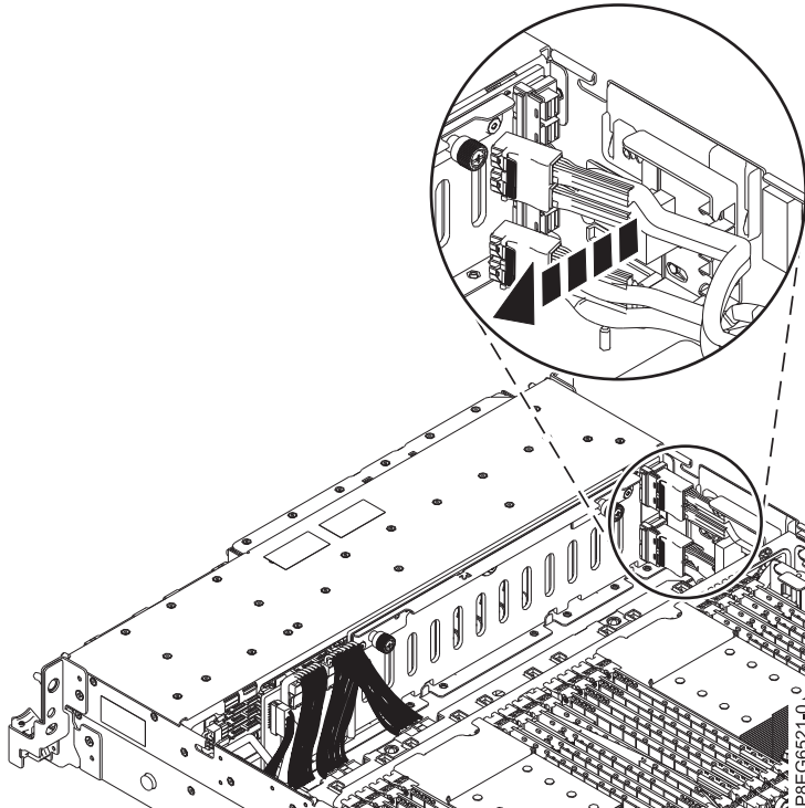
図 2. 前面 SAS ケーブルのガイド・ブロックからの取り外し
