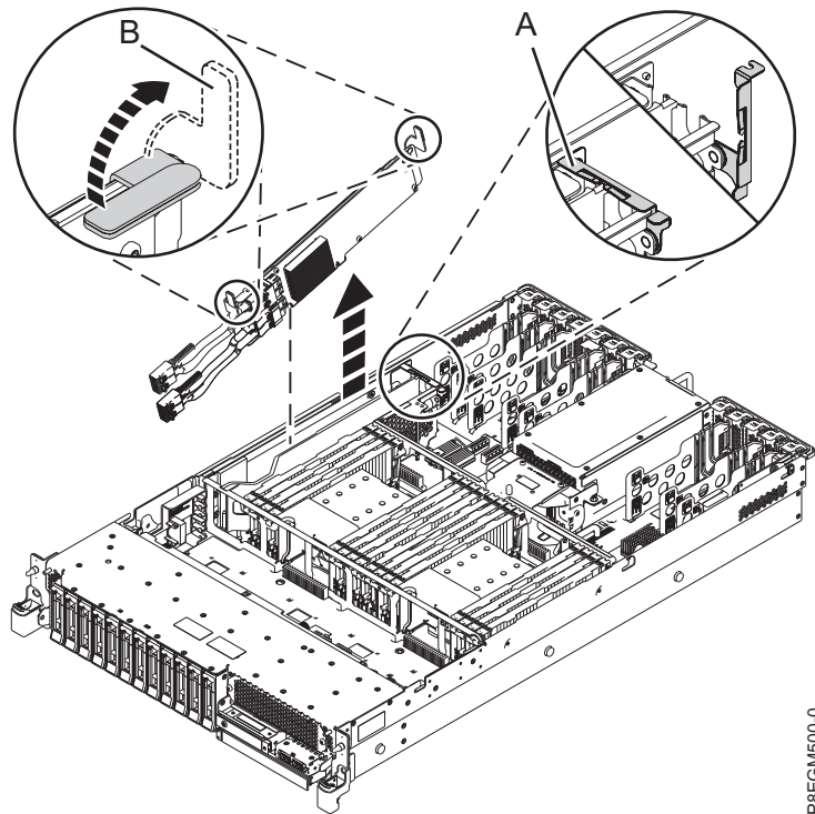
図 3. スロット P1-C14 の SAS RAID 内部アダプターの取り外し
