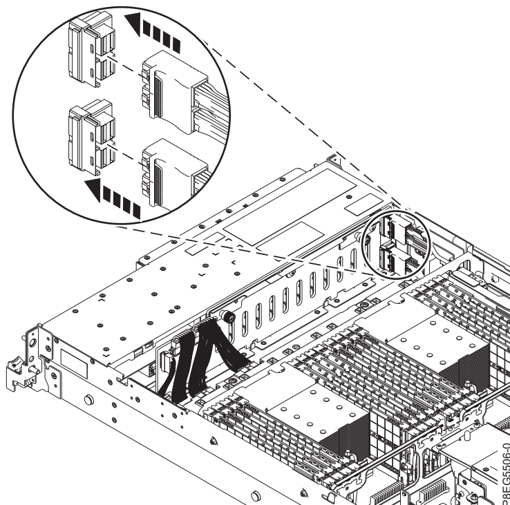
図 7. 前面 SAS ケーブルのディスク・ドライブ・バックプレーンへの再接続
