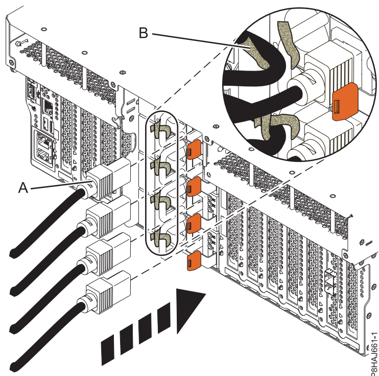
図 55. 8247-42L、8286-41A、または 8286-42A システムへの電源コードの接続
