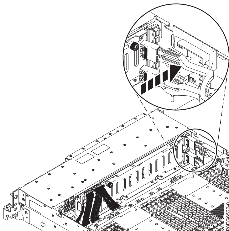
図 6. 前面 SAS ケーブルの配線
