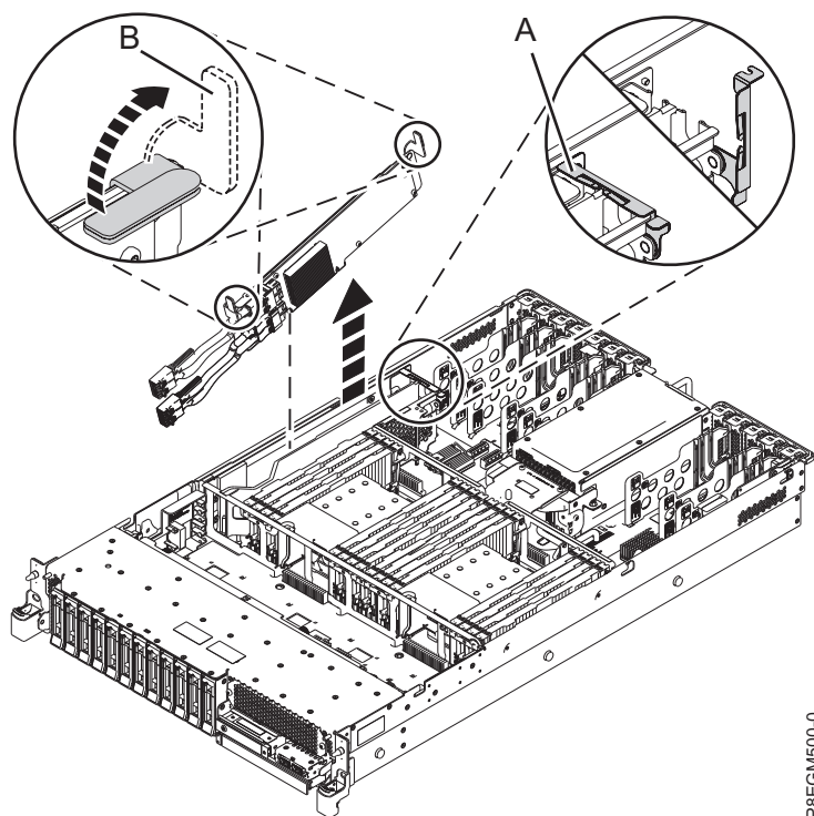
図 12. SAS RAID 内部アダプターの取り外し
