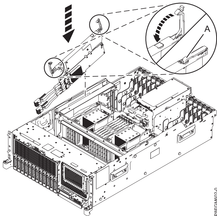
図 16. SAS RAID 内部アダプターの取り付け
