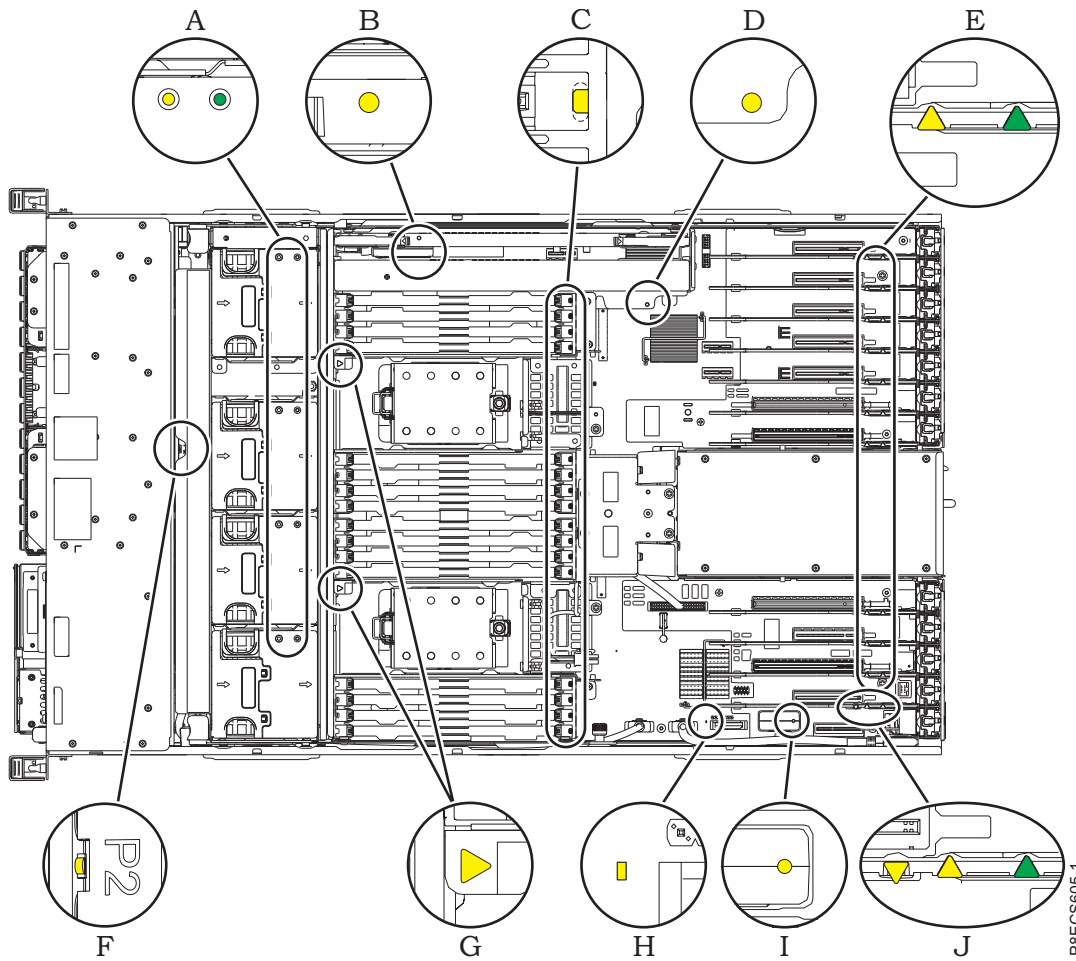
図 10. サービス・インジケター LED
