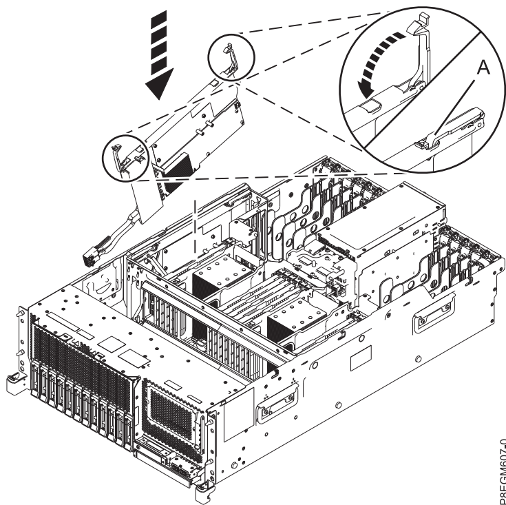
図 6. SAS RAID 内部アダプターのスロット P1-C15 への取り付け
