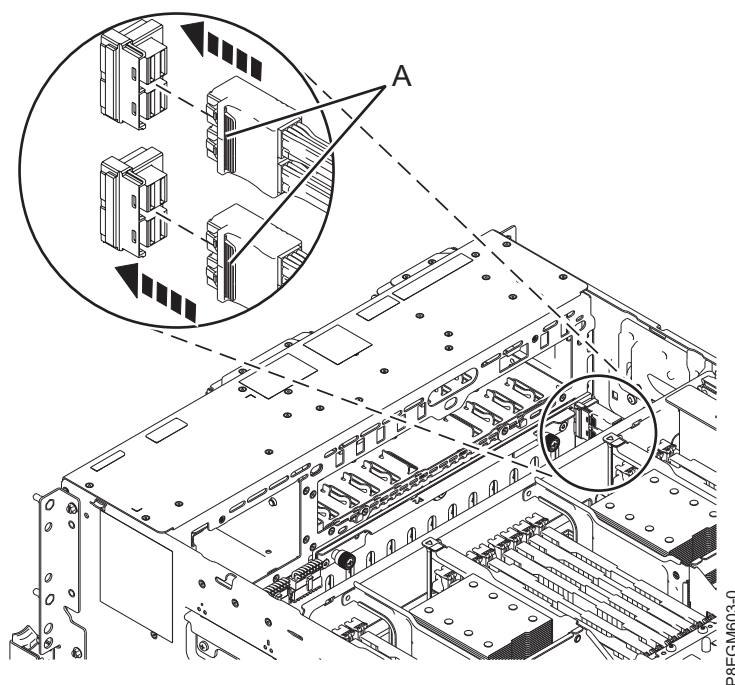
図 7. 前面 SAS ケーブルのディスク・ドライブ・バックプレーンへの接続
