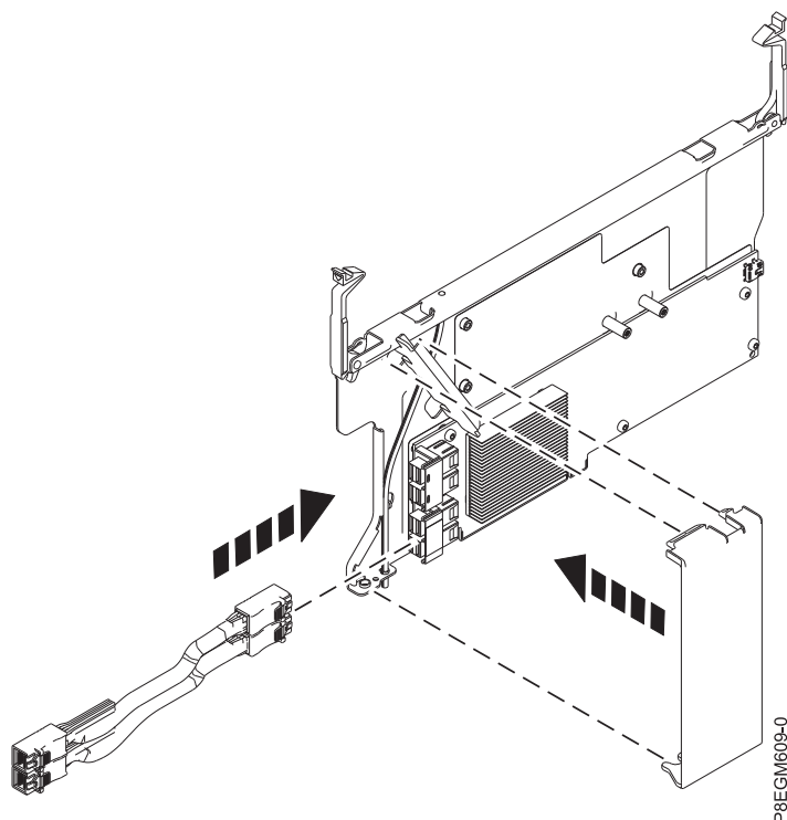
図 5. 通気カバーの取り付け
