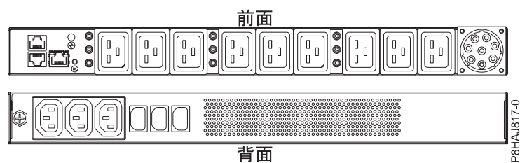
図 57. 8408-44E システムの PDU
