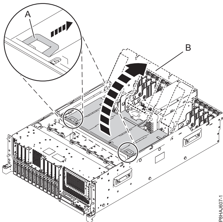
図 42. エア・バッフルのオープン
