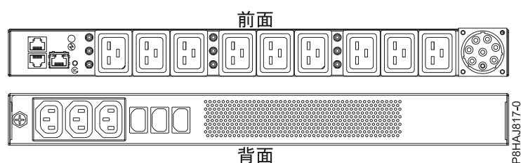
図 39. 8408-44E システムの PDU
