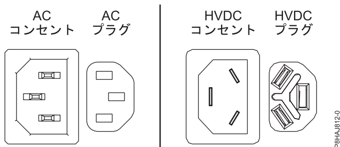
図 39. AC コネクターと HVDC コネクター
