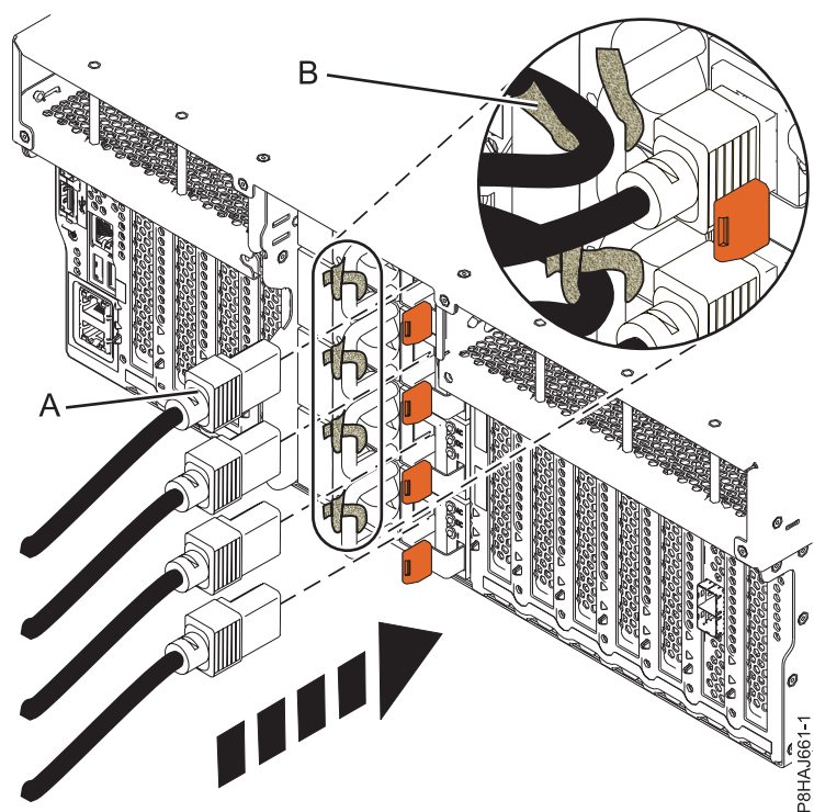
図 42. 8247-42L、8286-41A、または 8286-42A システムへの電源コードの接続
