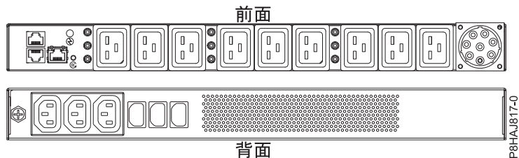
図 35. 8408-44E システムの PDU
