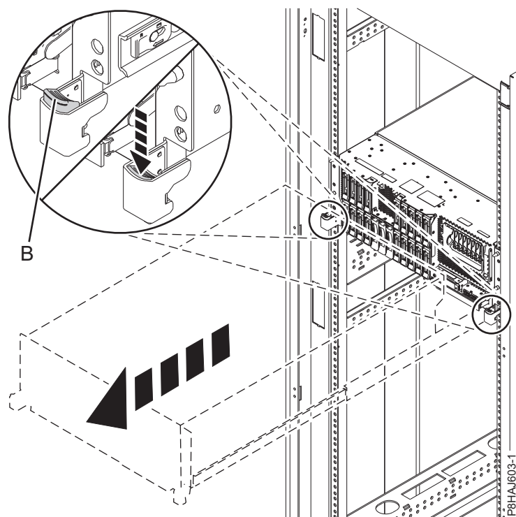
図 29. サイド・ラッチのリリース
