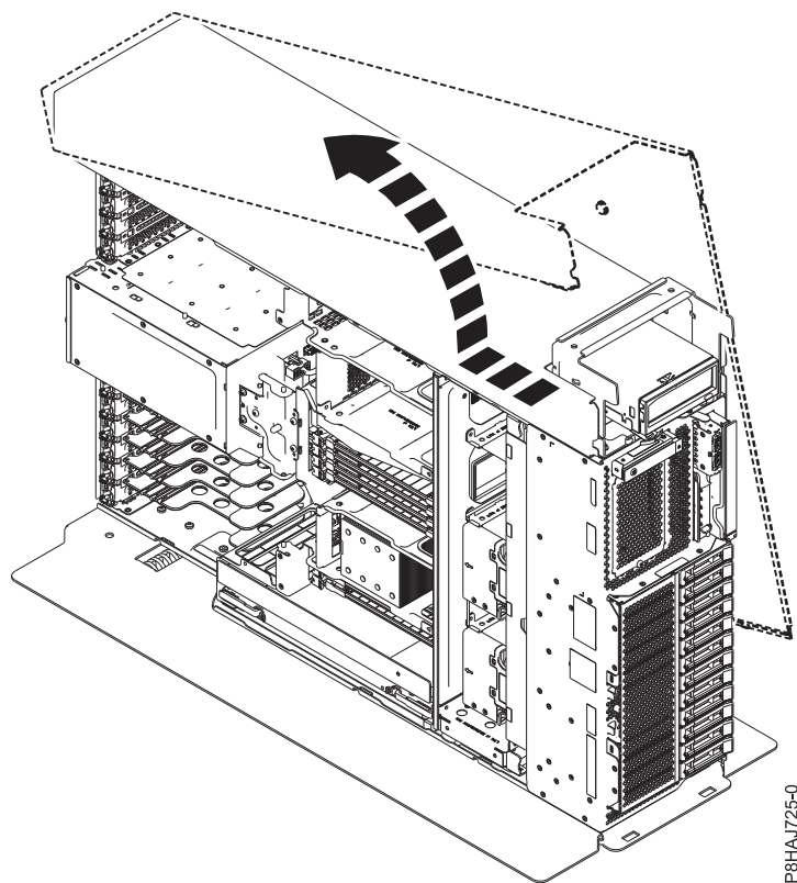
図 11. 8286-41A のサイド・カバーの取り外し
