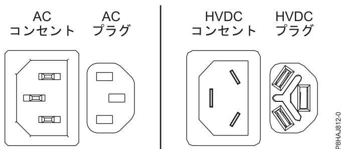
図 31. AC コネクターと HVDC コネクター
