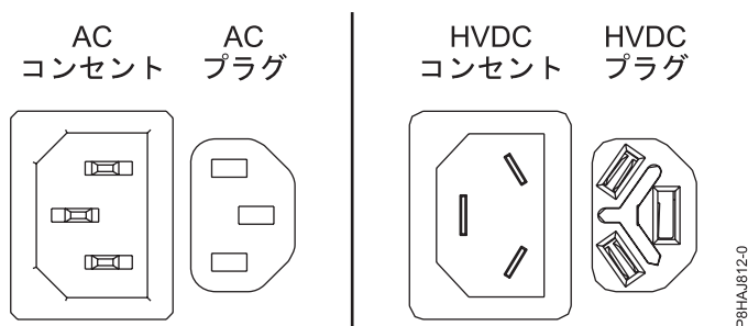
図 37. AC コネクターと HVDC コネクター
