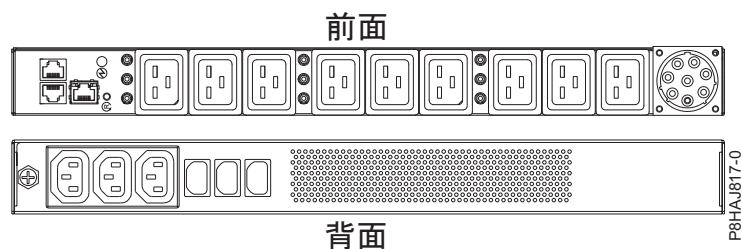
図 41. 8408-44E システムの PDU
