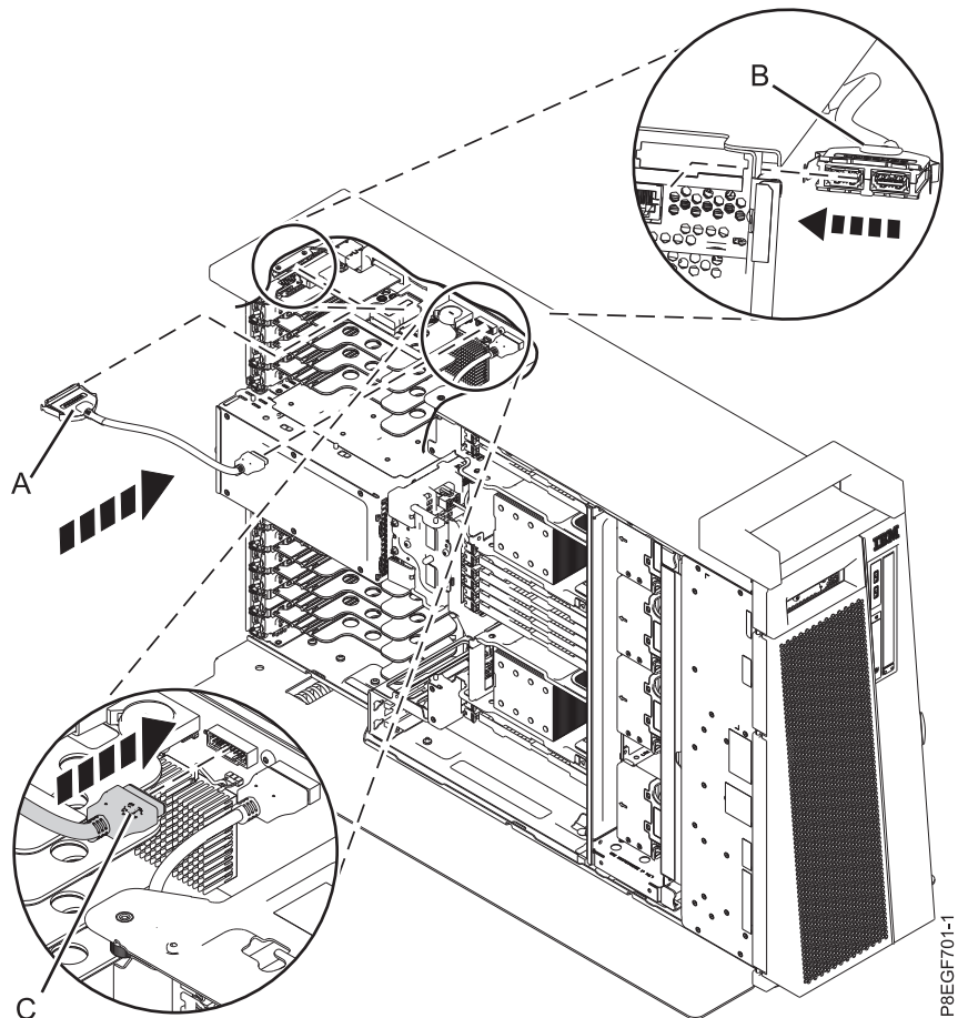
図 4. 8286-41A のスタンドアロン・バージョンでの背面 USB ケーブルの再取り付け
