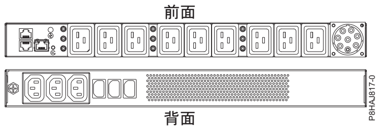
図 35. 8408-44E システムの PDU
