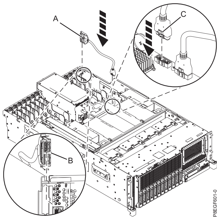
図 3. 背面 USB ケーブルの再取り付け
