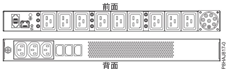
図 37. 8408-44E システムの PDU
