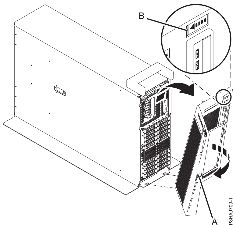
図 11. 前面カバーの取り外し
