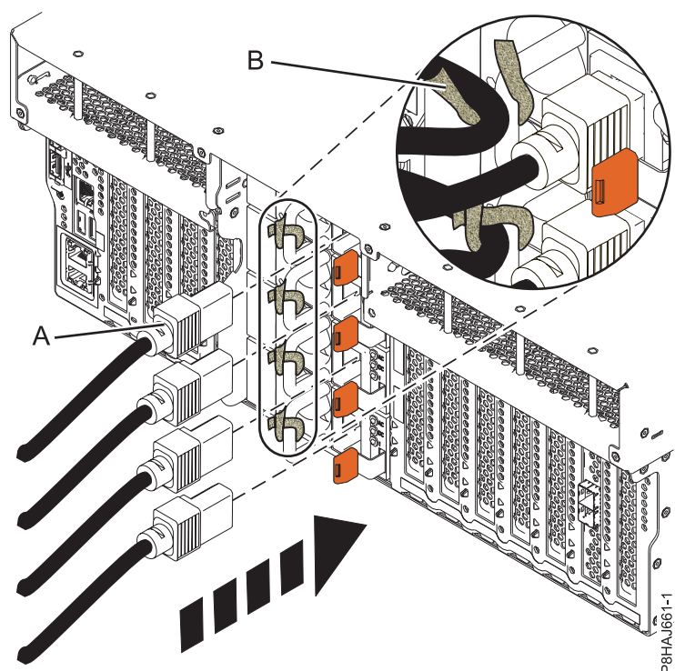
図 44. 8247-42L、8286-41A、または 8286-42A システムへの電源コードの接続
