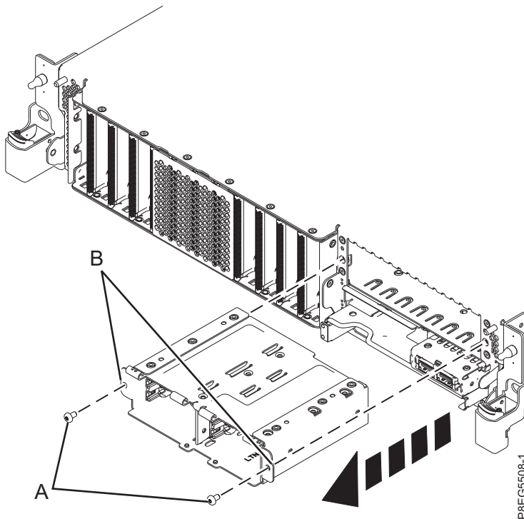
図 1. SSD ケージを部分的に引き出す
