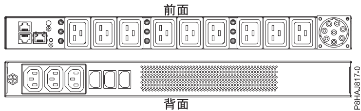
図 35. 8408-44E システムの PDU
