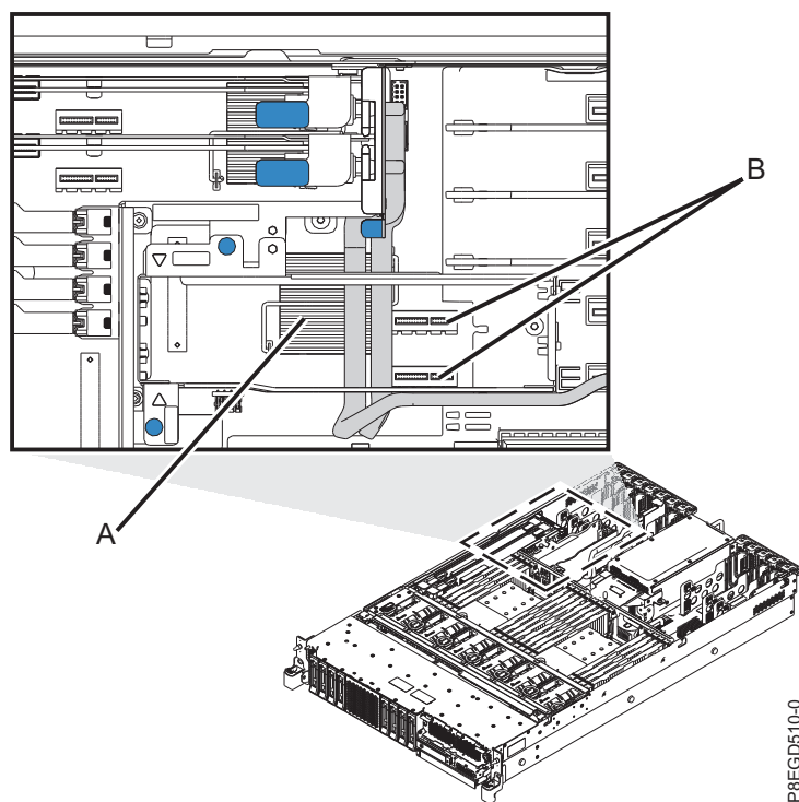
図 8. 背面 SAS ケーブルの配線
