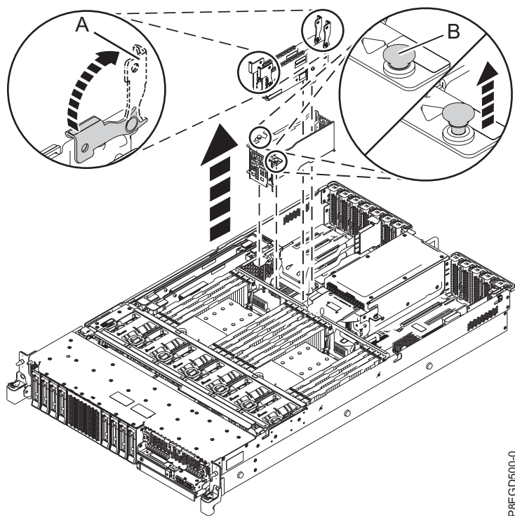
図 1. バックアップ電源モジュール・カードおよびケージの取り外し
