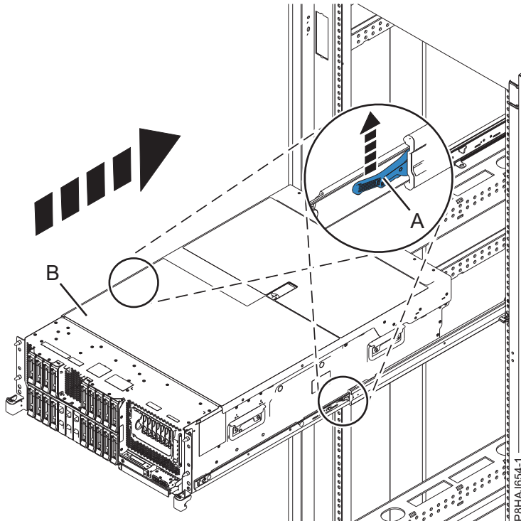
図 37. システムの操作位置への設置
