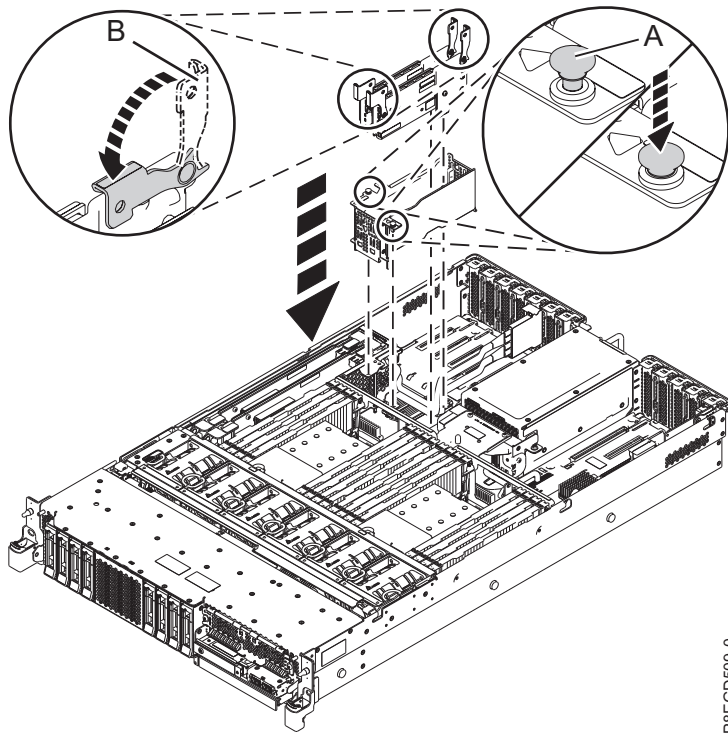
図 9. 電源モジュール・ケージの再取り付け
