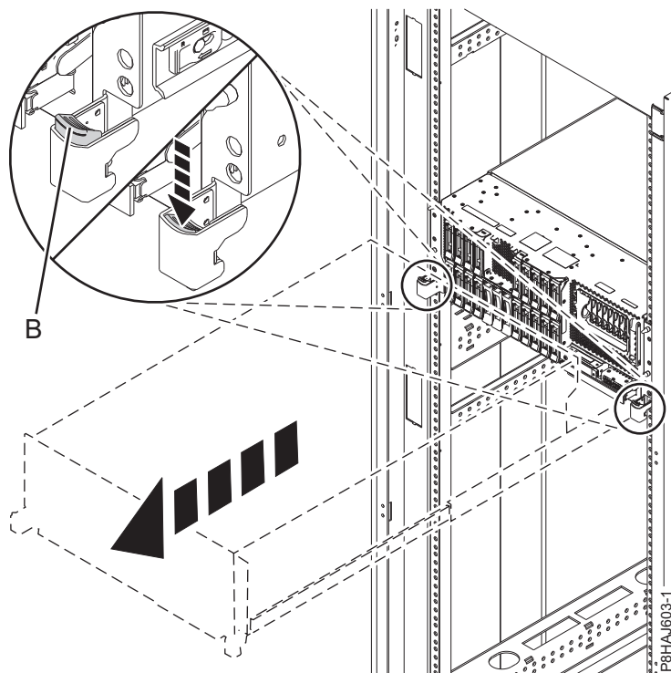
図 36. サイド・ラッチのリリース
