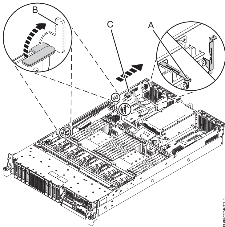
図 2. スロット位置 P1-C15 の SAS RAID 内部アダプターからの背面 SAS ケーブルの取り外し
