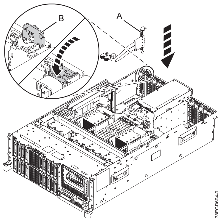
図 6. 背面 SAS ケーブルの取り付け
