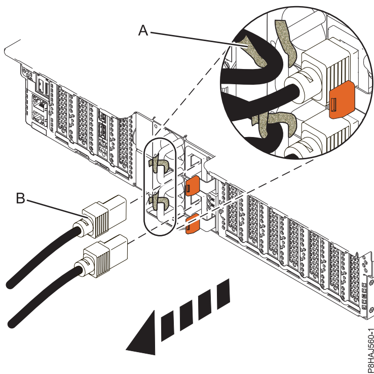
図 44. 5148-21L、5148-22L、8247-21L、8247-22L、8284-21A、または 8284-22A システムからの電源コードの取り外し
