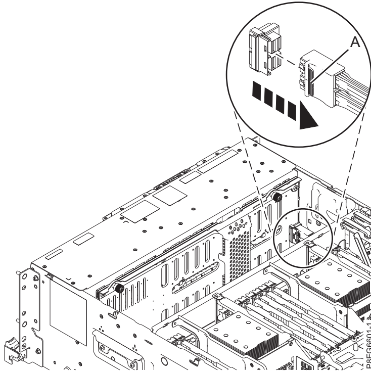
図 2. SAS ケーブルのプラグをディスク・ドライブ・バックプレーンから抜く
