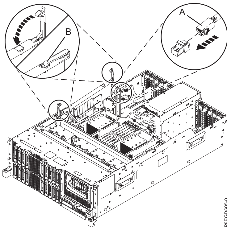
図 7. スロット P1-C14 の背面 SAS ケーブルの再取り付け
