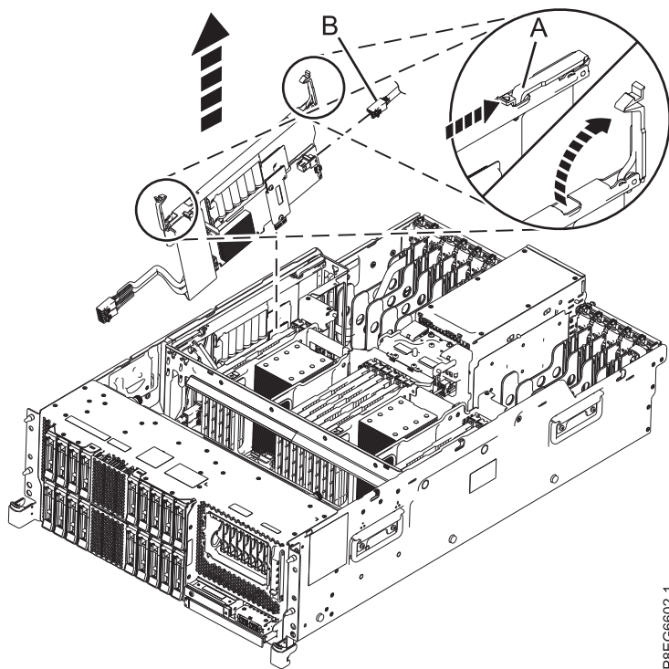
図 3. スロット P1-C15 の SAS RAID 内部アダプターの取り外し
