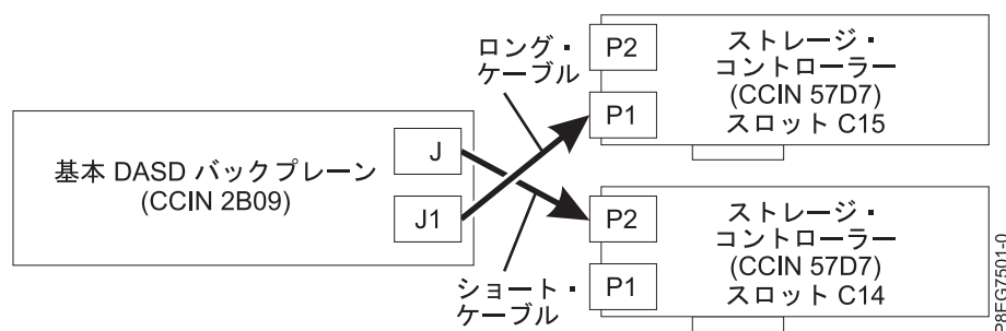
図 7. 分割ディスク構成での SAS ケーブルの再接続
