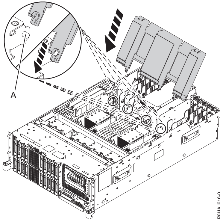
図 34. エア・バッフルの取り替え
