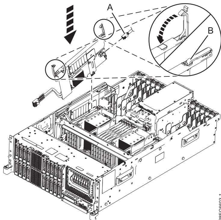
図 4. SAS RAID 内部アダプターの取り替え
