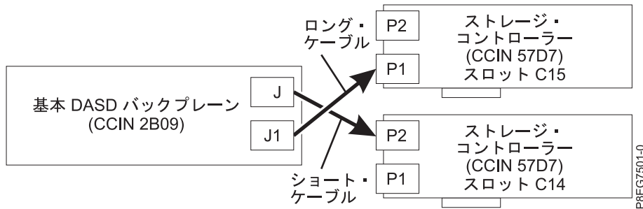
図 6. 分割ディスク構成での SAS ケーブルの再接続
