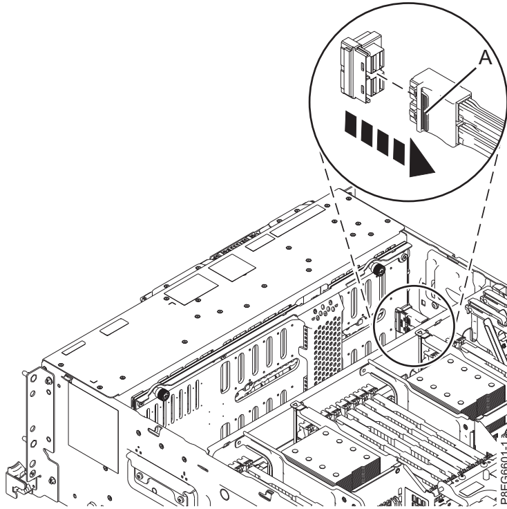
図 2. SAS ケーブルのプラグを抜く
