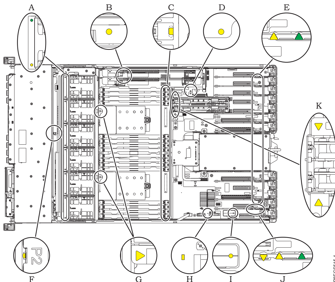
図 1. サービス・インディケーター LED
