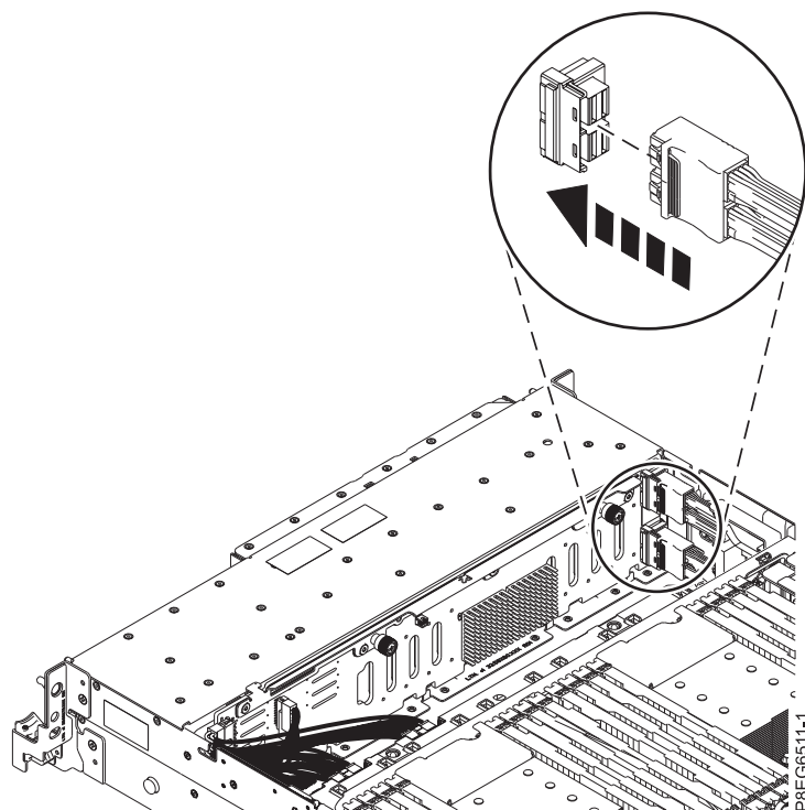
図 9. 前面 SAS ケーブルのディスク・ドライブ・バックプレーンへの再接続
