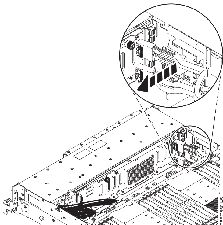
図 3. ケーブル・ガイドからの前面 SAS ケーブルの取り外し
