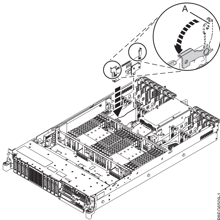
図 10. バックアップ電源モジュール・カードの再取り付け
