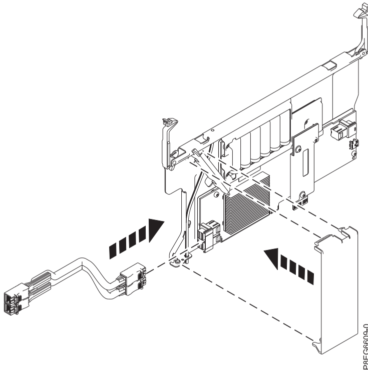
図 6. P1-C15 の位置に取り付けられた PCIe3 x8 キャッシュ SAS RAID 内部アダプター 6 Gb への通気カバーの取り付け
