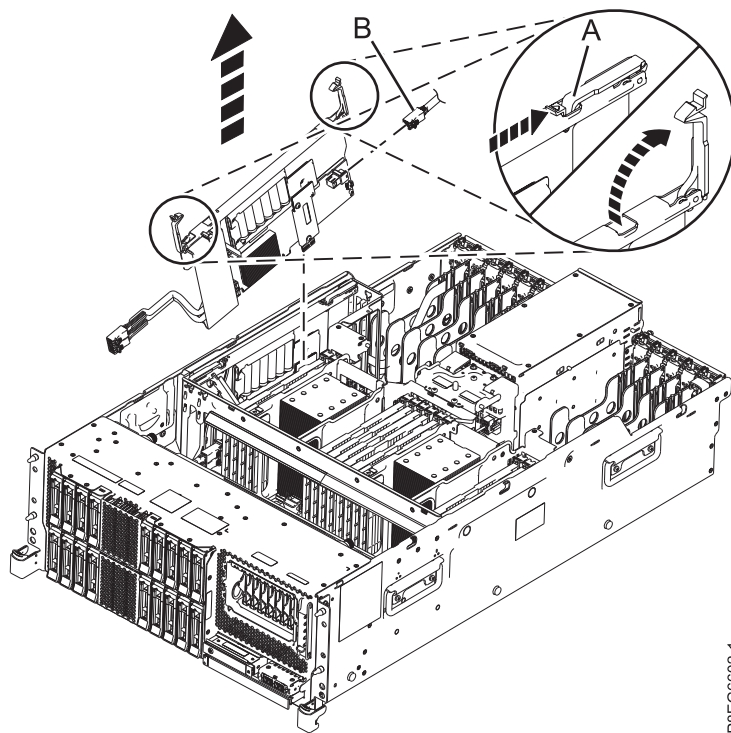
図 4. PCIe x8 キャッシュ SAS RAID 内部アダプター 6 Gb の取り外し
