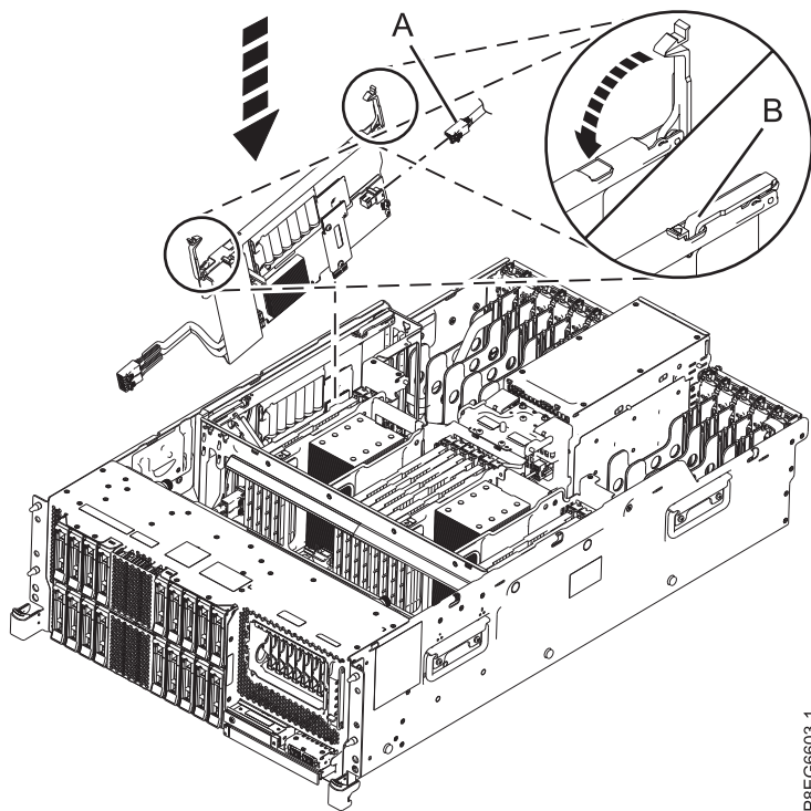
図 7. PCIe3 x8 キャッシュ SAS RAID 内部アダプター 6 Gb の取り替え
