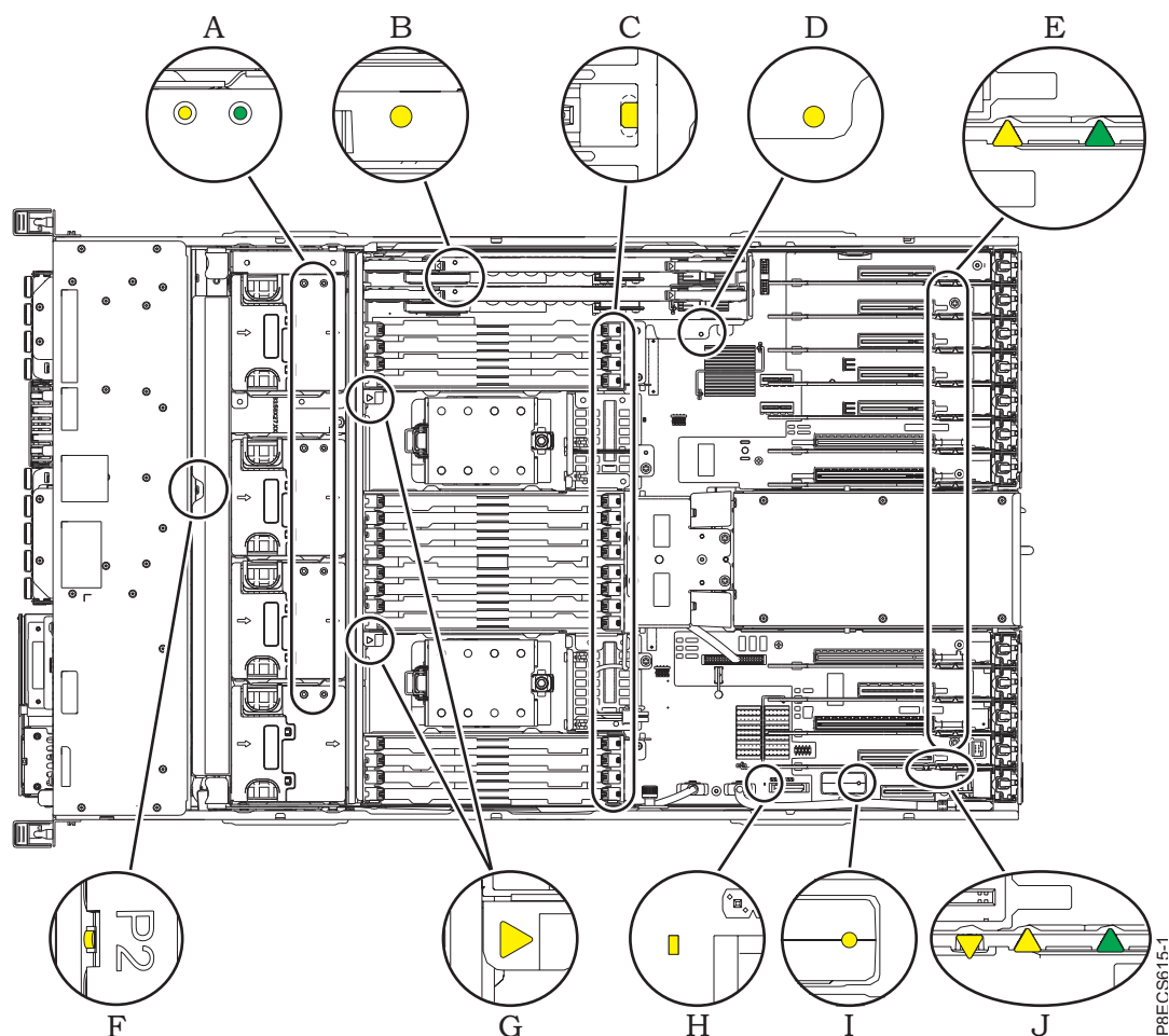
図 1. サービス・インディケーター LED
