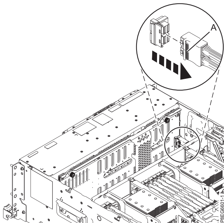
図 3. SAS ケーブルのプラグをディスク・ドライブ・バックプレーンから抜く
