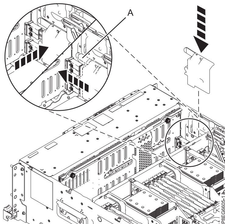
図 10. SAS ケーブル・カバーの再取り付け
