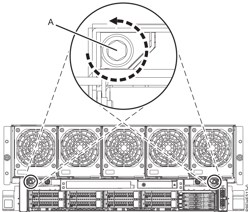
図 2. 配送用ねじを緩める
