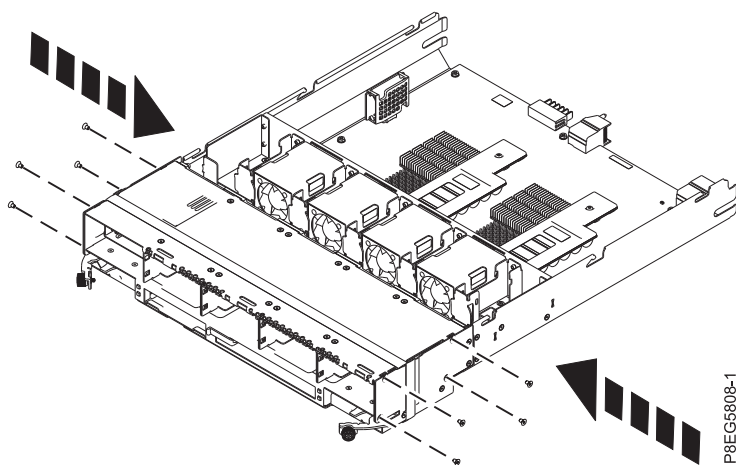
図 15. ねじの再取り付け
