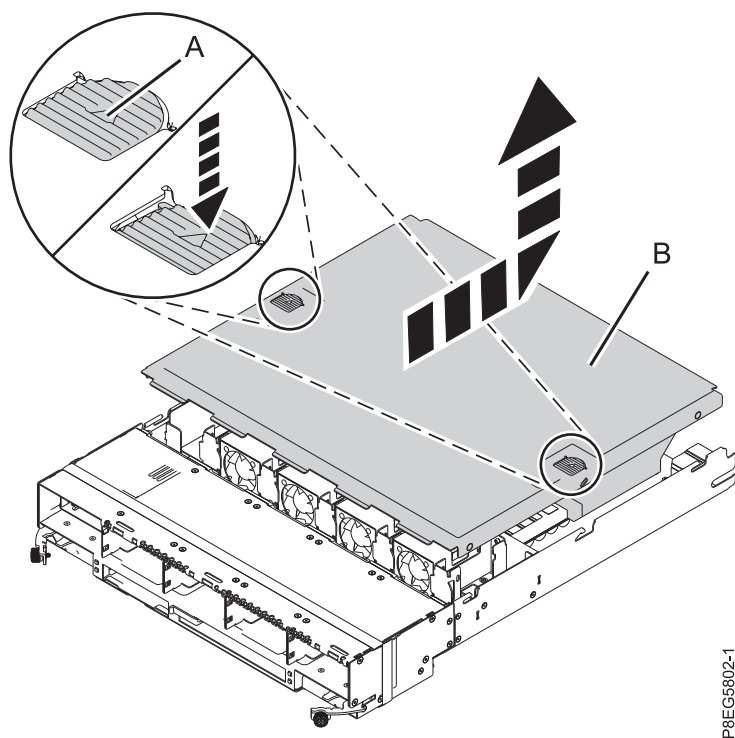
図 9. RAID アセンブリー・カバーの取り外し
