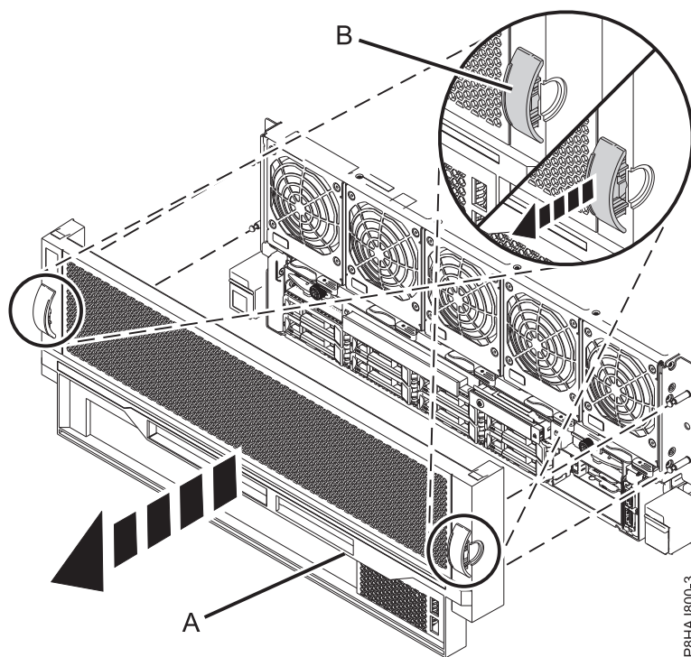
図 37. 前面カバーの取り外し
