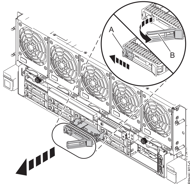
図 5. ディスク・ドライブの取り外し
