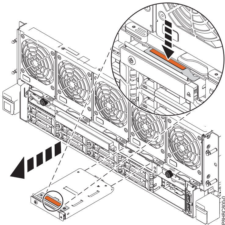
図 3. コントロール・パネルの取り外し
