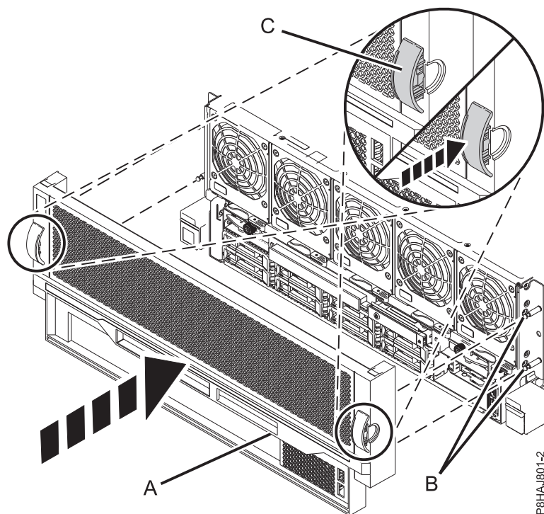
図 38. 前面カバーの取り付け
