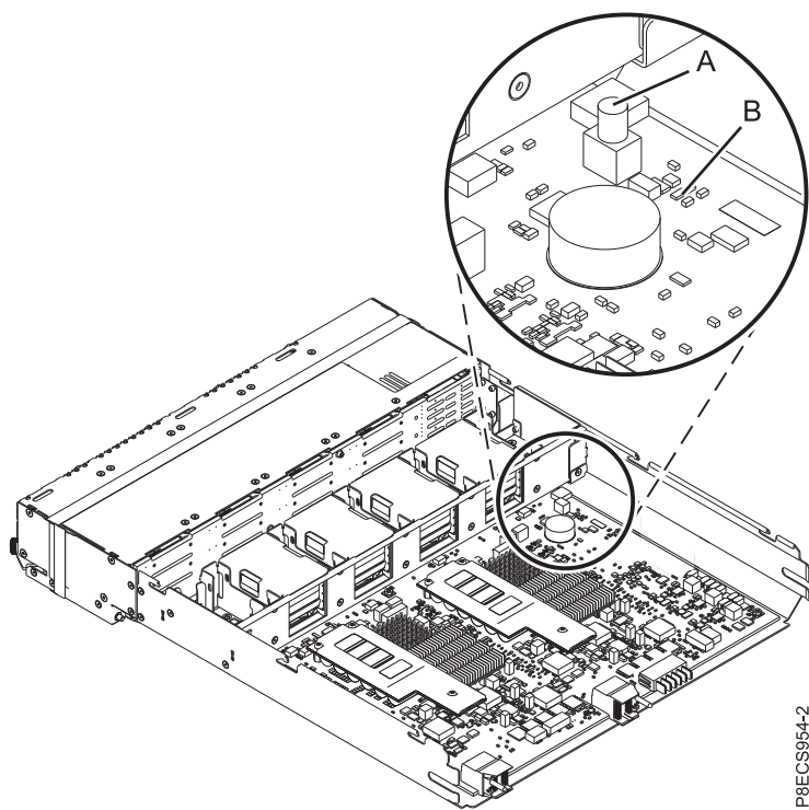
図 10. 識別 LED の活動化
