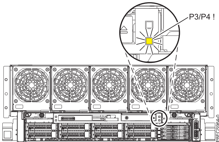
図 1. 8408-44E または 8408-E8E システム上の前面「P3/P4 !」 障害ロールアップ LED
