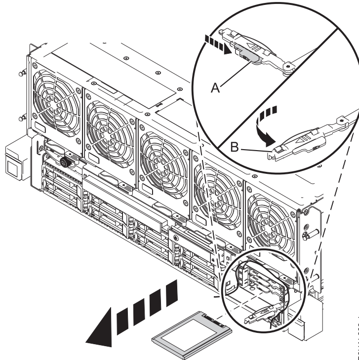
図 6. ソリッド・ステート・ドライブの取り外し
