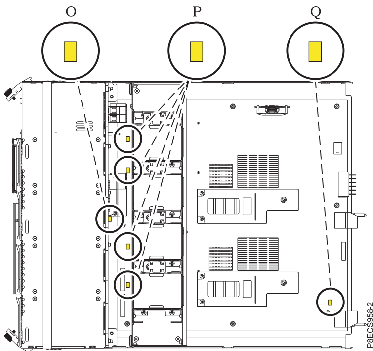
図 11. サービス・インディケータ LED
