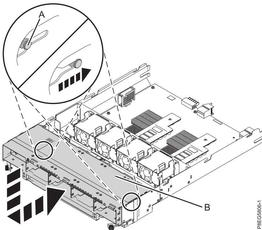
図 14. ディスク・ドライブ・バックプレーンの再取り付け
