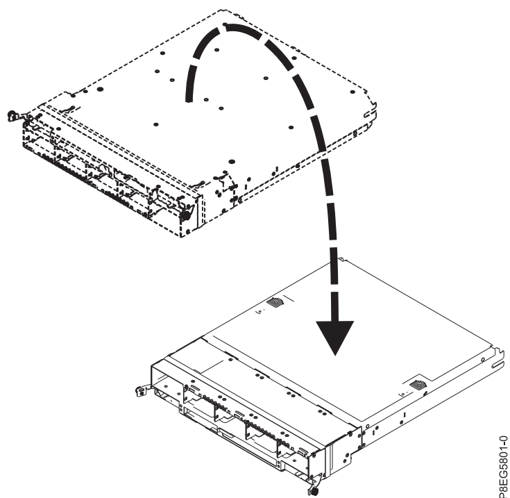
図 8. RAID アセンブリーの反転
