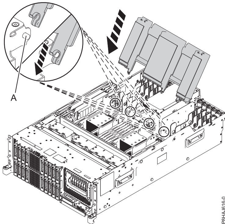
図 48. エア・バッフルの取り替え
