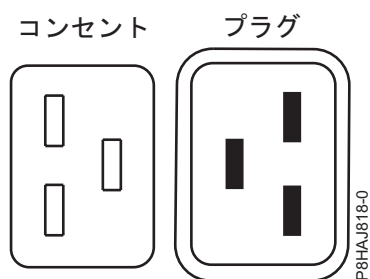
図 51. 8408-44E システムのコネクター
