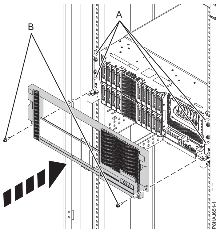
図 32. 前面カバーの取り付け
