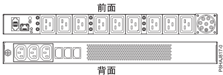
図 52. 8408-44E システムの PDU
