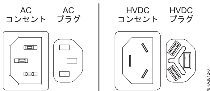
図 56. AC コネクターと HVDC コネクター
