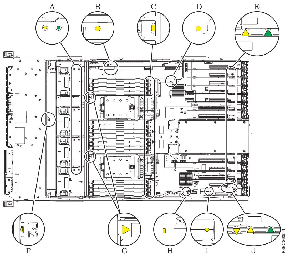
図 1. サービス・インジケター LED
