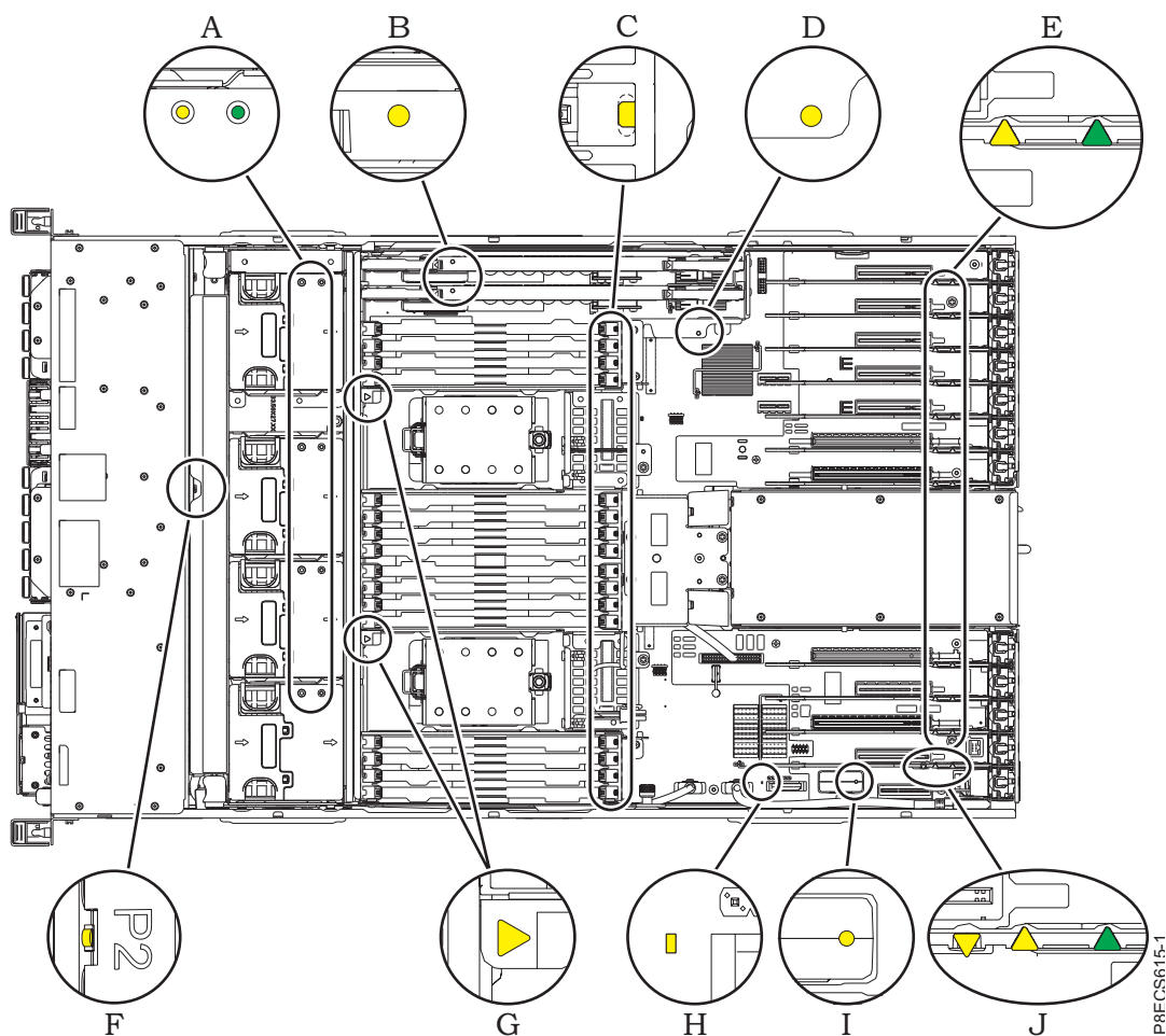
図 12. サービス・インジケター LED
