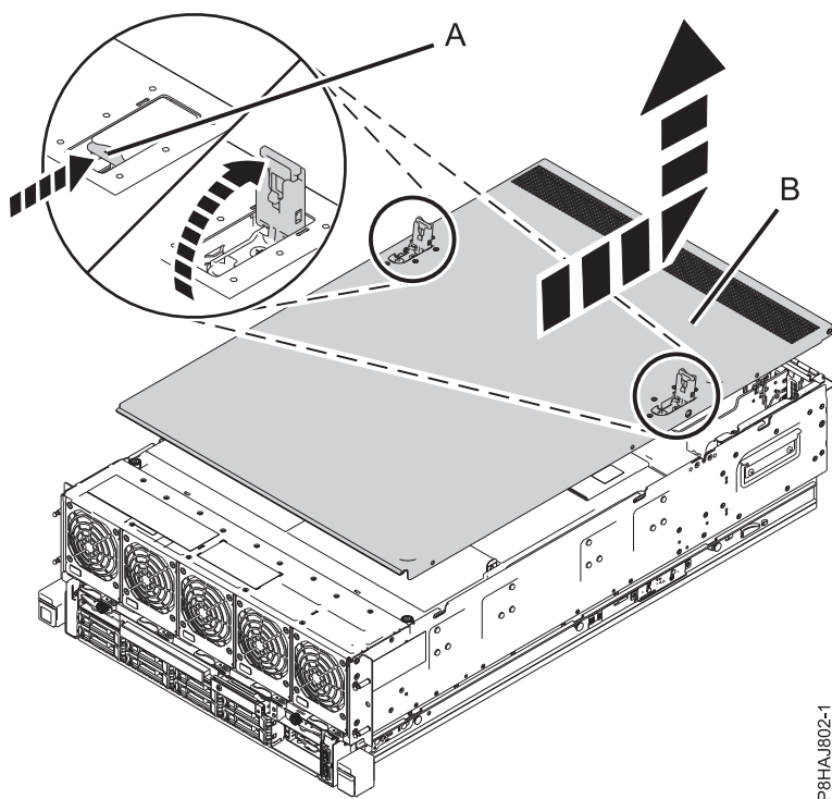
図 8. 保守アクセス・カバーの取り外し
