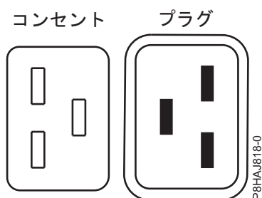
図 17. 8408-44E システムのコネクター
