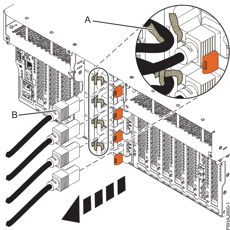
図 19. 8247-42L、8286-41A、または 8286-42A システムからの電源コードの取り外し
