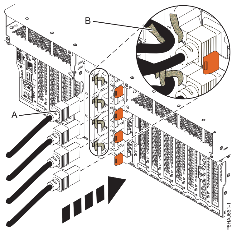
図 25. 8247-42L、8286-41A、または 8286-42A システムへの電源コードの接続
