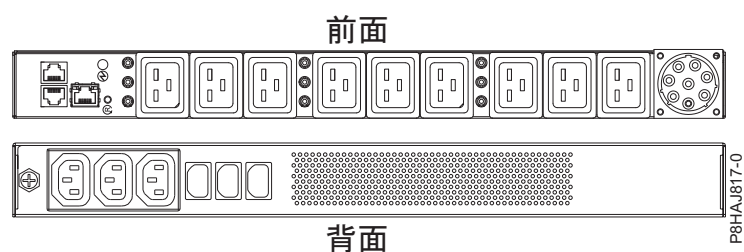
図 24. 8408-44E システムの PDU
