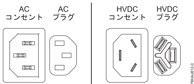
図 16. AC コネクターと HVDC コネクター
