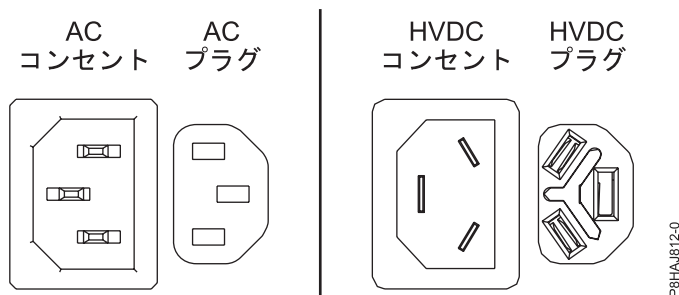
図 22. AC コネクタと HVDC コネクタ
