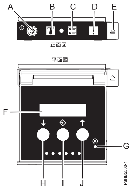
図 5. コントロール・パネル
