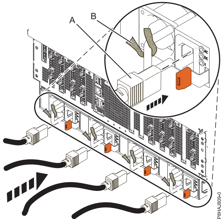
図 27. 8408-44E または 8408-E8E システムへの電源コードの接続
