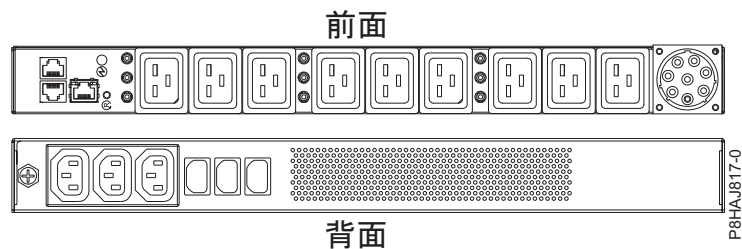
図 18. 8408-44E システムの PDU
