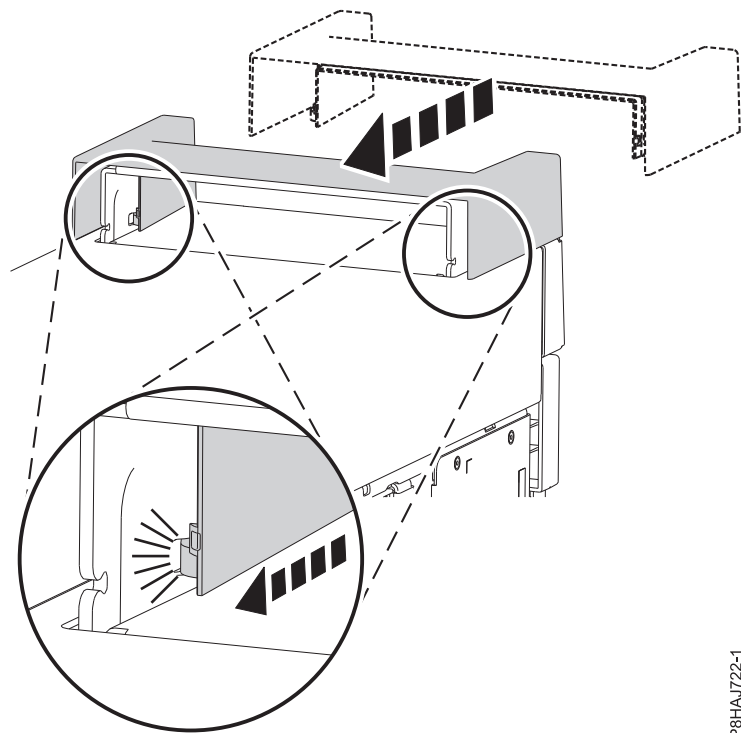
図 16. 8286-41A スタンドアロン・システムへのハンドル・カバーの固定
