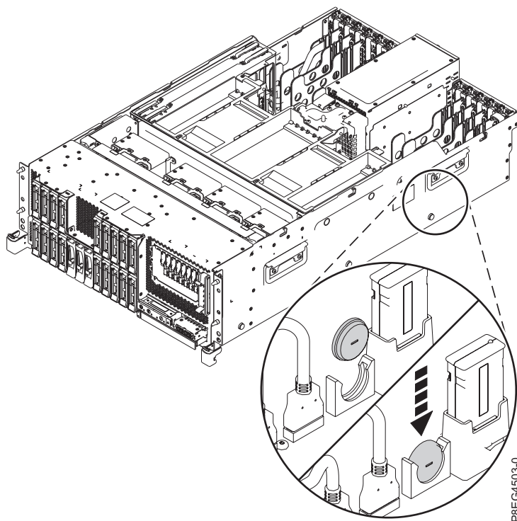
図 2. 時刻バッテリーの挿入
