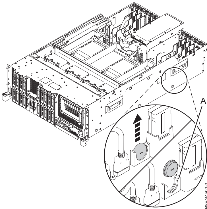
図 1. 時刻バッテリーの取り外し
