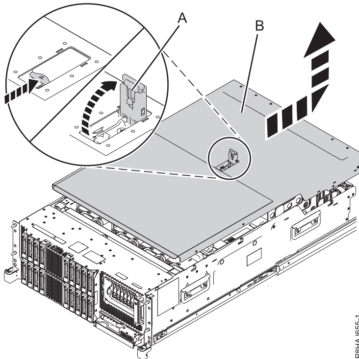
図 20. 保守アクセス・カバーの取り外し
