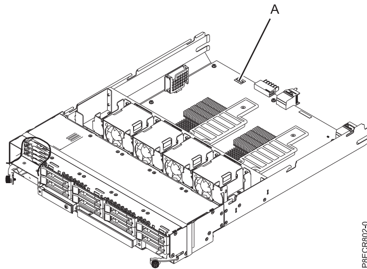
図 5. 書き込みキャッシュ構成のないデュアル RAID コントローラーを備えた SAS サブシステム (FC EPVP)。CCIN 2CD2 はラベル (A) に記載されています。
