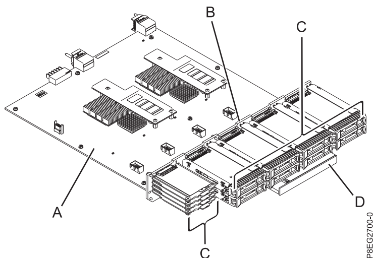
図 1. 書き込みキャッシュ構成を持つデュアル RAID コントローラーを使用するシステム内の SAS サブシステム部品 部品のリストと各部品の位置については、図 1 と一緒に表 1 を使用してください。
