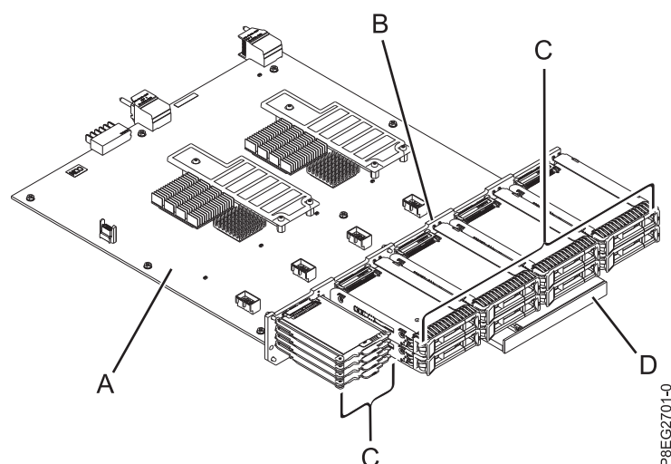
図 2. 書き込みキャッシュ構成のないデュアル RAID コントローラー内の SAS サブシステム部品
