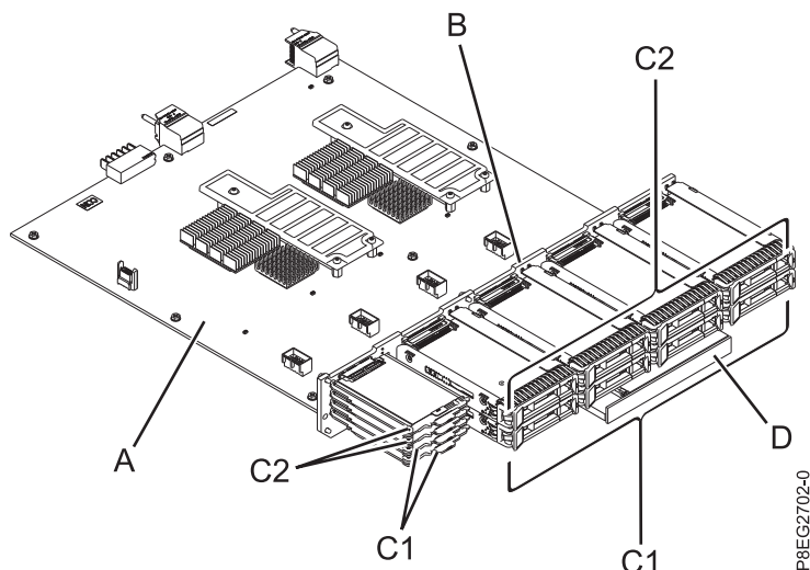
図 3. 書き込みキャッシュ構成のない 2 つの RAID コントローラーを備えた分割ストレージ・バックプレーン内の SAS サブシステム部品
