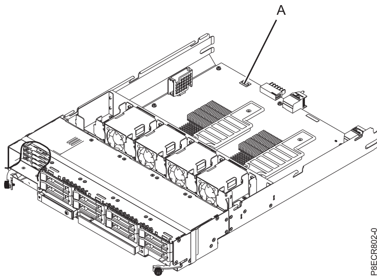
図 6. 書き込みキャッシュ構成のない 2 つの RAID コントローラーを備えた分割バックプレーン付きの SAS サブシステム (FC EPVQ)。CCIN 2CCD はラベル (A) に記載されています。
