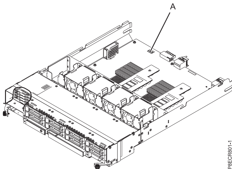
図 4. デュアル書き込みキャッシュのある SAS サブシステム構成 (FC EPVN)。CCIN 2CCA はラベル (A) に記載されています。
