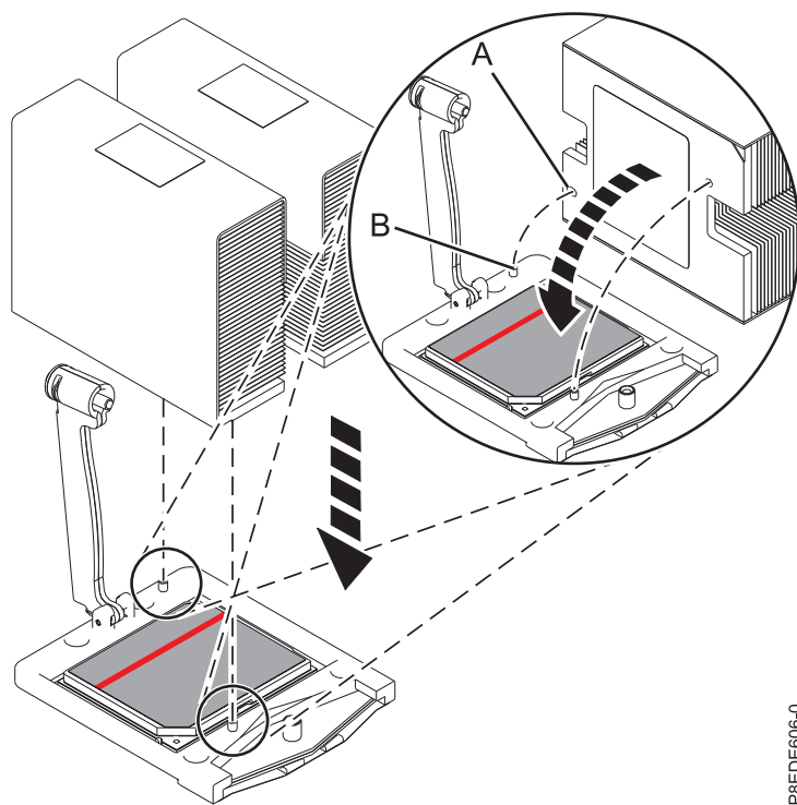
図 19. ヒート・シンクの取り付け
