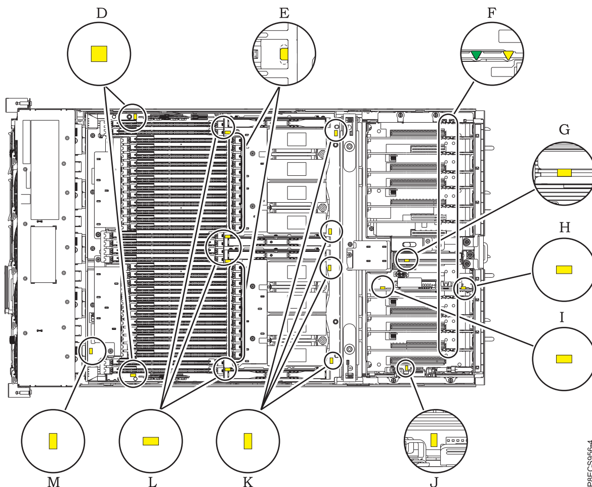
図 3. サービス・インディケーター LED
