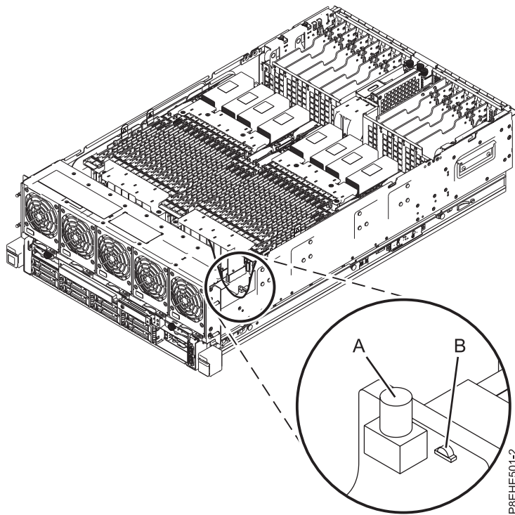
図 2. 識別 LED の活動化
