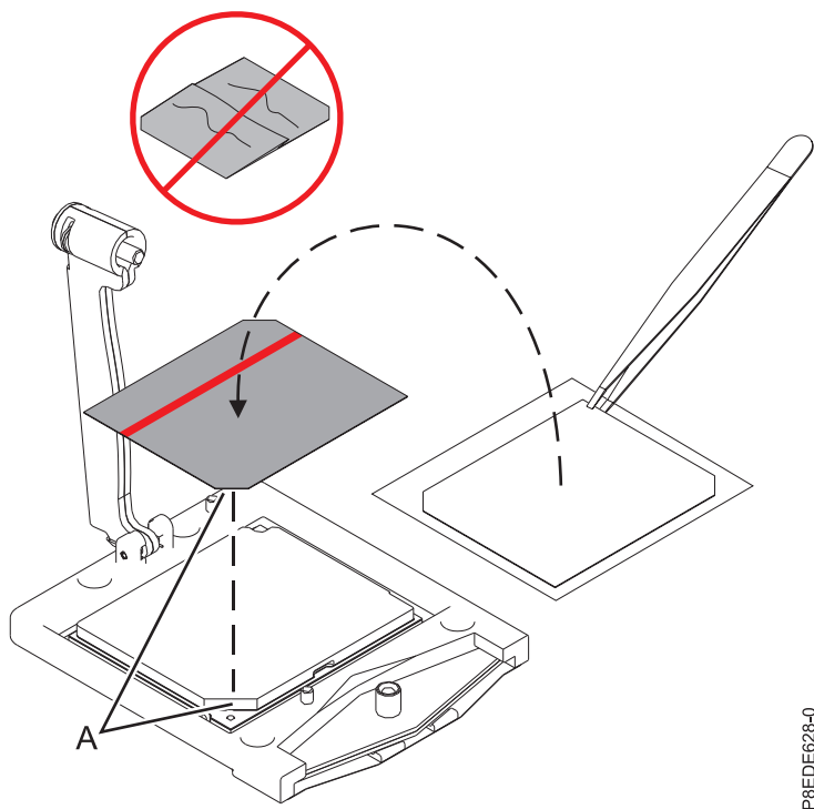
図 18. 熱伝導材料の取り付け
