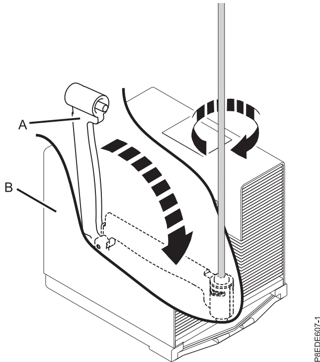
図 20. ロード・アームのねじを締める
