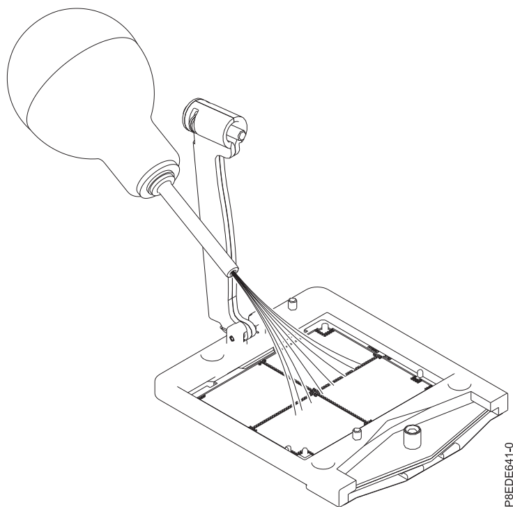
図 15. システム・プロセッサ・ソケットからほこりやごみを除去
