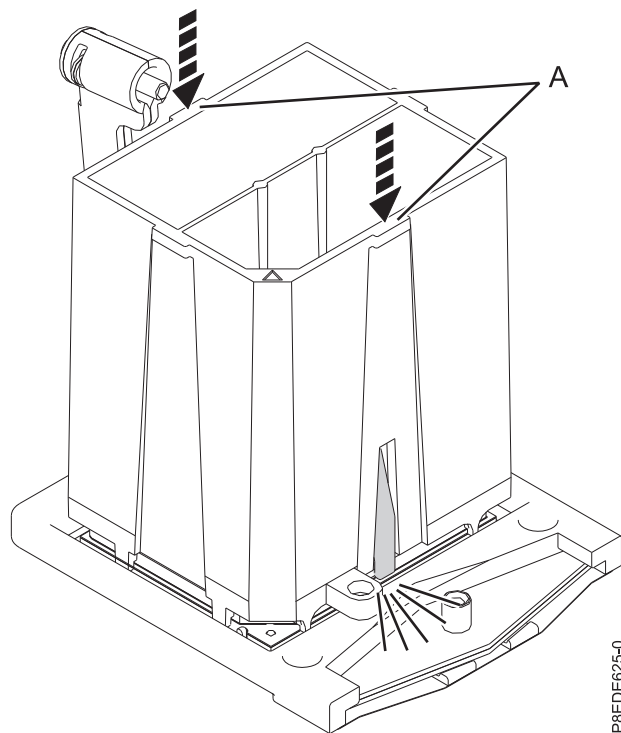
図 9. システム・プロセッサ・モジュールを取り外しツールにロック
