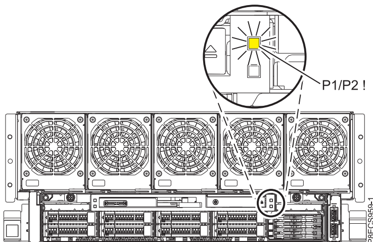
図 1. 8408-44E または 8408-E8E システム上の前面 P1/P2 ! 障害ロールアップ LED
