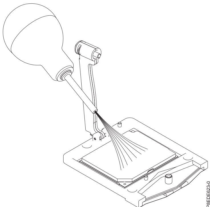
図 7. システム・プロセッサ・モジュールの領域のクリーニング
