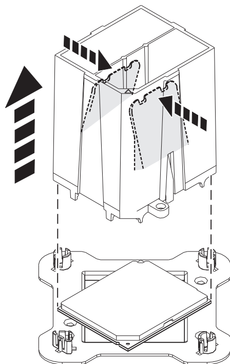
図 11. ツールからのシステム・プロセッサ・モジュールの解放
