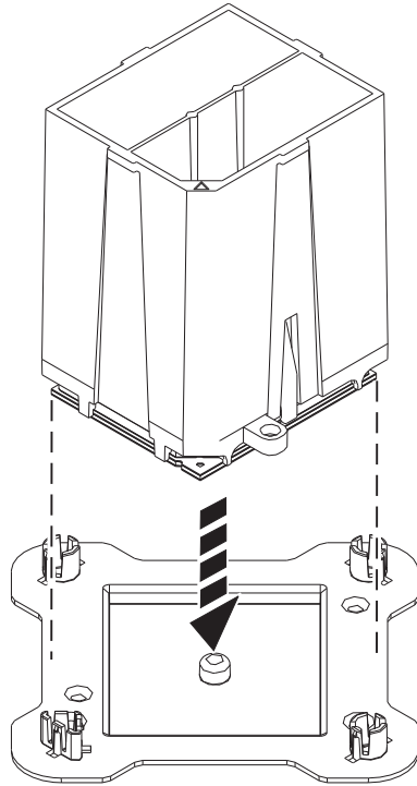
図 10. パッケージのトップ・カバーへのシステム・プロセッサ・モジュールの配置
