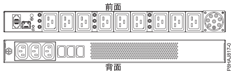
図 36. 8408-44E システムの PDU
