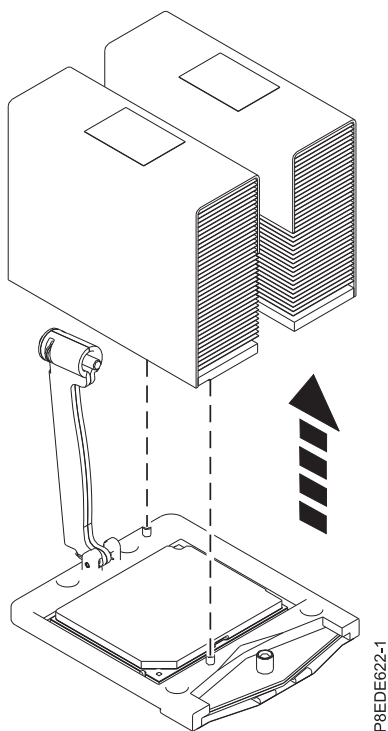
図 6. ヒート・シンクの取り外し
