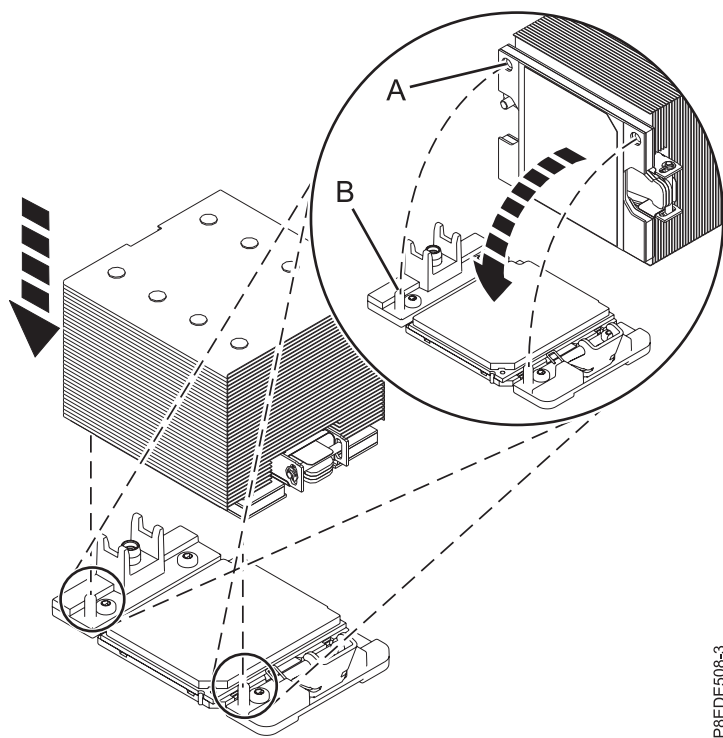
図 18. ヒート・シンクの取り付け
