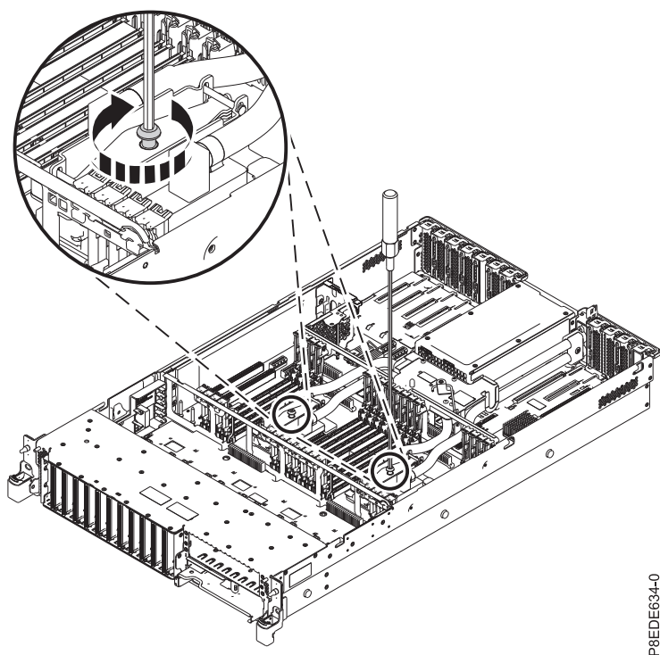
図 42. 冷却プレートの保持ねじを締める
