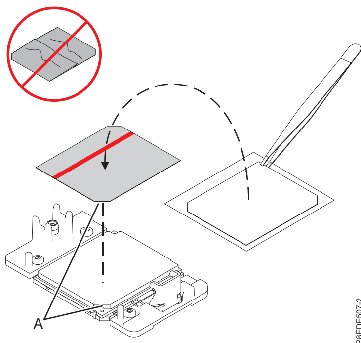
図 17. TIM をプロセッサのふたに取り付ける
