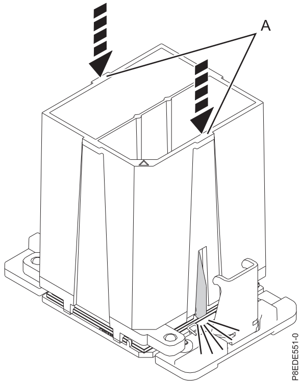
図 30. システム・プロセッサ・モジュールをツールにロック
