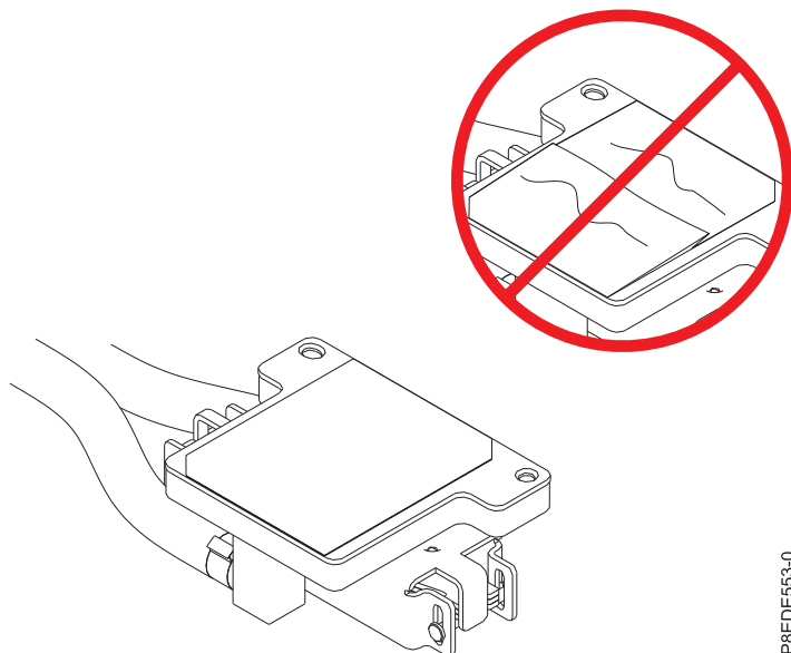
図 39. 熱伝導材料 (TIM) の検査
