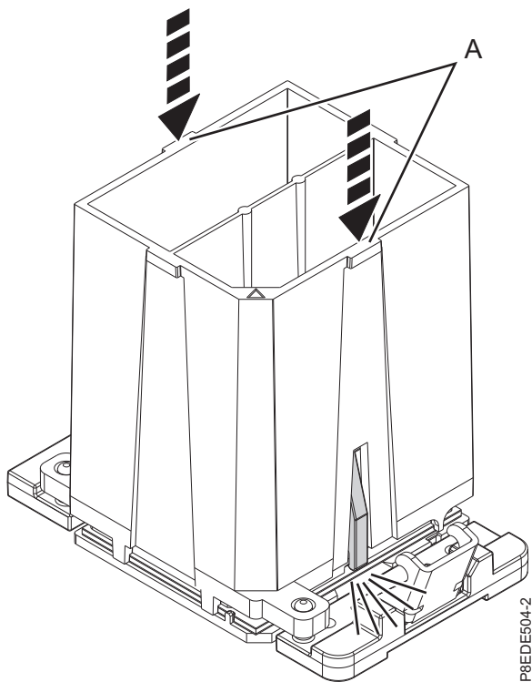
図 7. システム・プロセッサ・モジュールをツールにロック
