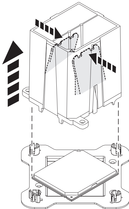
図 32. ツールからのシステム・プロセッサ・モジュールの解放
