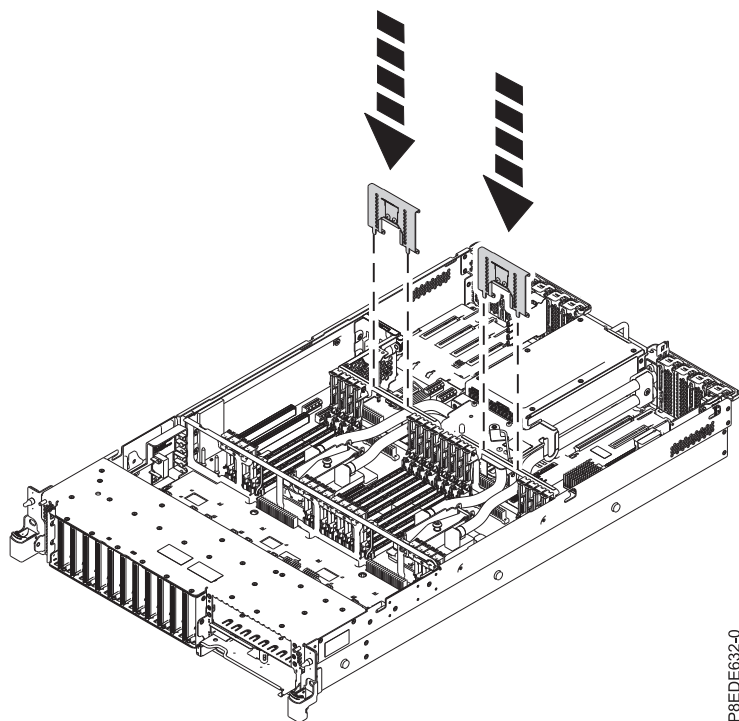
図 44. バッフルを下げて所定の位置に入れる
