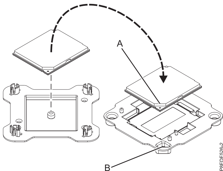
図 45. パッケージへのシステム・プロセッサ・モジュールの取り付け
