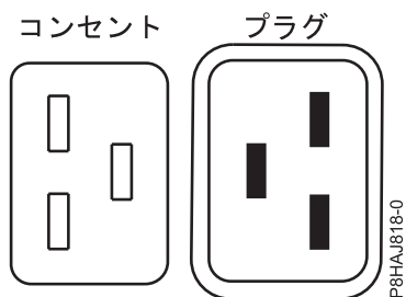
図 81. 8408-44E システムのコネクター
