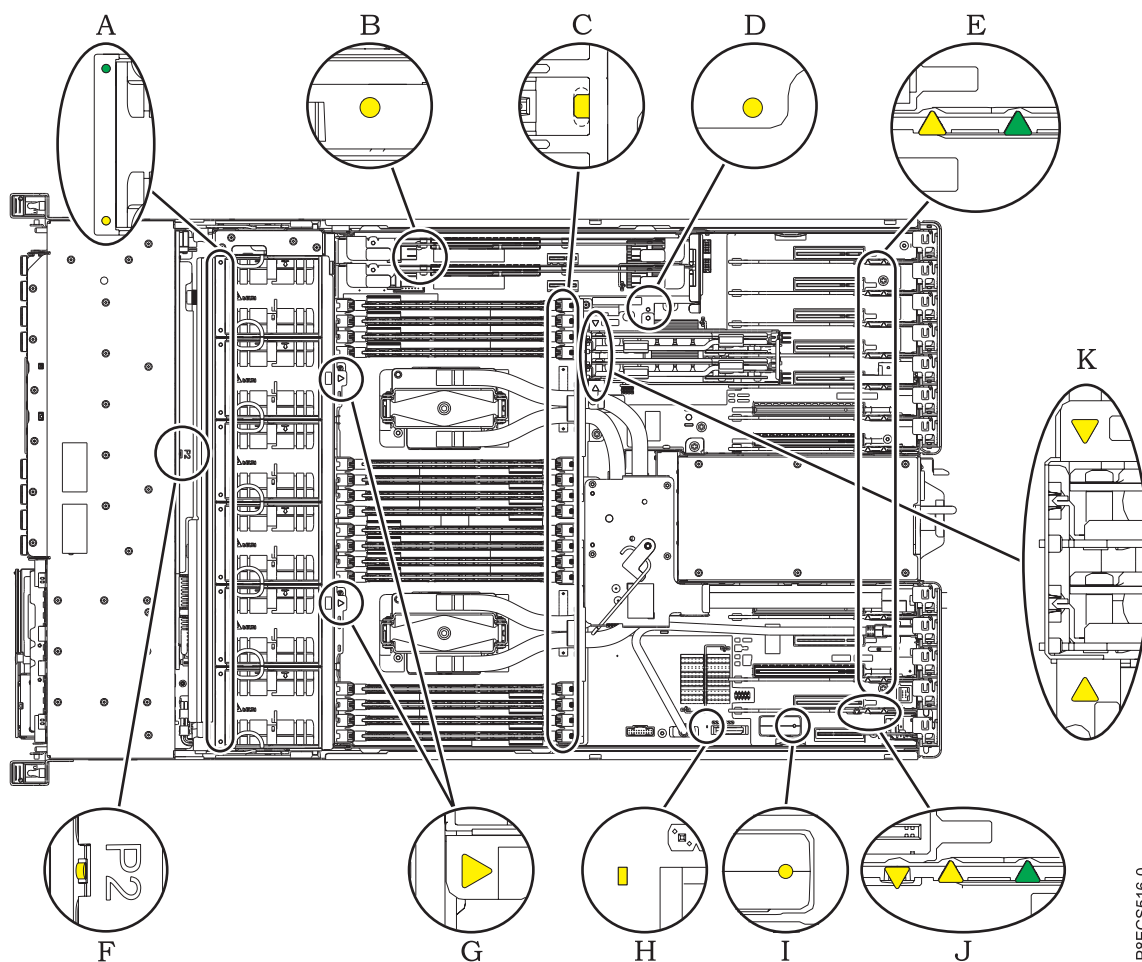
図 22. サービス・インジケター LED
