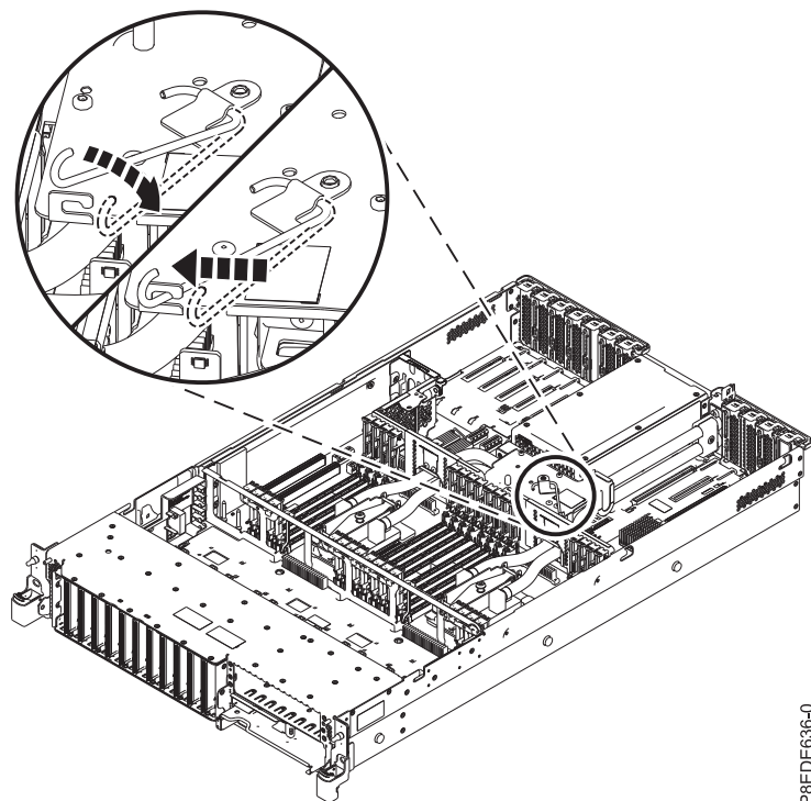
図 43. 保守フックを止め金の付いている位置に戻す
