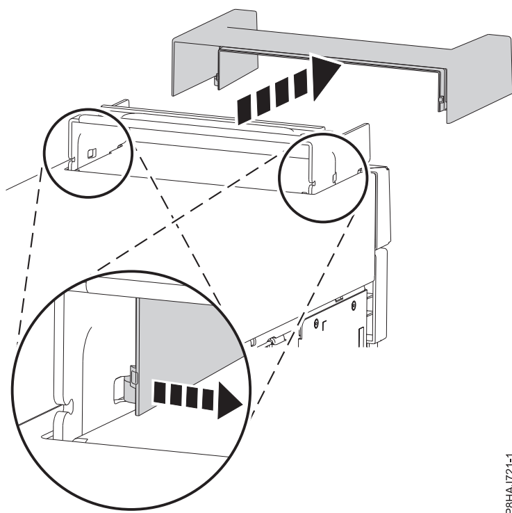
図 52. 8286-41A スタンドアロン・システムからのハンドル・カバーの取り外し
