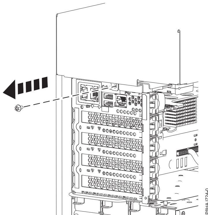
図 53. 8286-41A のサイド・カバーからのねじの取り外し
