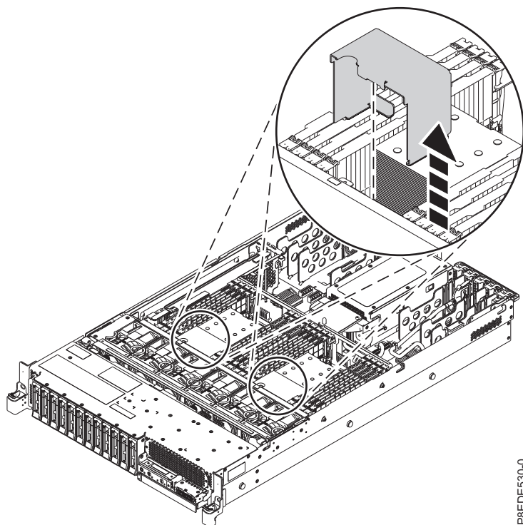
図 3. エア・パффルの取り外し
