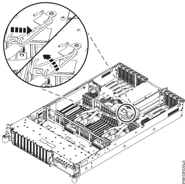
図 25. 保守フックの止め金を外す
