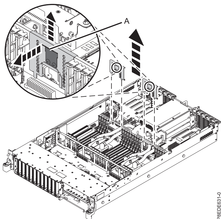
図 24. バッフルの取り外し
