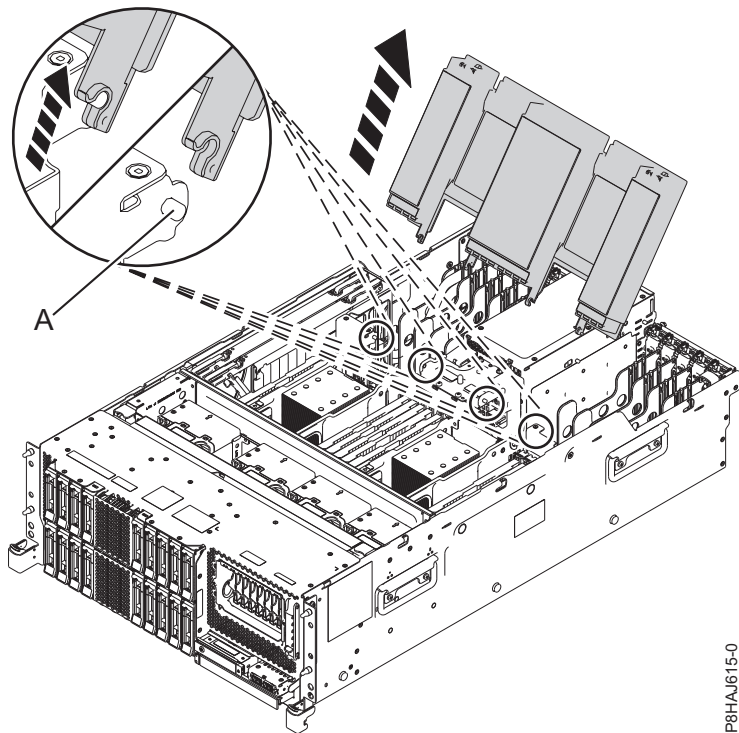
図 69. エア・バッフルの取り外し
