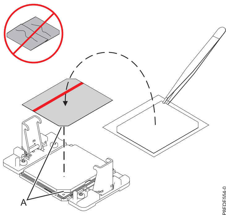
図 40. 熱伝導材料 (TIM) の取り替え
