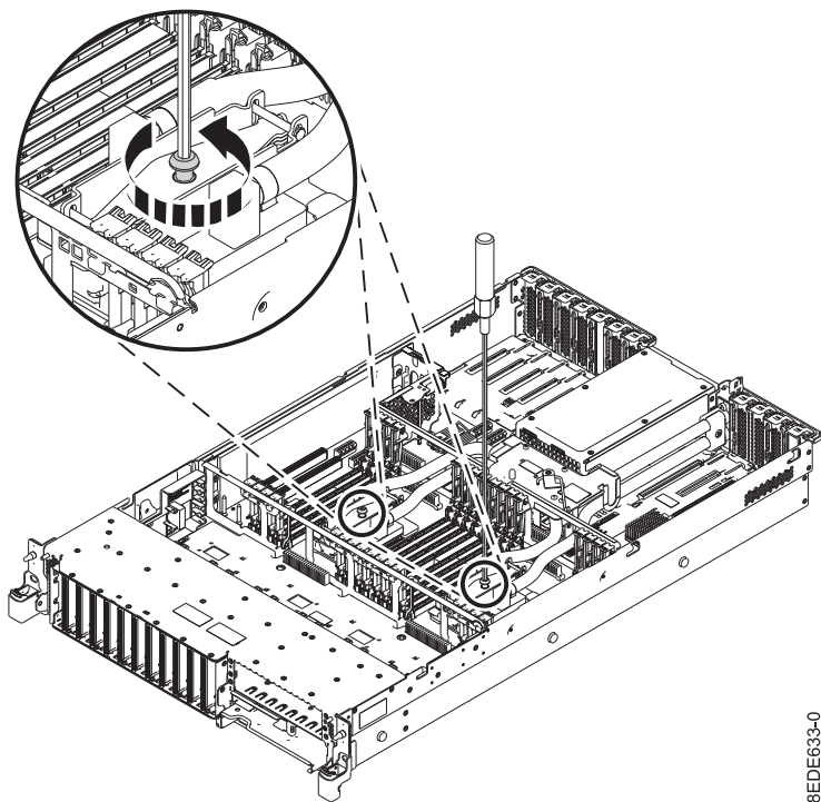
図 26. 冷却プレートの保持ねじを緩める
