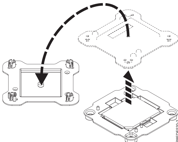
図 2. システム・プロセッサ・モジュールのパッケージを開く
