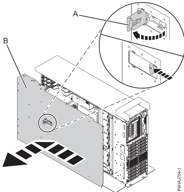
図 38. 保守アクセス・カバーの取り外し
