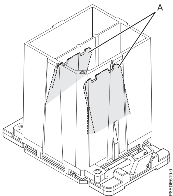
図 14. システム・プロセッサ・モジュール・ツールの取り外し
