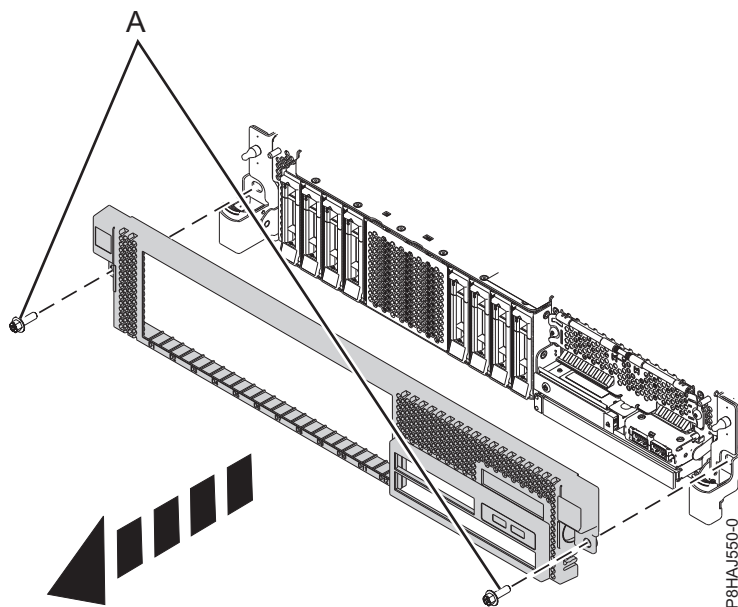
図 22. 前面カバーの取り外し
